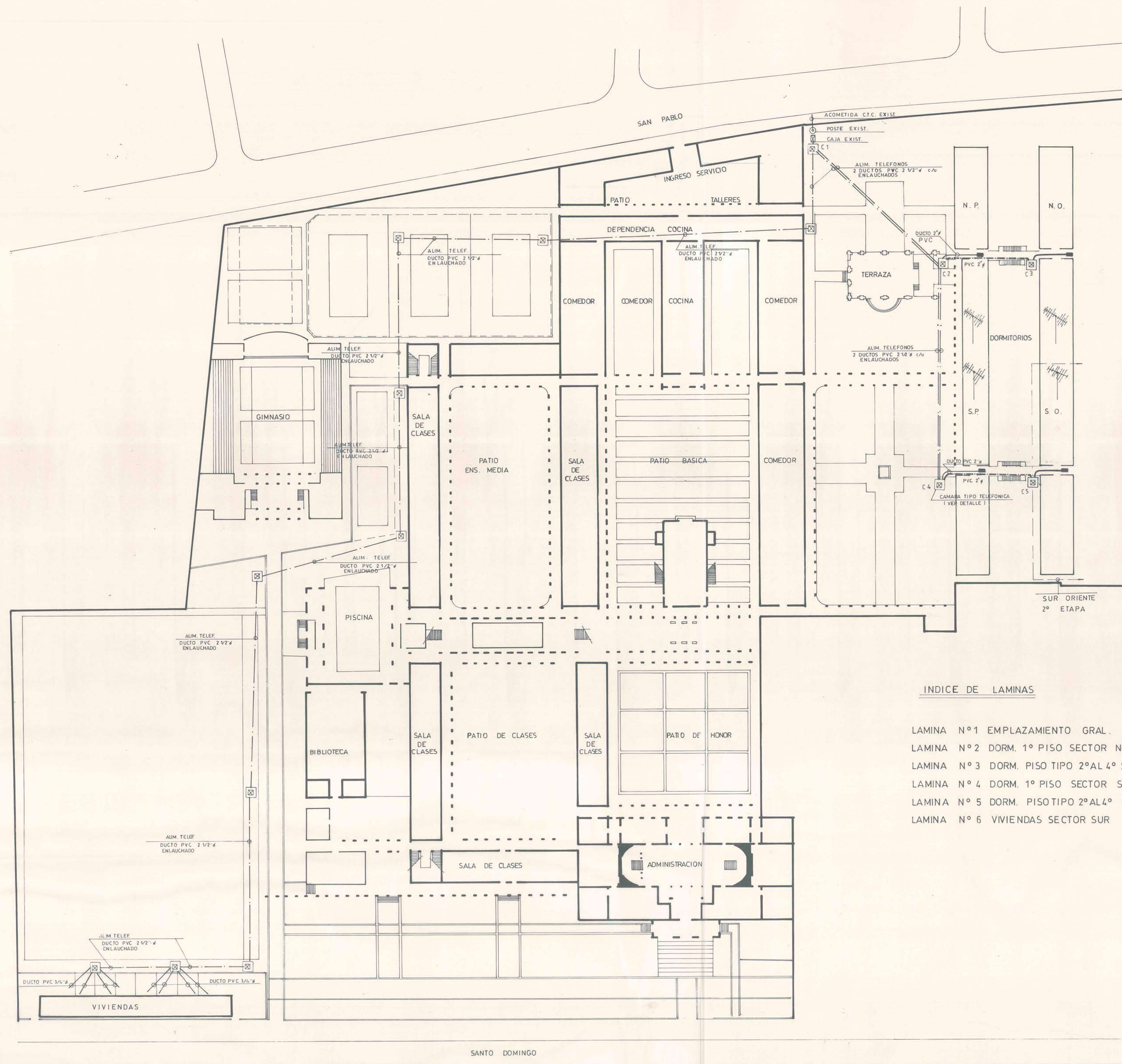
PLANTA EMPLAZAMIENTO GENERAL
