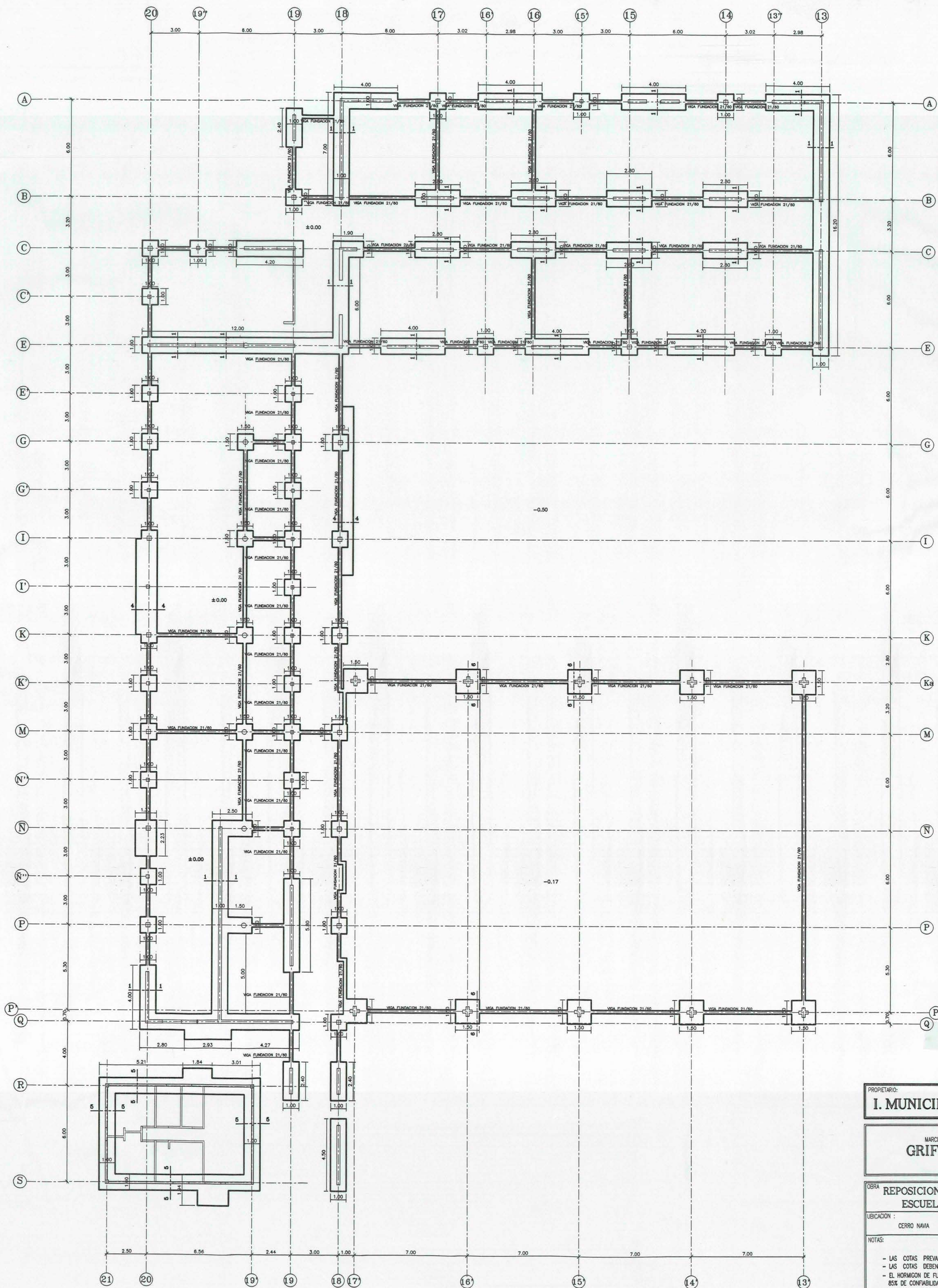
PLANTA FUNDACIONES ETAPA III
