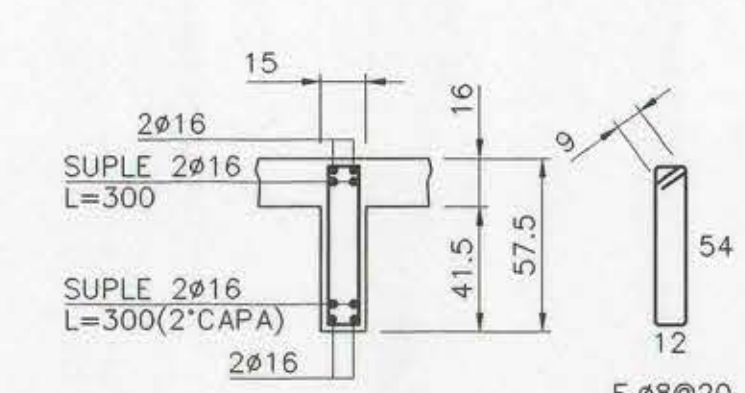
DETALLE V1-V2 15/57.5 ESCALA 1:25
