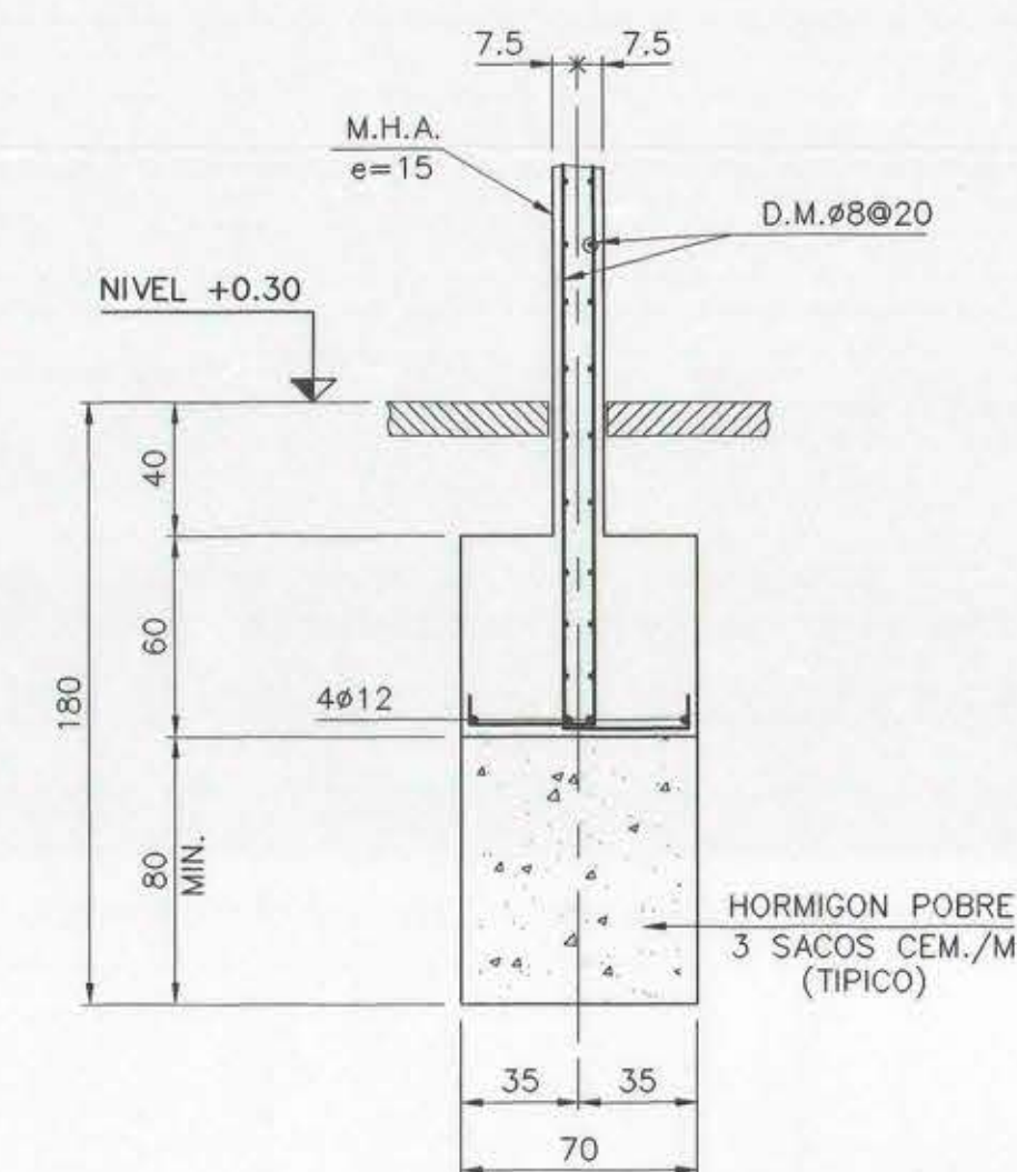
SECCION A ESCALA 1:25
