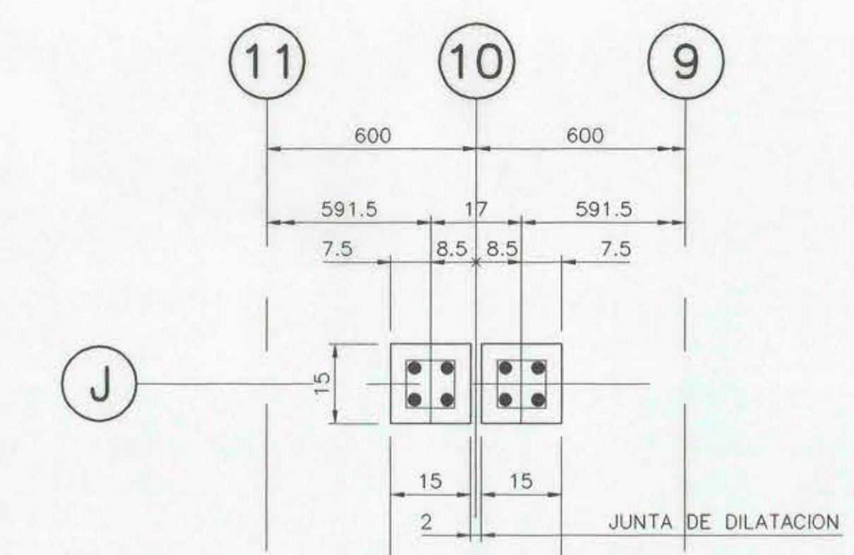
DETALLE PILARES EN JUNTA DE DILATACION ESCALA 1:25
