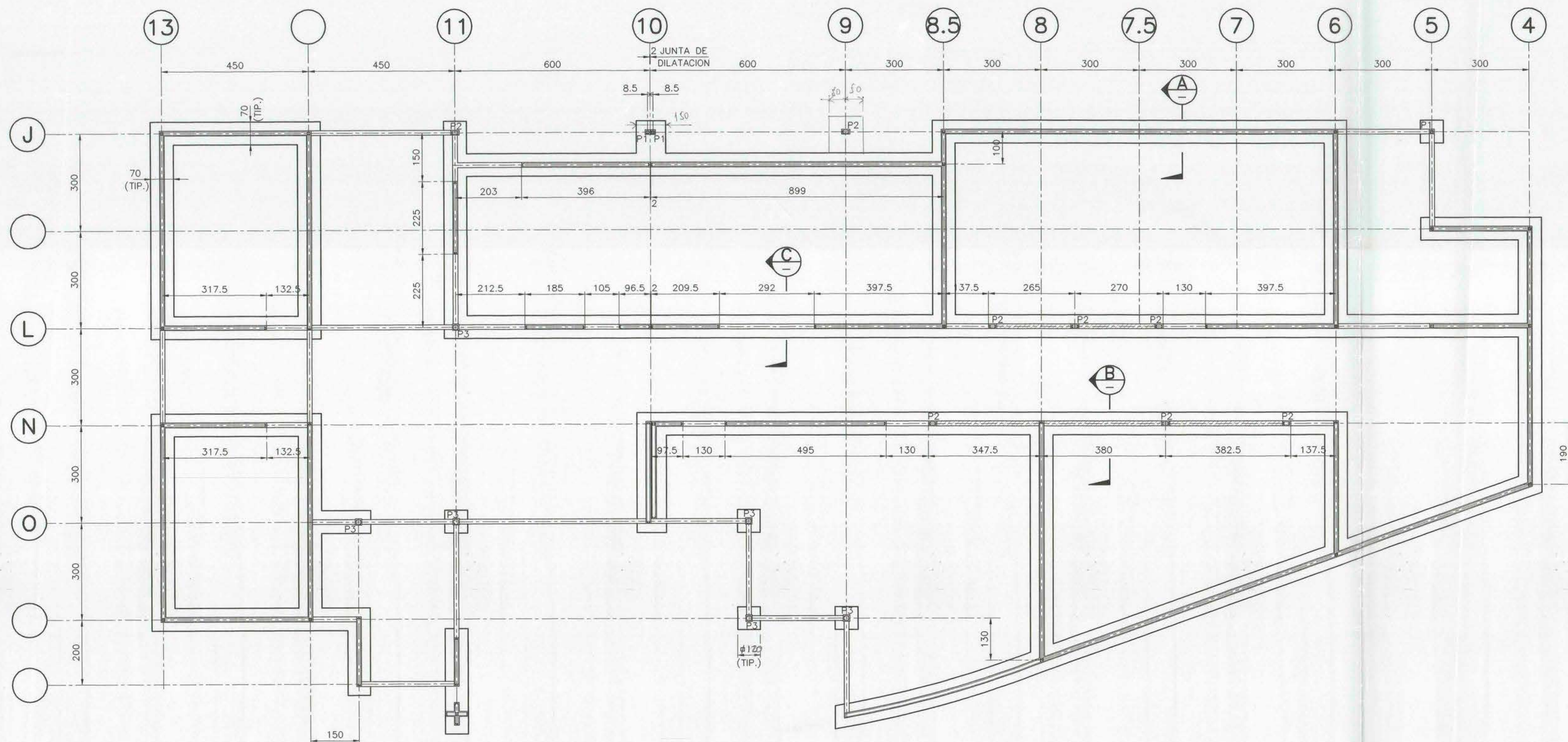
PLANTA DE FUNDACIONES ESCALA 1:75
