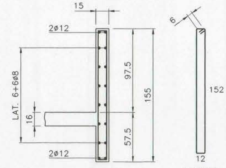
DETALLE V.S.I. 15/57.5+97.5 ESCALA 1:25
