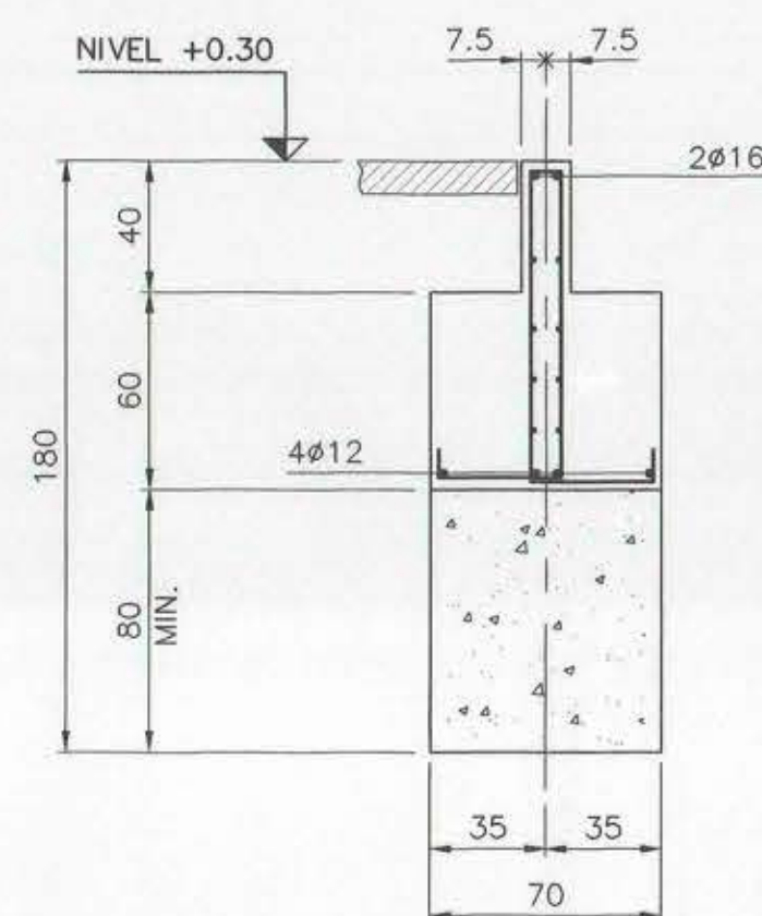
SECCION C ESCALA 1:25
