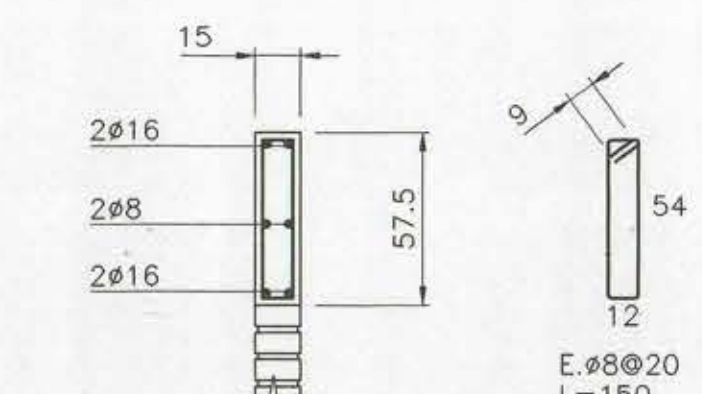
DETALLE CAD.15/57.5 ESCALA 1:25
