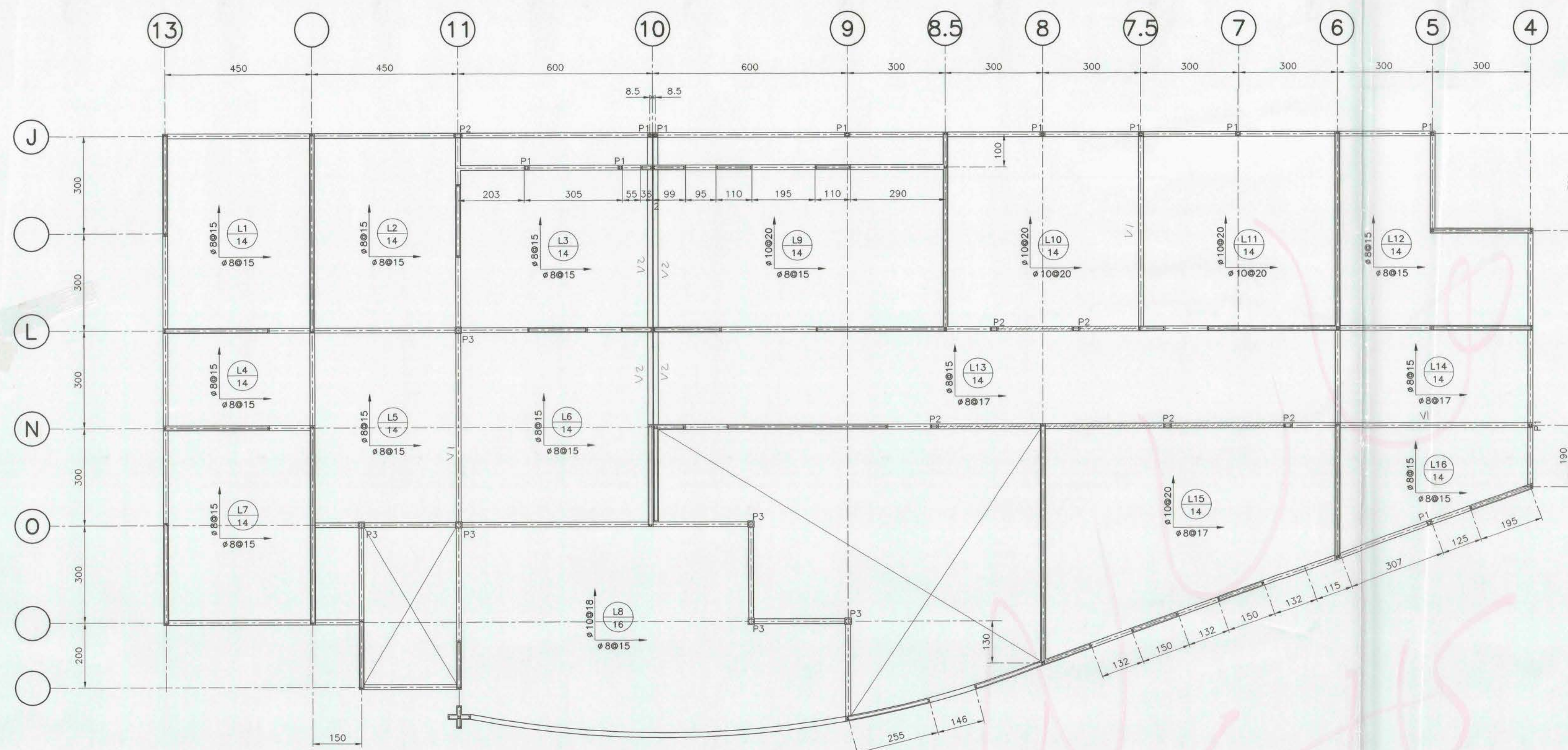
PLANTA DE CIELO 1° PISO ESCALA 1:75
