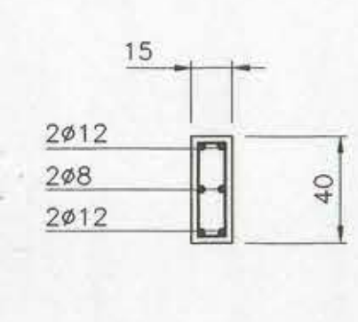
DETALLE V.F.15/40 ESCALA 1:25
