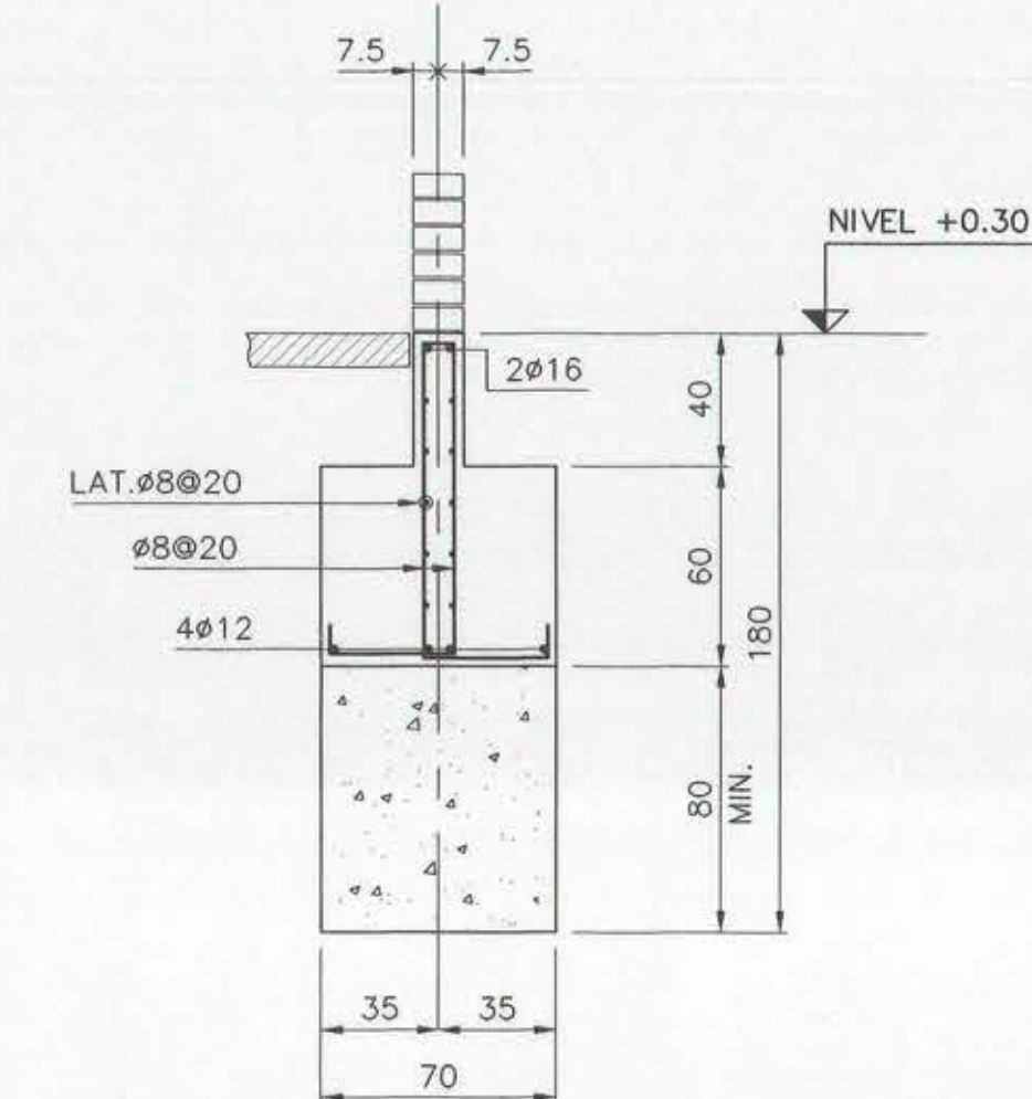
SECCION B ESCALA 1:25
