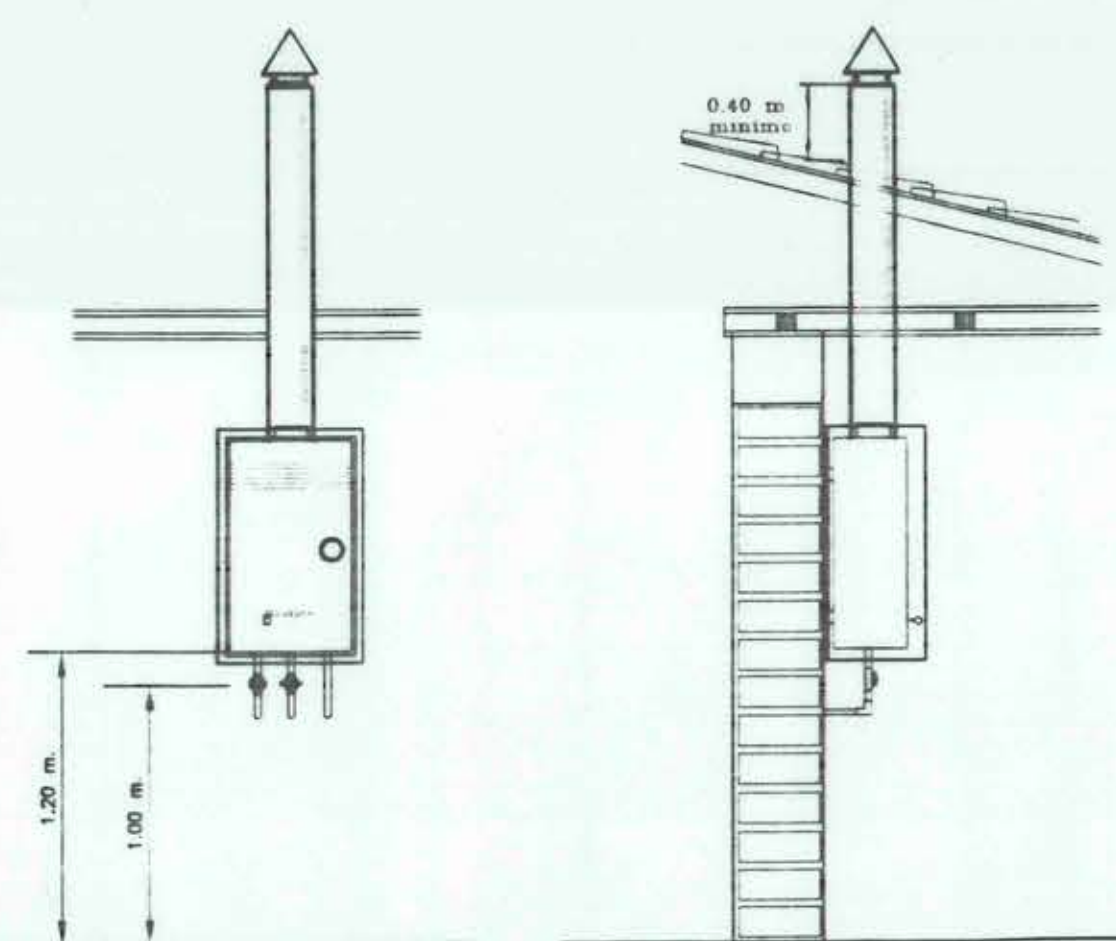
ELEVACION PERFIL DETALLE : DUCTO VENTILACION CALEFON AL EXTERIOR EN CASETA METALICA
