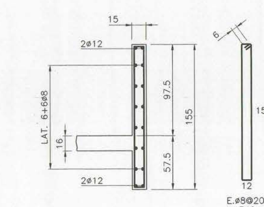
DETALLE V.S.I. 15/57.5+97.5 ESCALA 1:25
