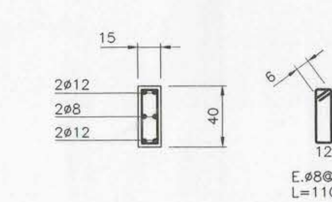
DETALLE V.F.15/40 ESCALA 1:25
