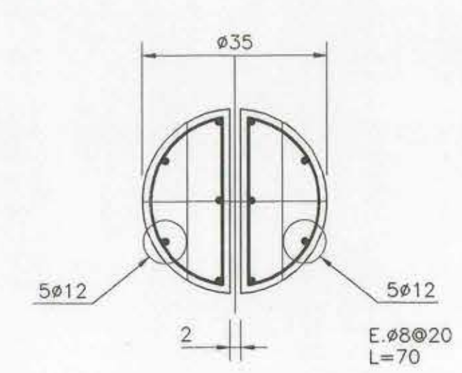
DETALLE PILAR P4 ESCALA 1:10
