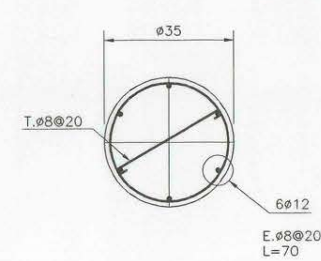
DETALLE PILAR P3 ESCALA 1:10
