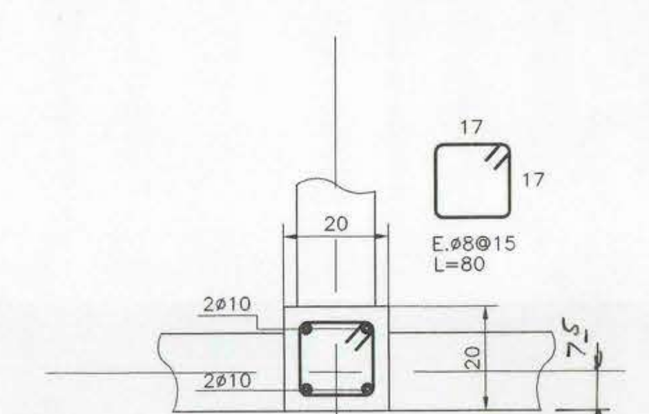
DETALLE 1 ESCALA 1:10
