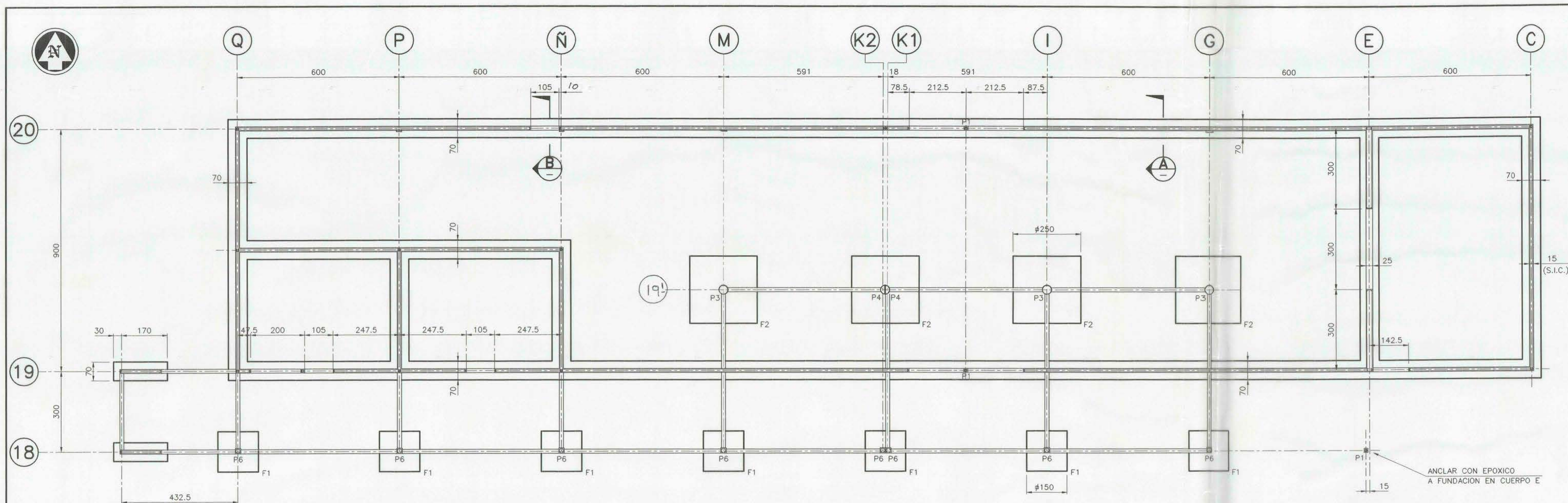
PLANTA DE FUNDACIONES ESCALA 1:75
