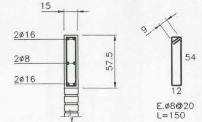
DETALLE CAD.15/57.5 ESCALA 1:25
