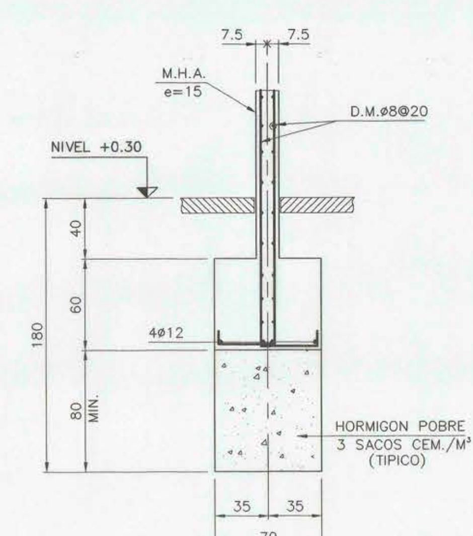
SECCION A ESCALA 1:25
