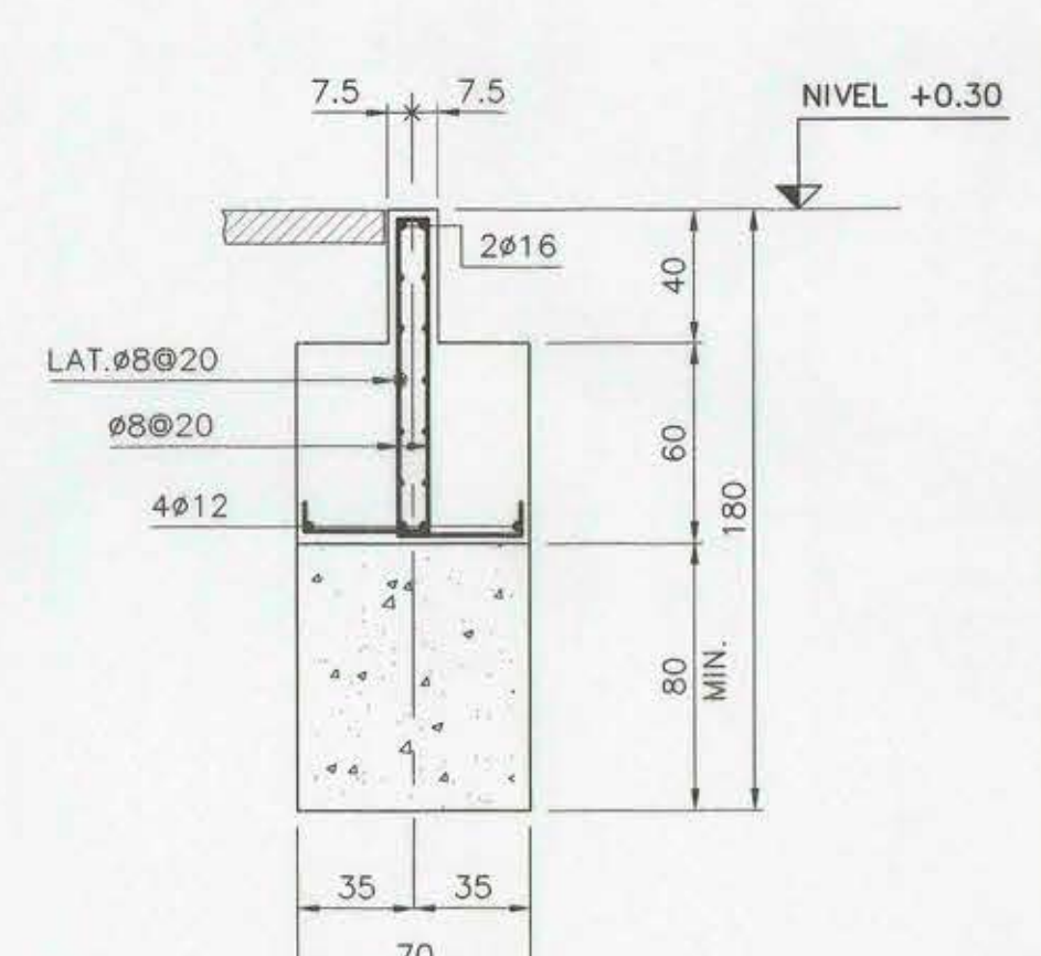
SECCION B ESCALA 1:25
