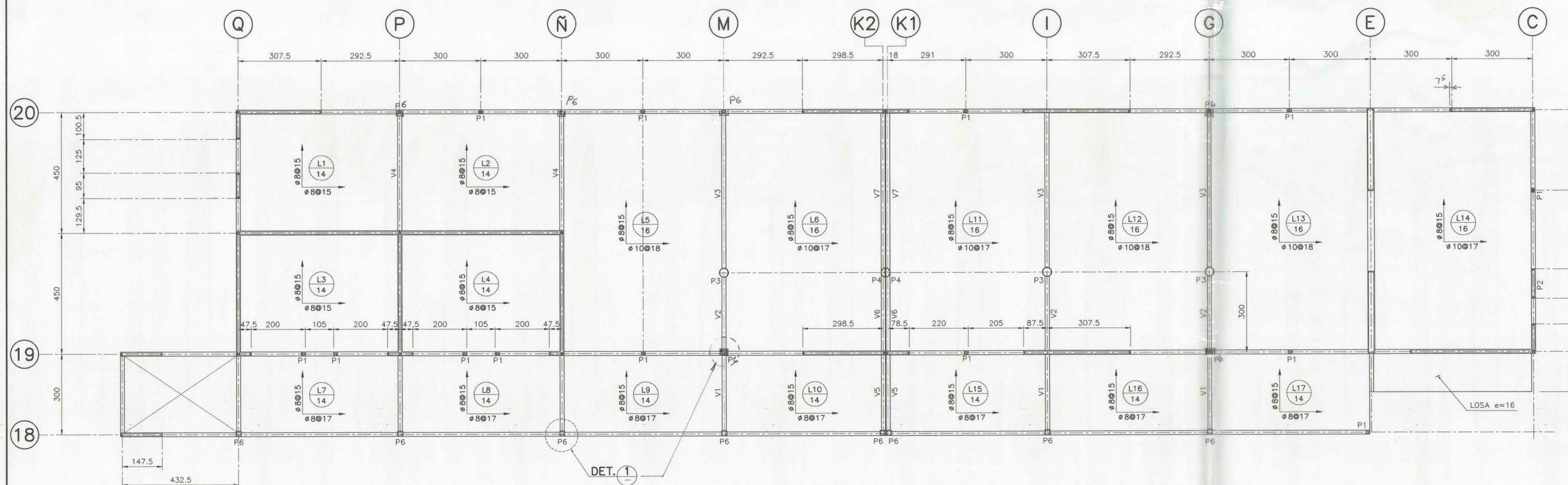
PLANTA CIELO 1° PISO ESCALA 1:75
