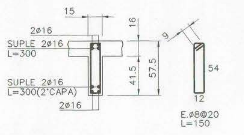
DETALLE V1-V2-V3 15/57.5 ESCALA 1:25
