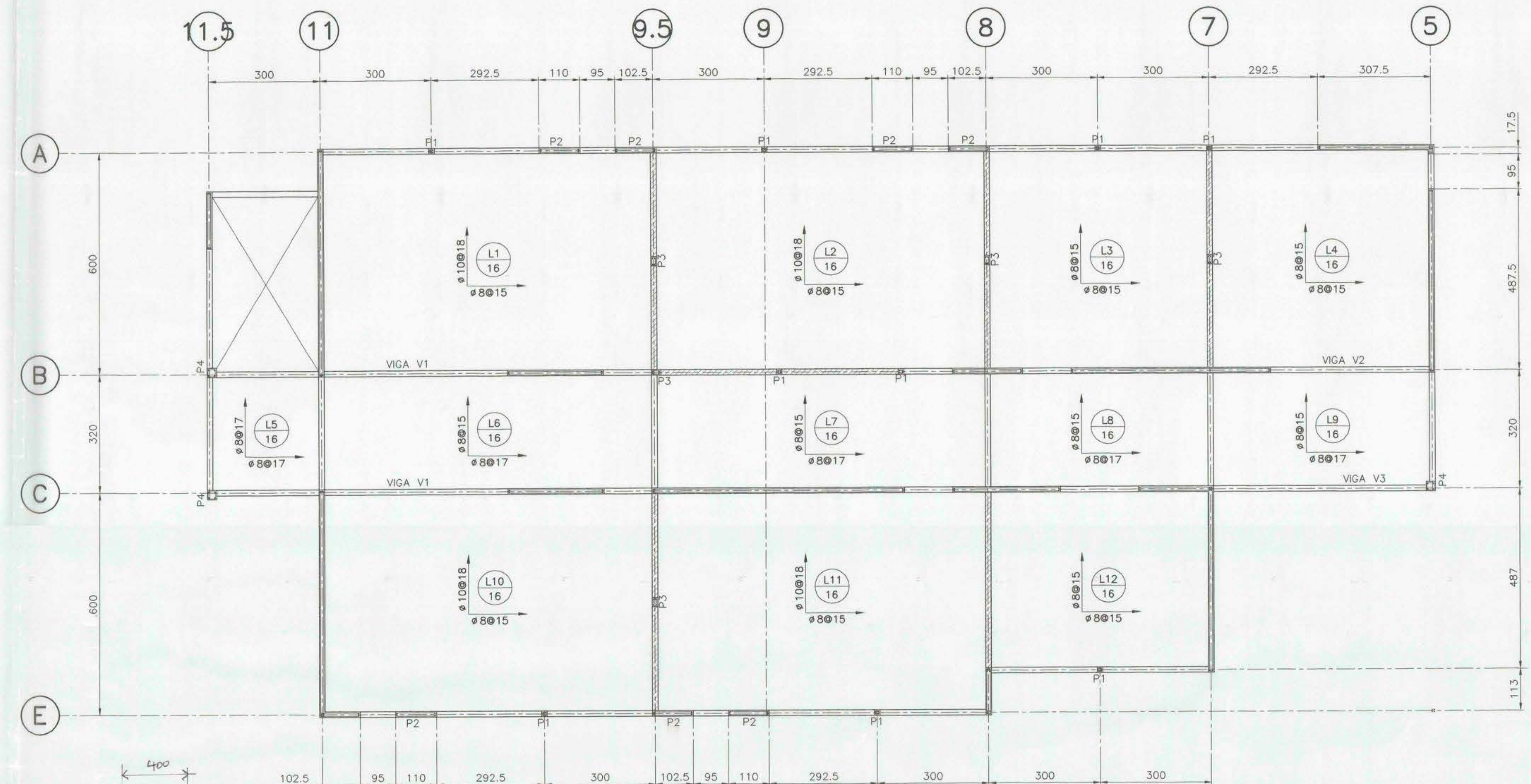
PLANTA CIELO 1° PISO ESCALA 1:75
