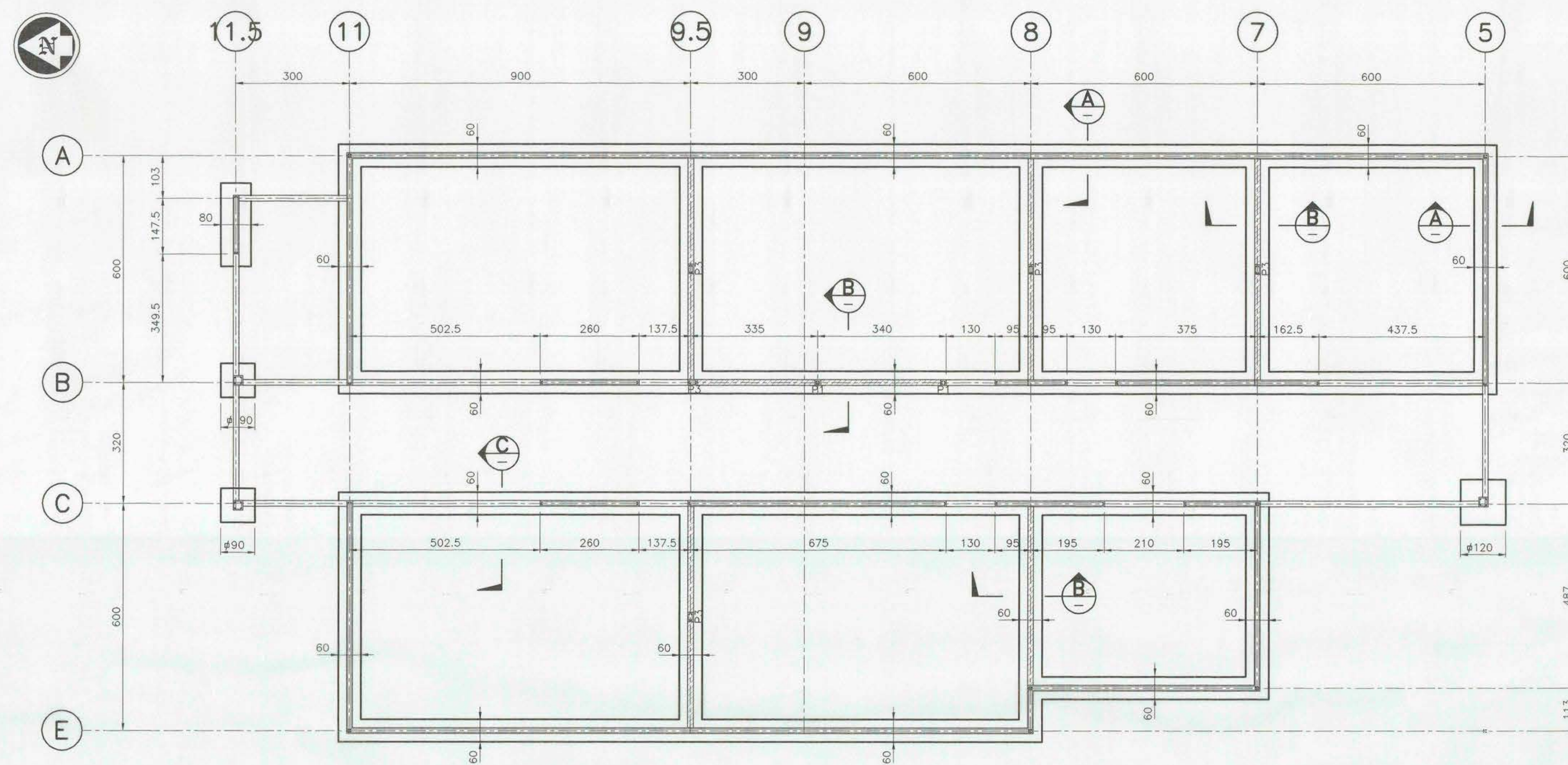
PLANTA DE FUNDACIONES ESCALA 1:75
