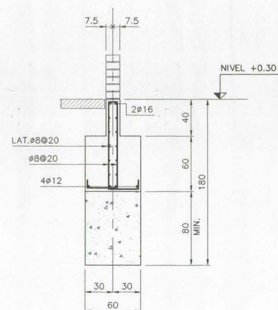
SECCION B ESCALA 1:25
