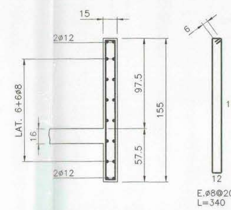
DETALLE V.S.I. 15/57.5+97.5 ESCALA 1:25
