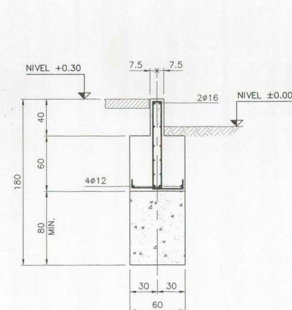
SECCION C ESCALA 1:25
