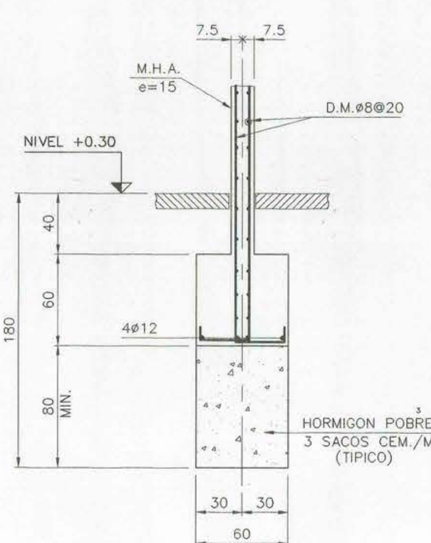
SECCION A ESCALA 1:25
