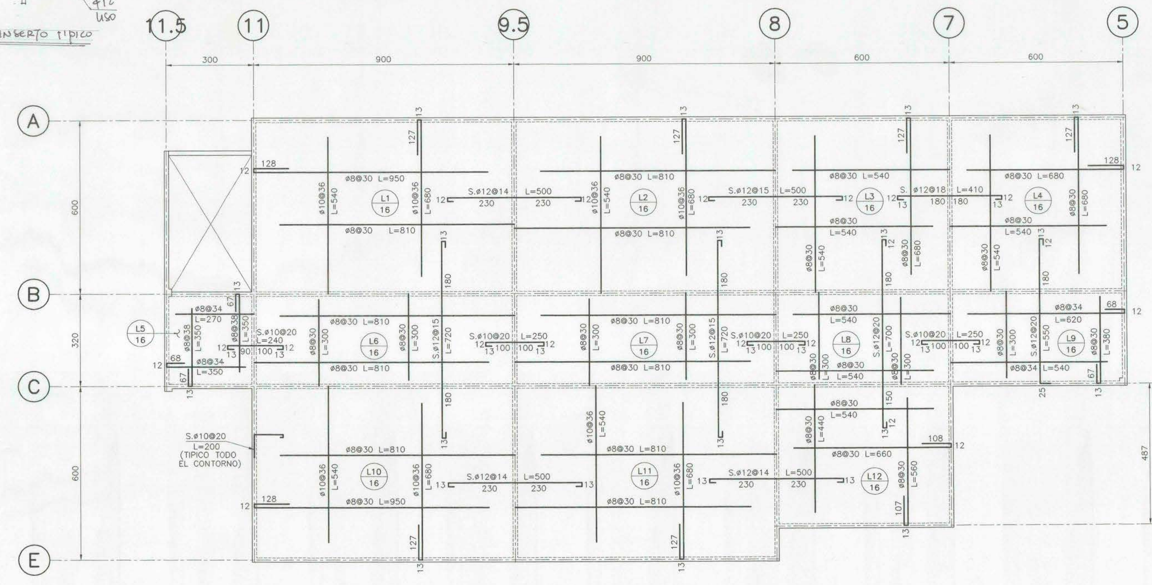
PLANTA ENFIERRADURAS DE LOSAS CIELO 1° PISO ESCALA 1:75
