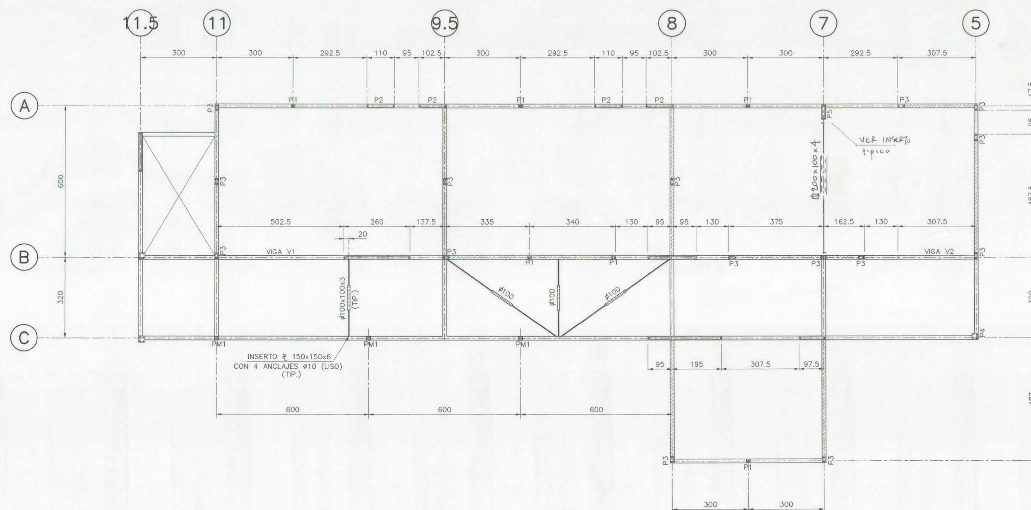
PLANTA CIELO 2° PISO ESCALA 1:75
