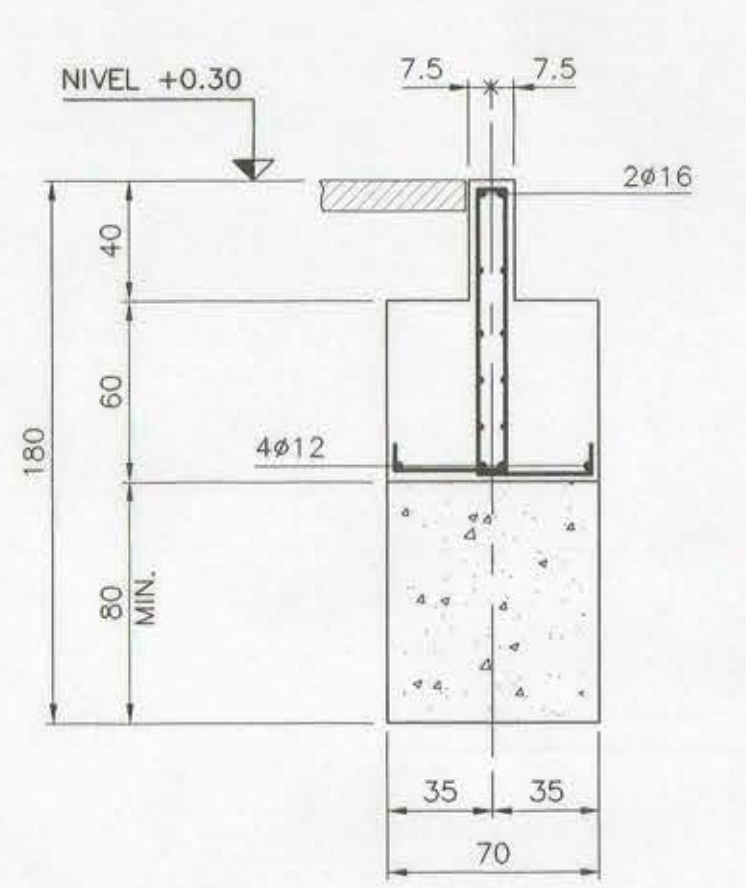
SECCION C ESCALA 1:25
