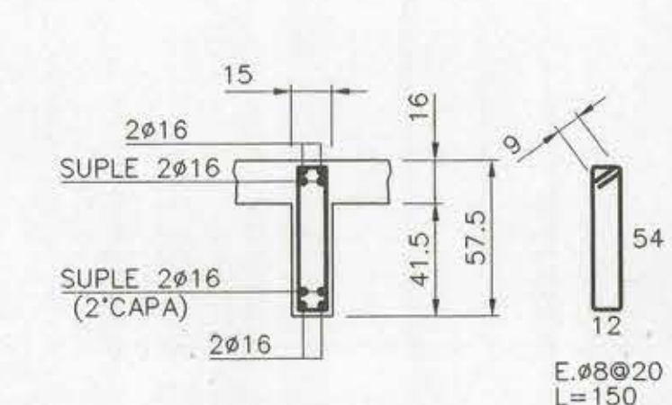
DETALLE V1-V2 15/57.5 ESCALA 1:25
