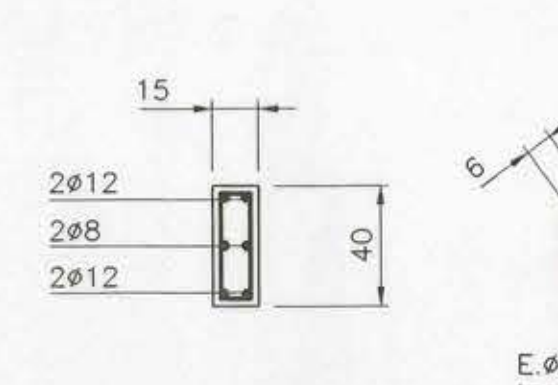
DETALLE V.F.15/40 ESCALA 1:25
