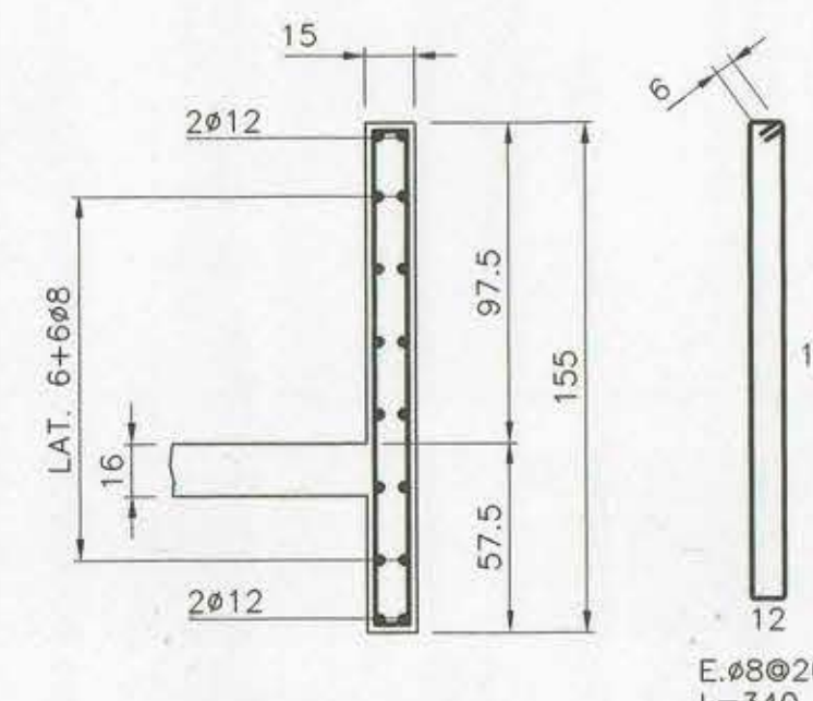
DETALLE V.S.I. 15/57.5+97.5 ESCALA 1:25
