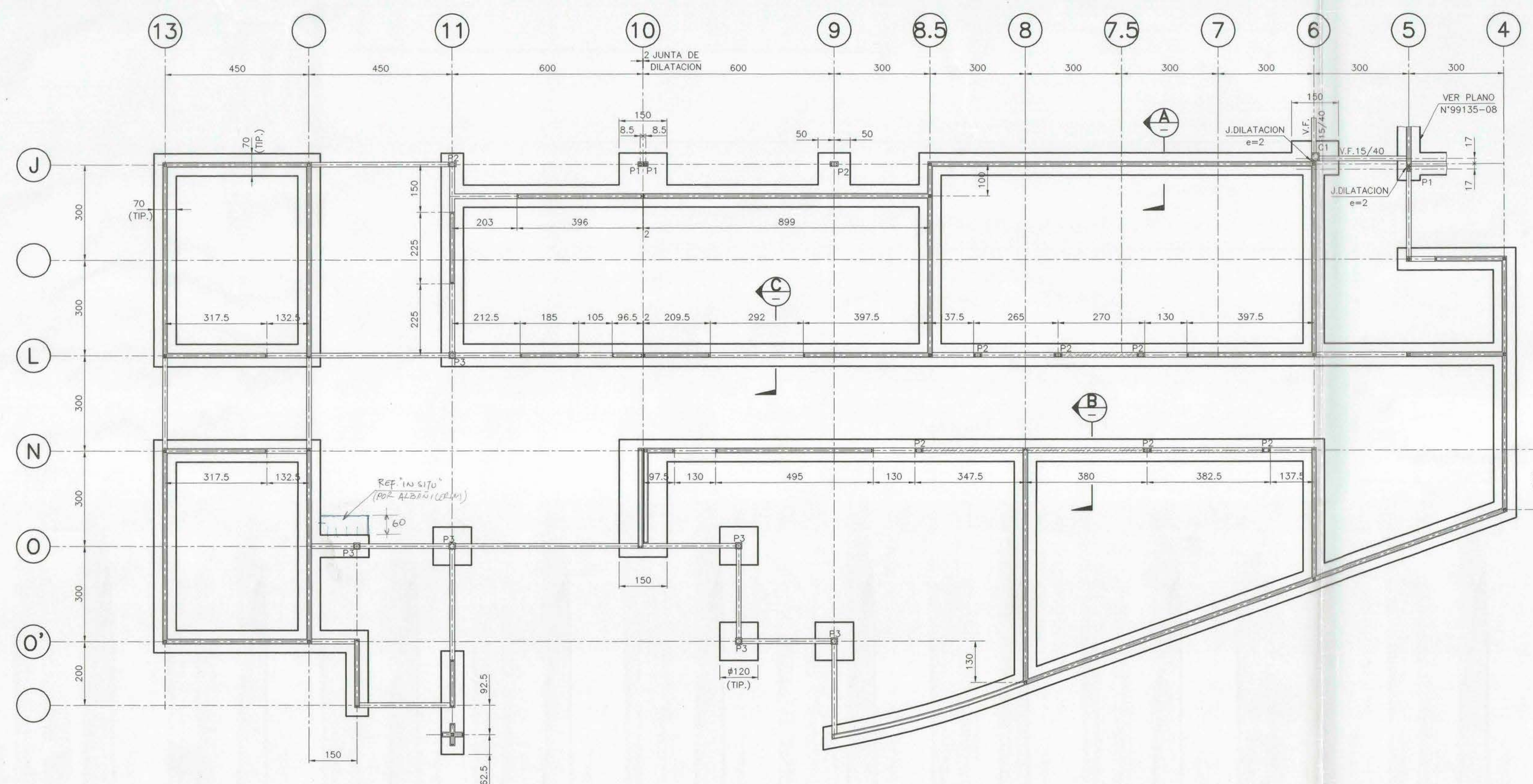
PLANTA DE FUNDACIONES ESCALA 1:75
