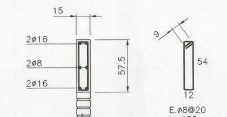
DETALLE CAD.15/57.5 ESCALA 1:25
