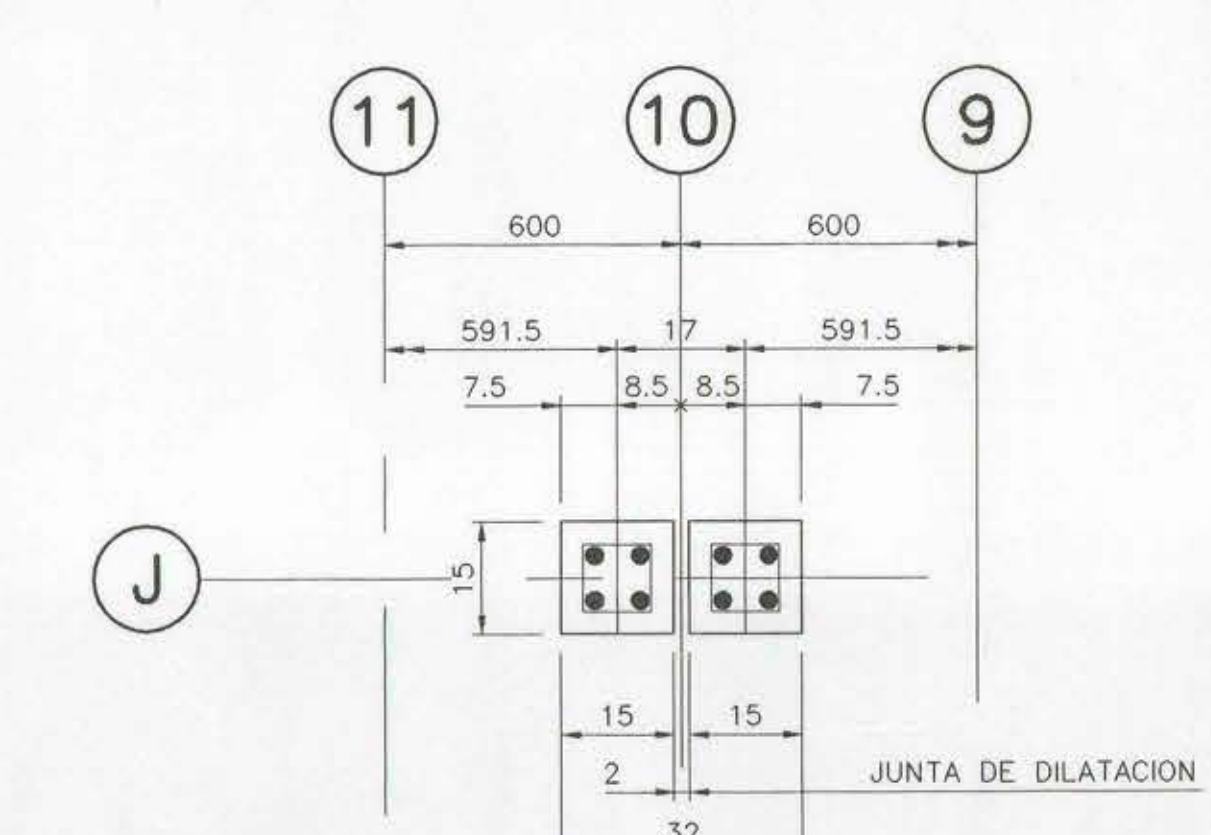
DETALLE PILARES EN JUNTA DE DILATACION ESCALA 1:10
