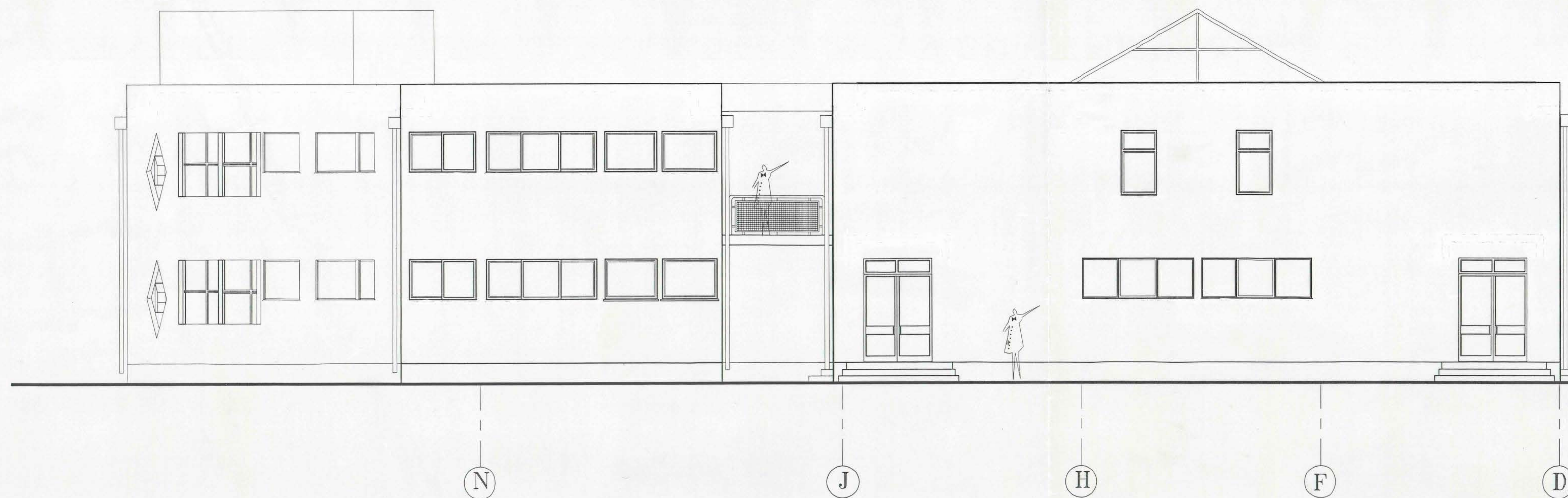
ELEVACION SUR ESC 1 : 50
