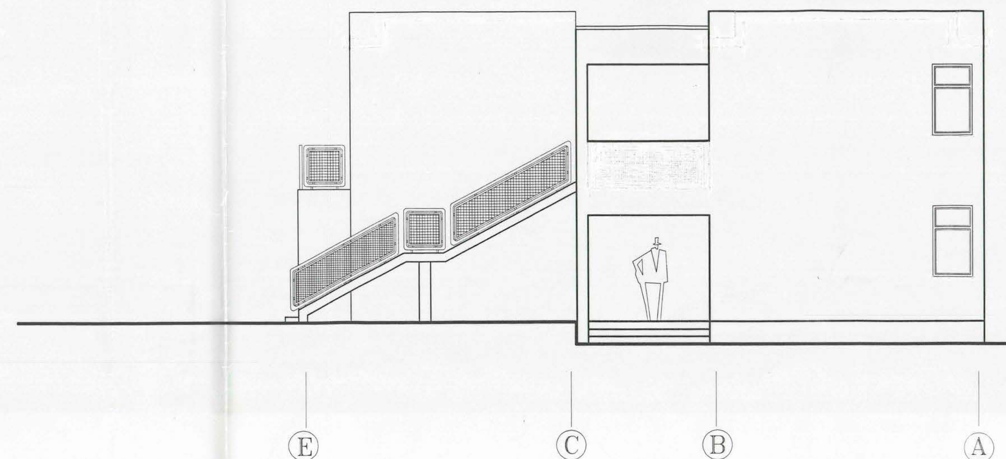
ELEVACION SUR ESC 1 : 50
