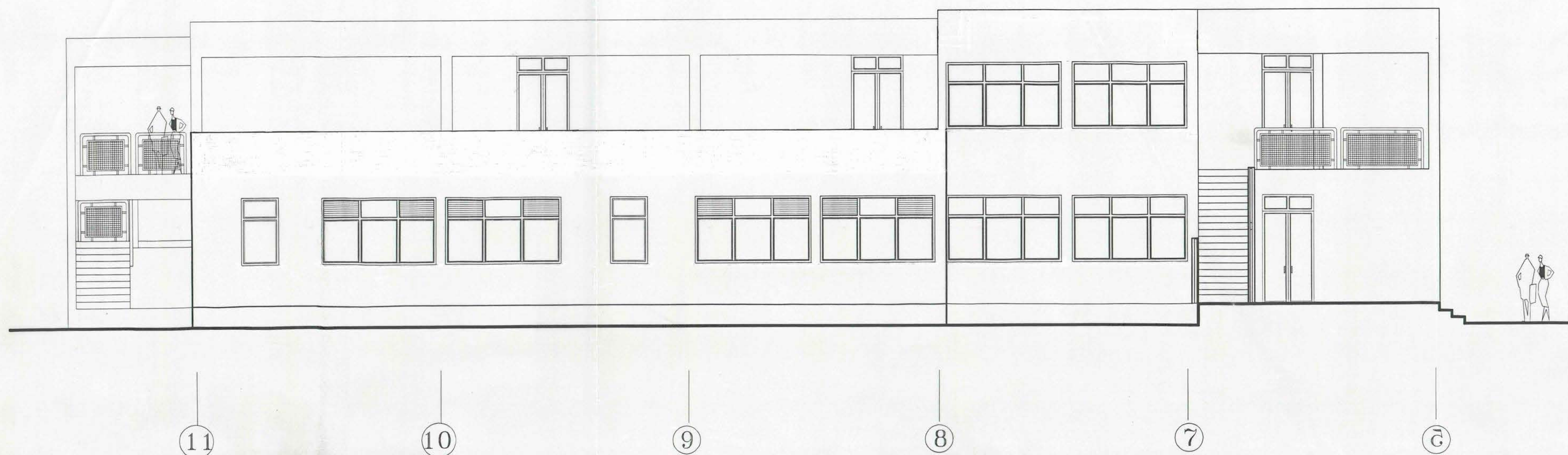
ELEVACION PONIENTE ESC 1 : 50
