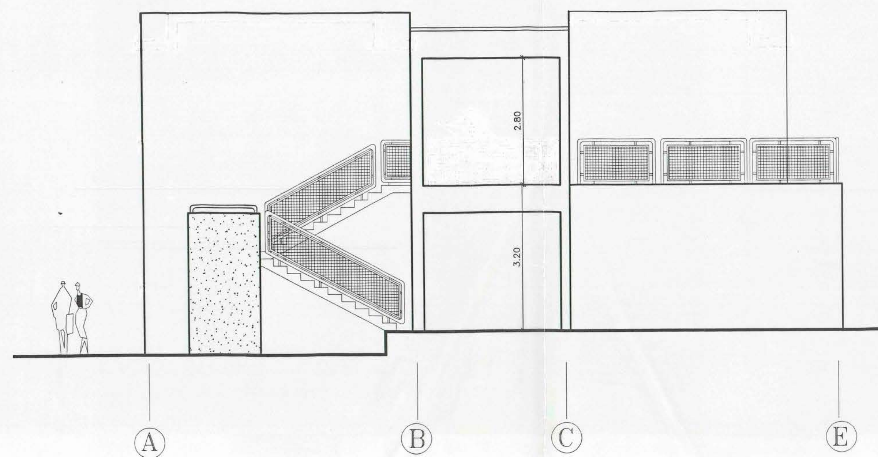
ELEVACION NORTE ESC 1 : 50
