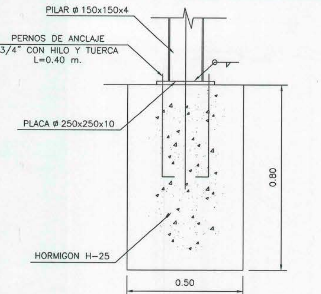
DETALLE 2 ESC. 1:10
