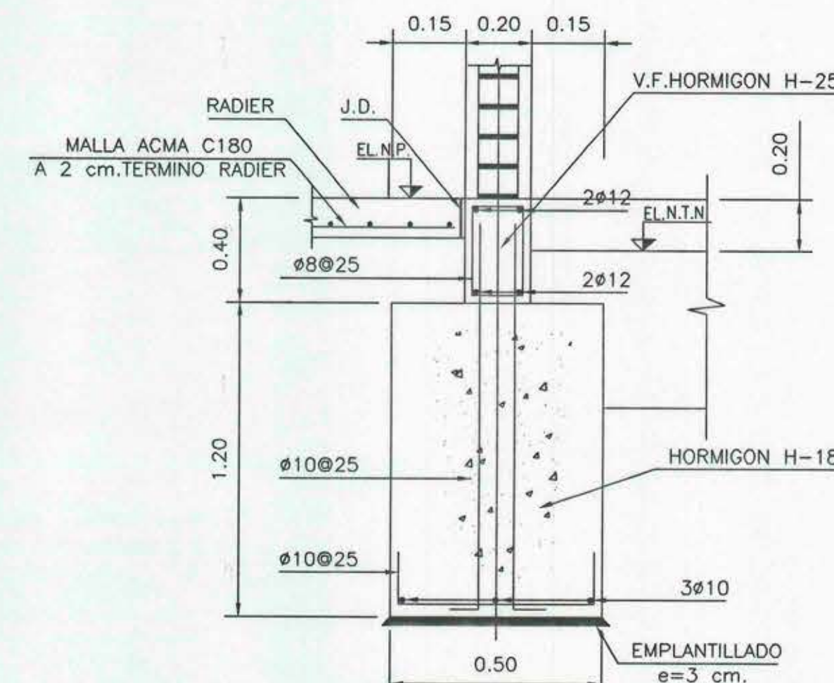
SECCION A-A ESC. 1:20
