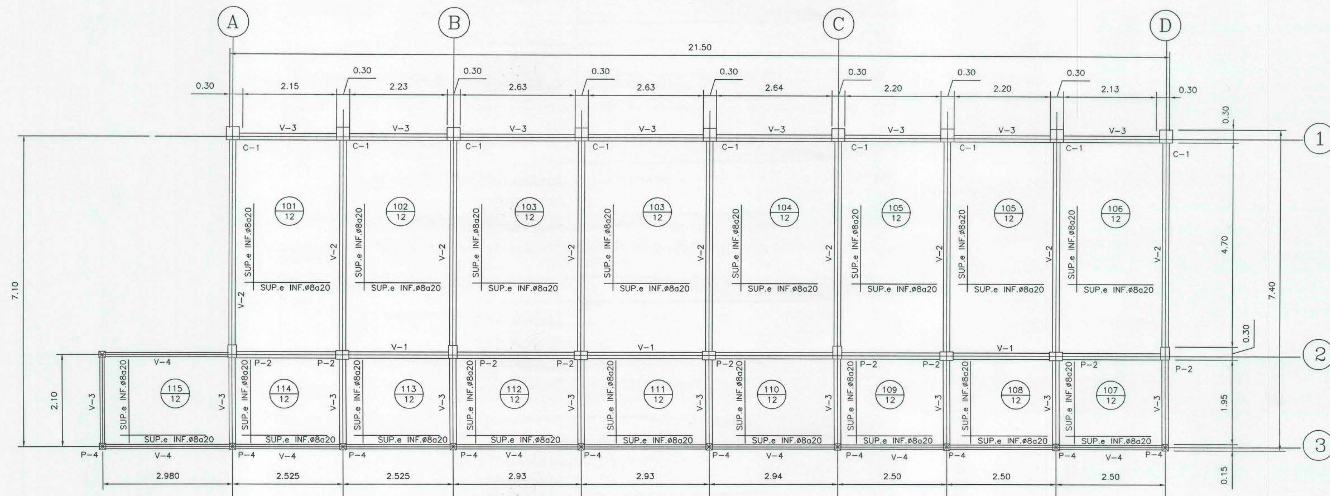
PLANTA VIGAS LOSAS NIVEL +3.30 Y PILARES
