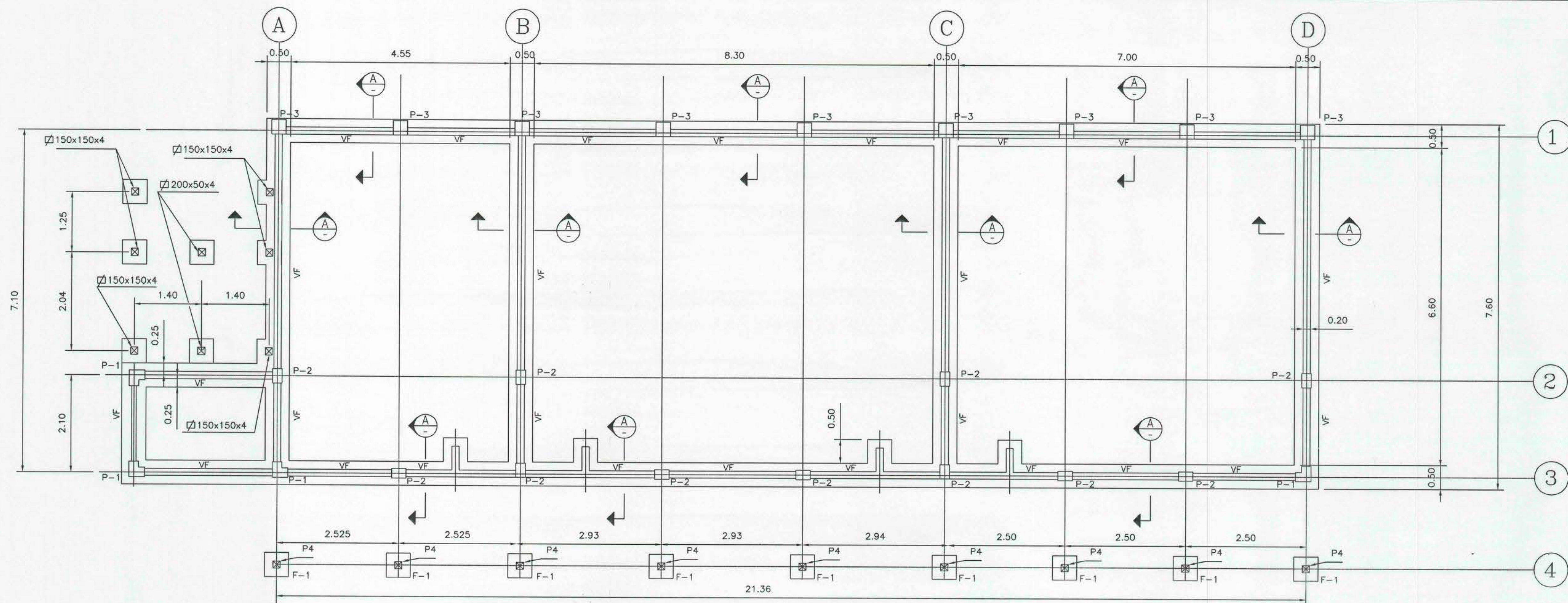
PLANTA FUNDACIONES Y PILARES NIVEL 0.00 ESCALA 1:50
