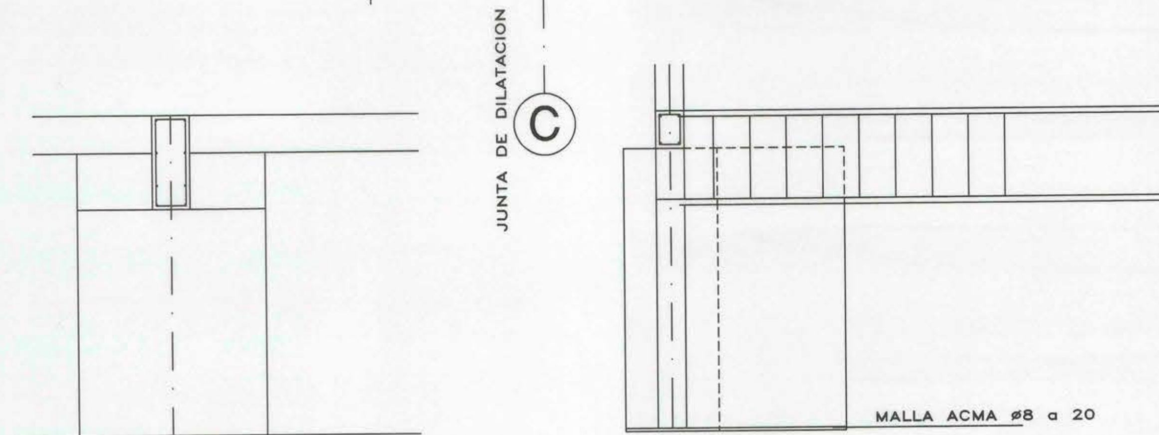
CORTE TIP VIGA DE FUNDACION ESC. 1: 20
