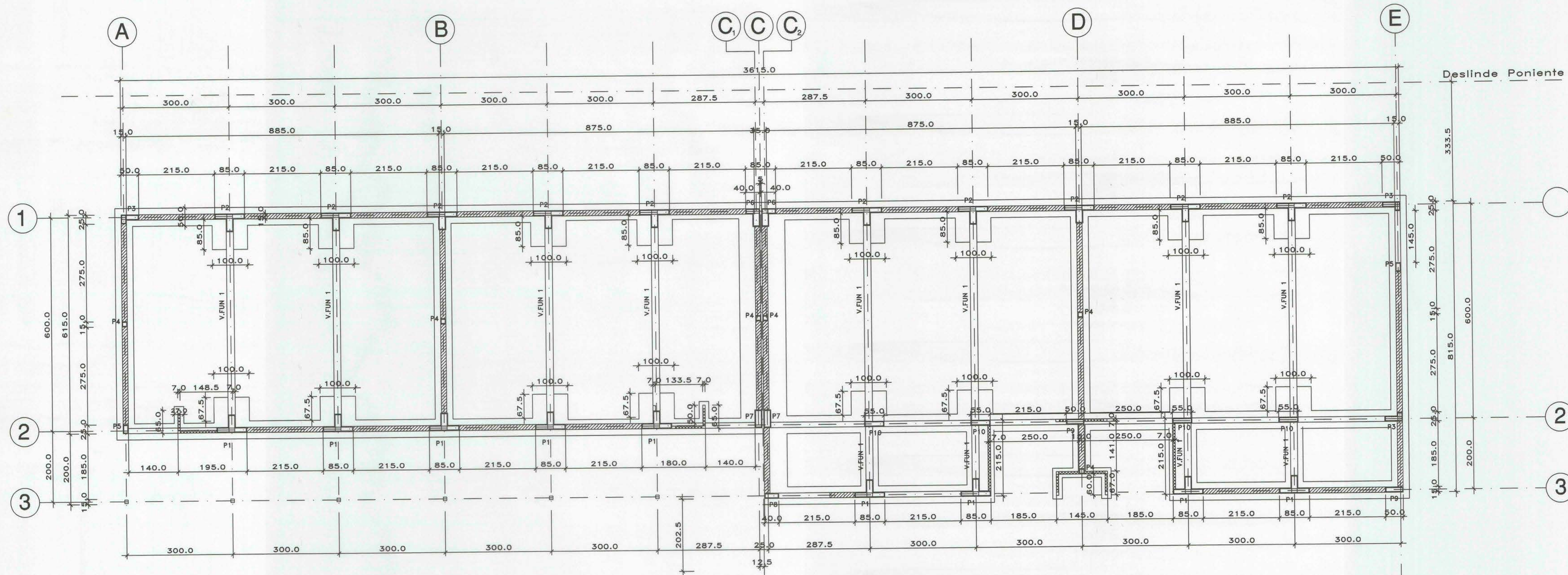
PLANTA DE FUNDACIONES ESC. 1: 50
