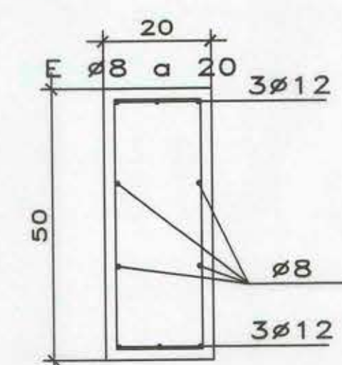
VIGA FUNDACION
