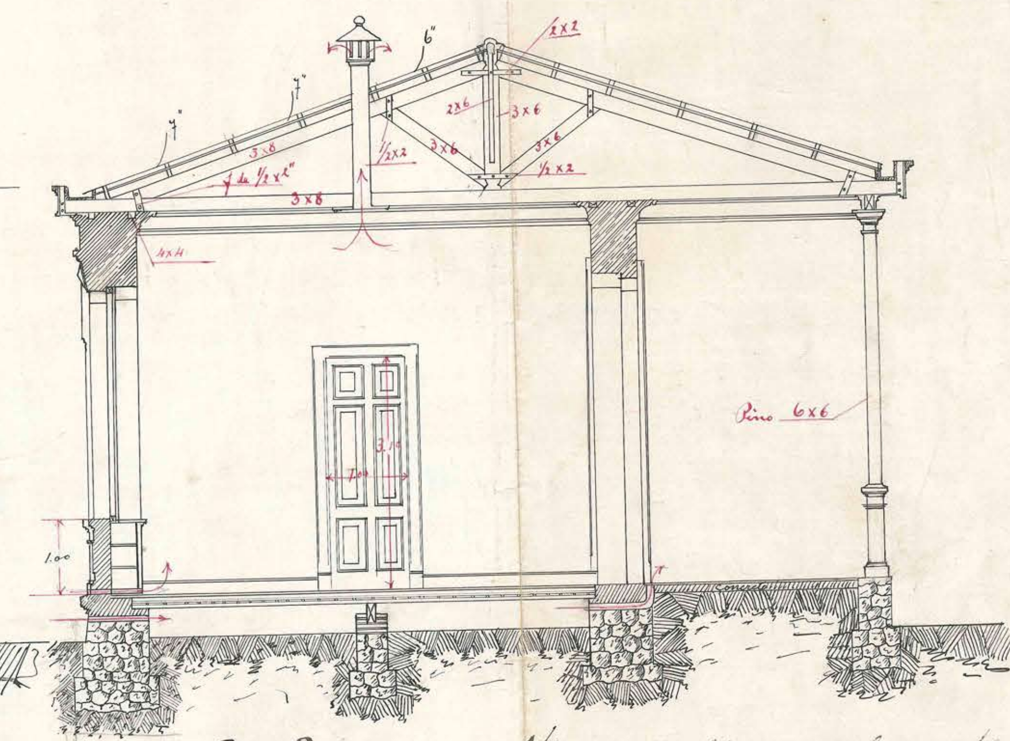
Seccion transversal
