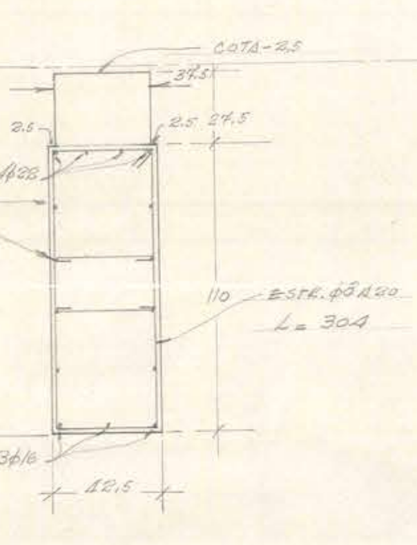
V.F. 40/110 SECC. P-P.
