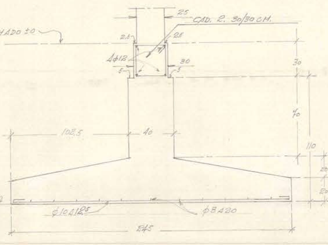
SECCION G-G ALBAÑILERIA EXTERIORES.
