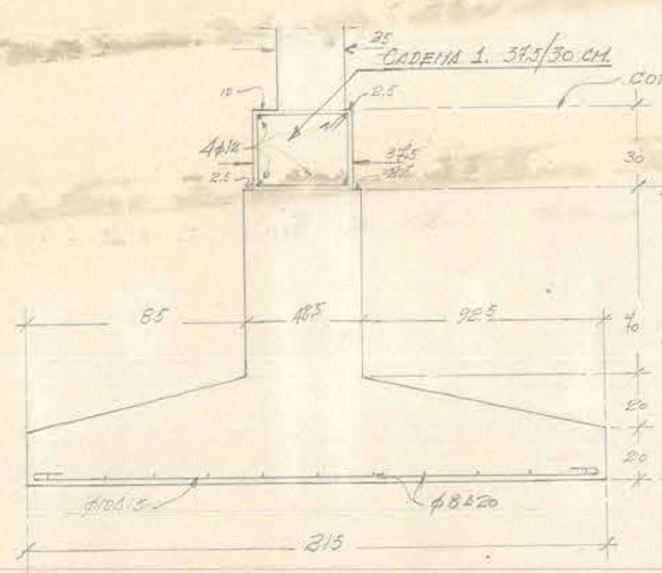
SECCION A-A MURO ALB. SUR 25CM.
