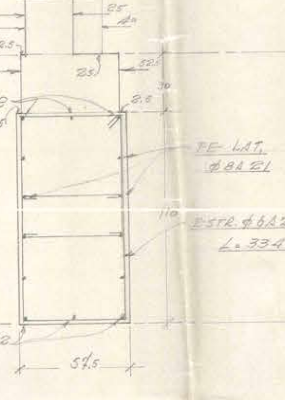
V.F. 40/110 SECC. N-N.
