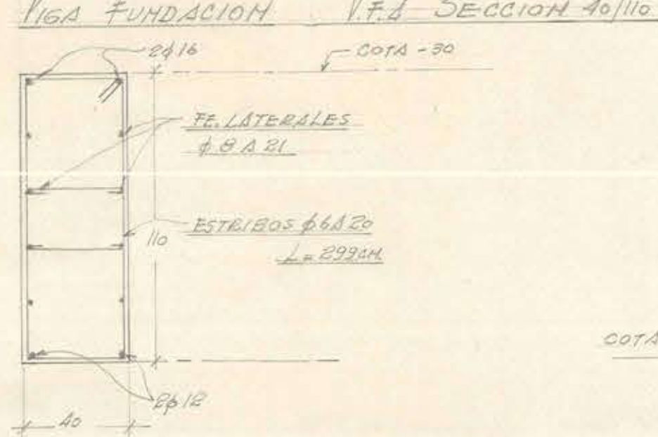
SECCION F-F VIGA FUNDACION V.F. SECCION 40/110.
