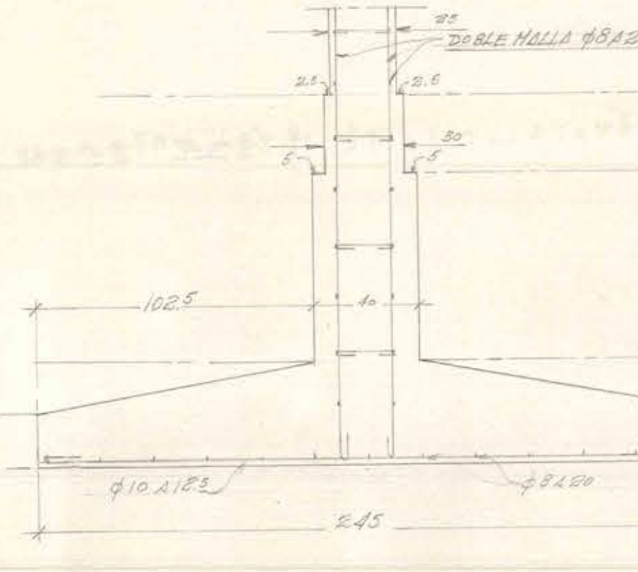
V.F. 40/110 SECC. L-L.
