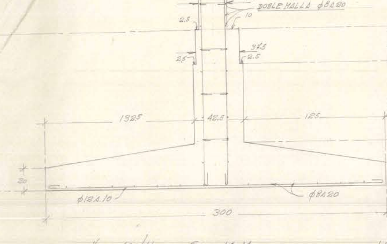
V.F. 40/110 SECC. P-P.
