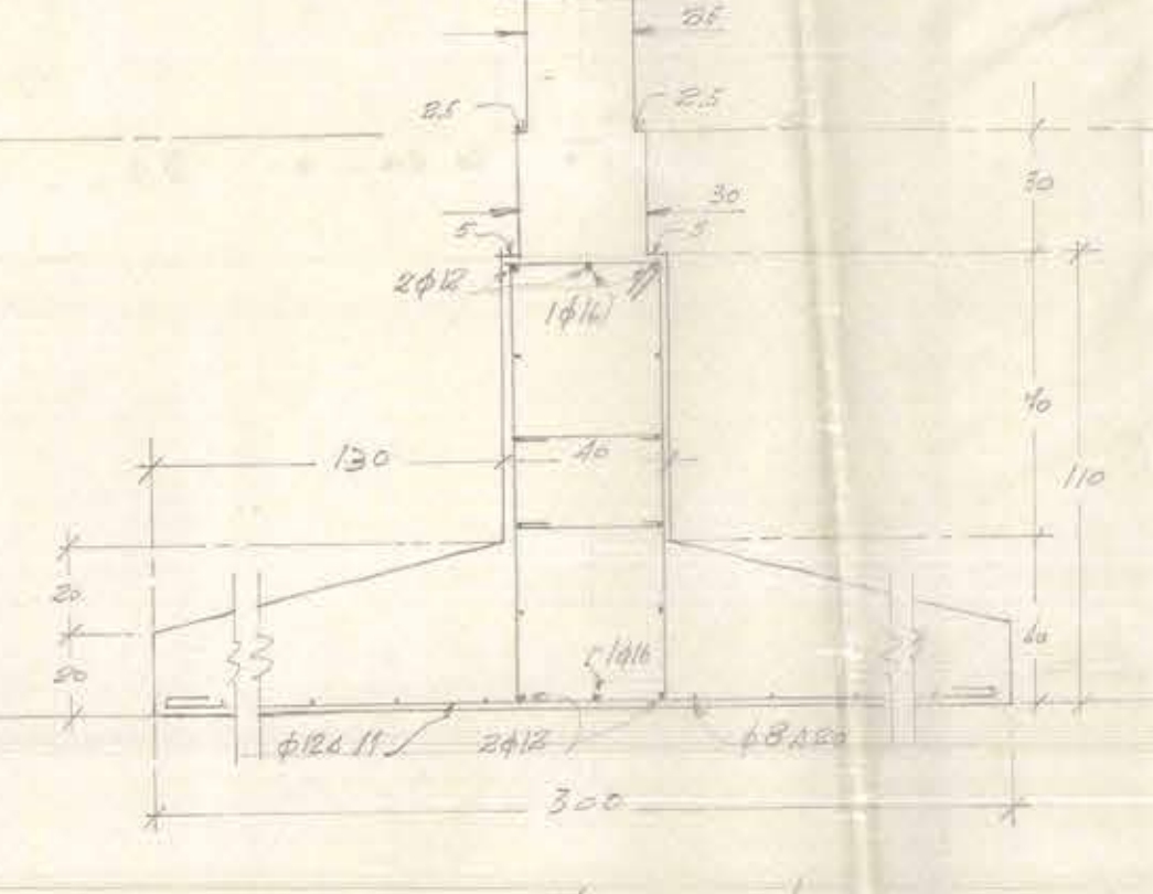
V.F. 40/110 SECC. M-M.
