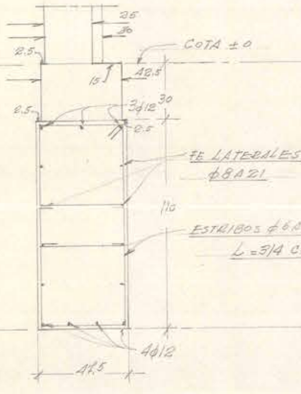
V.F. 40/110 SECC. L-L.
