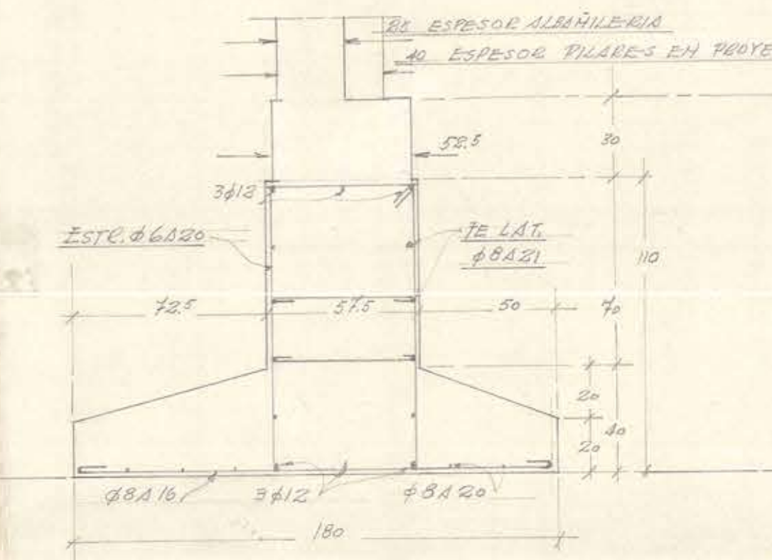
SECCION G-G ALBAÑILERIA EXTERIORES.
