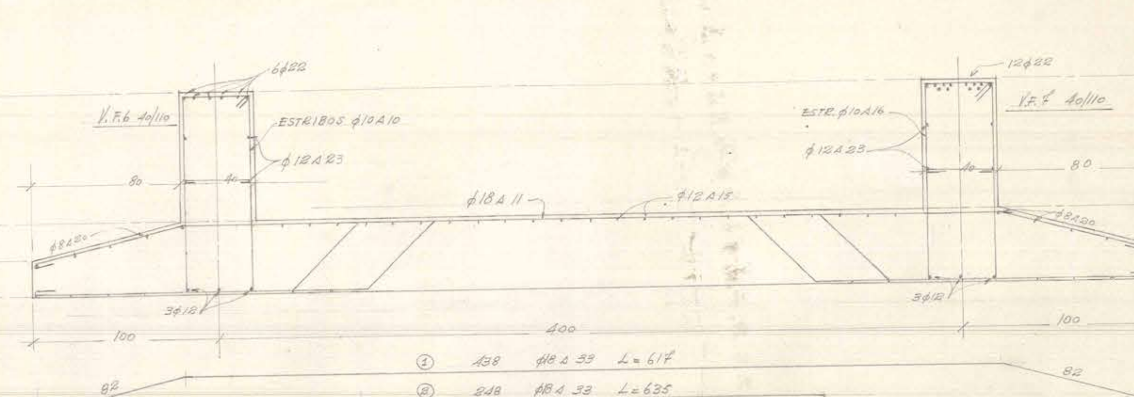
SECCION H-H PLACA FUND. L/40 FE=4800KG. SECCION J-J PLACA FUND. 2x/40 FE=4800KG.
