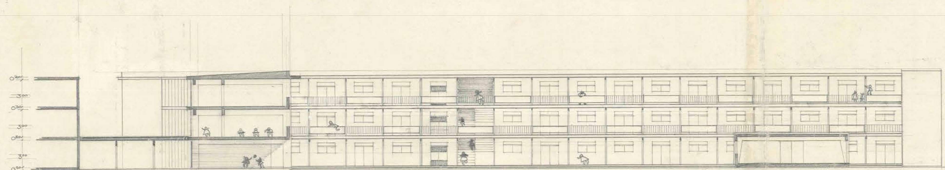
ELEVACION NOR-ORIENTE
