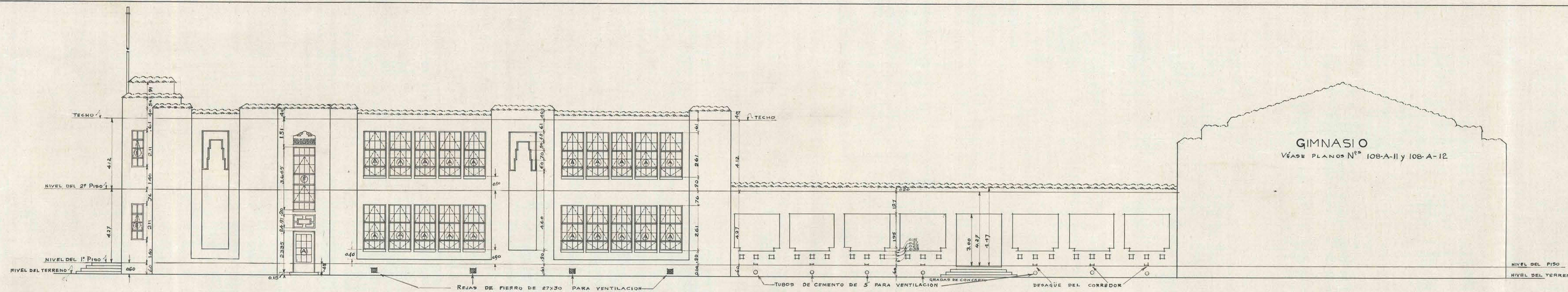
FACHADA LATERAL DERECHA
