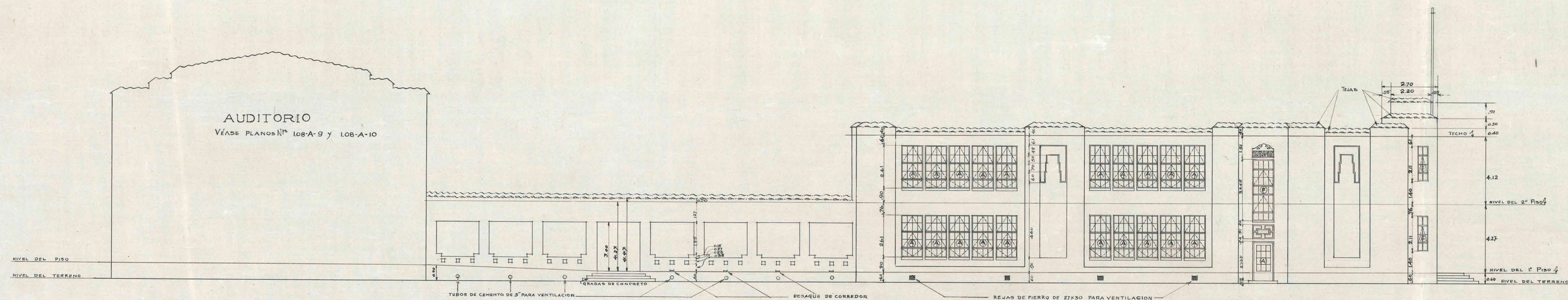
FACHADA LATERAL IZQUIERDA
