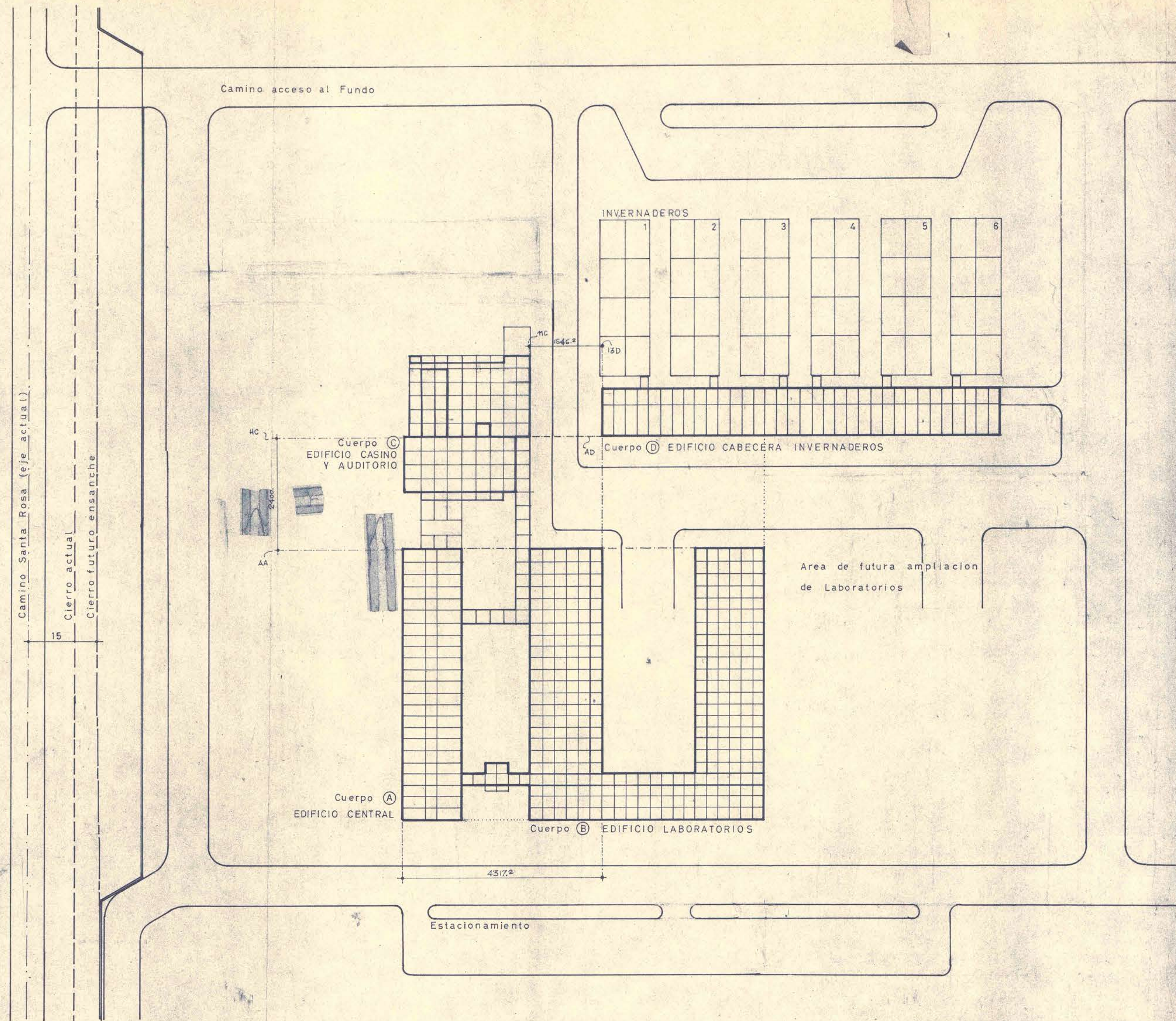
PLANO DE CONJUNTO Y EJES Esc. 1: 500
