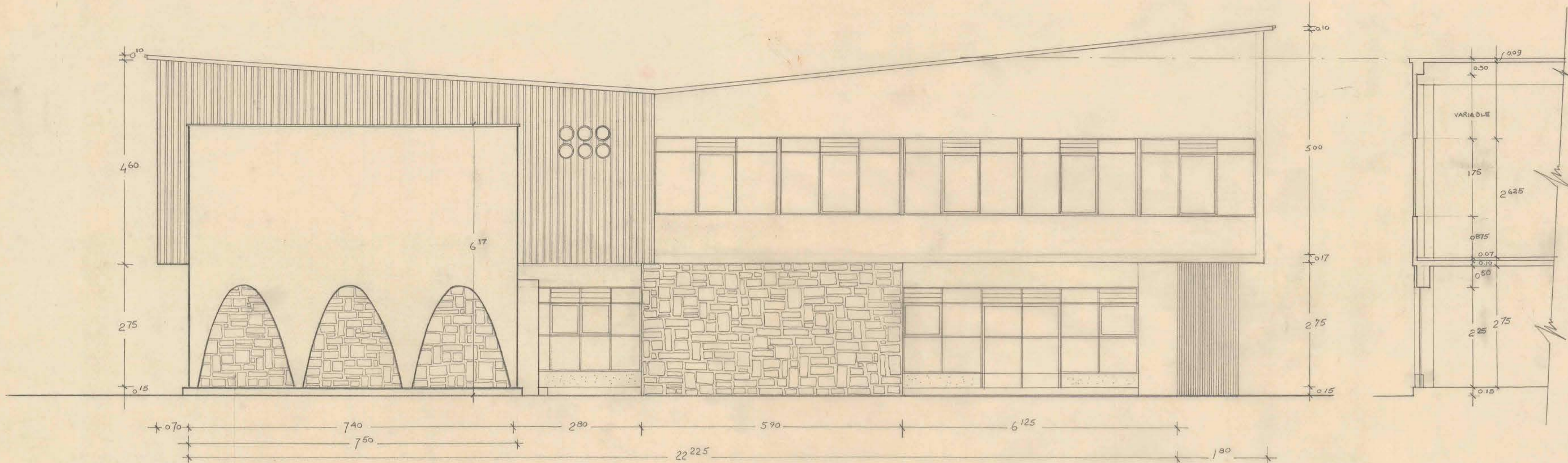
FACHADA SUR-ORIENTE
