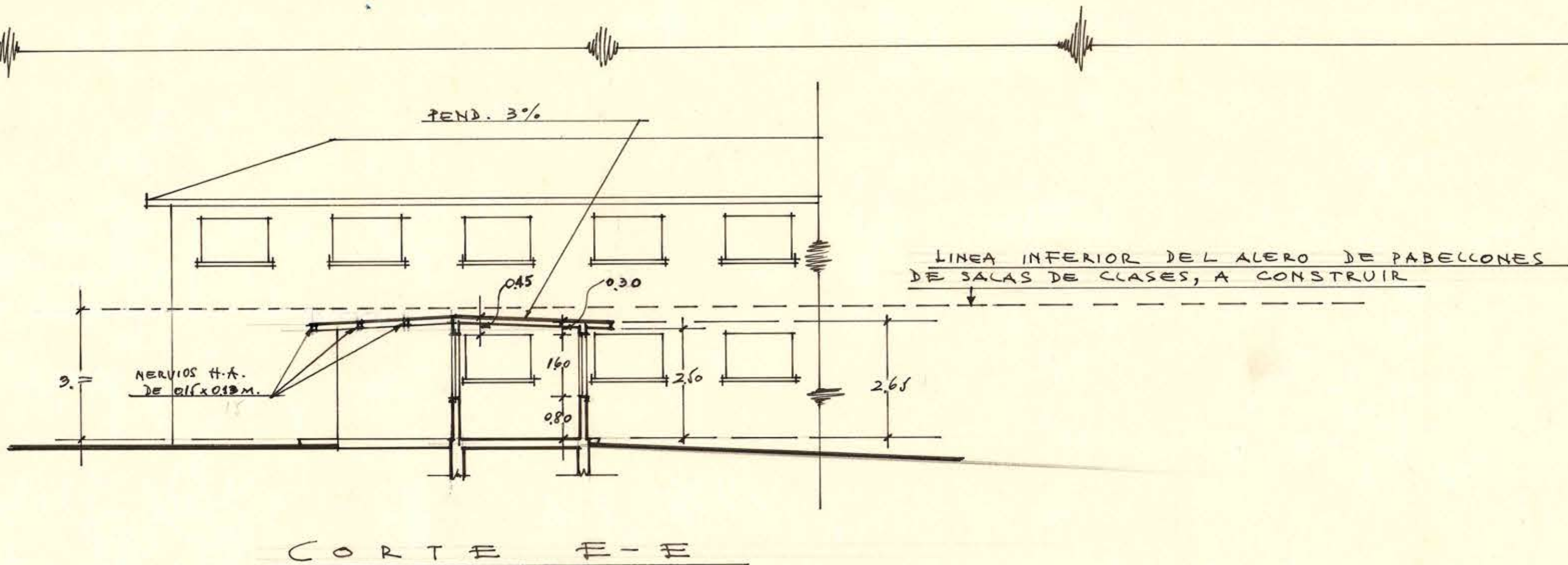
CORTE E-E
