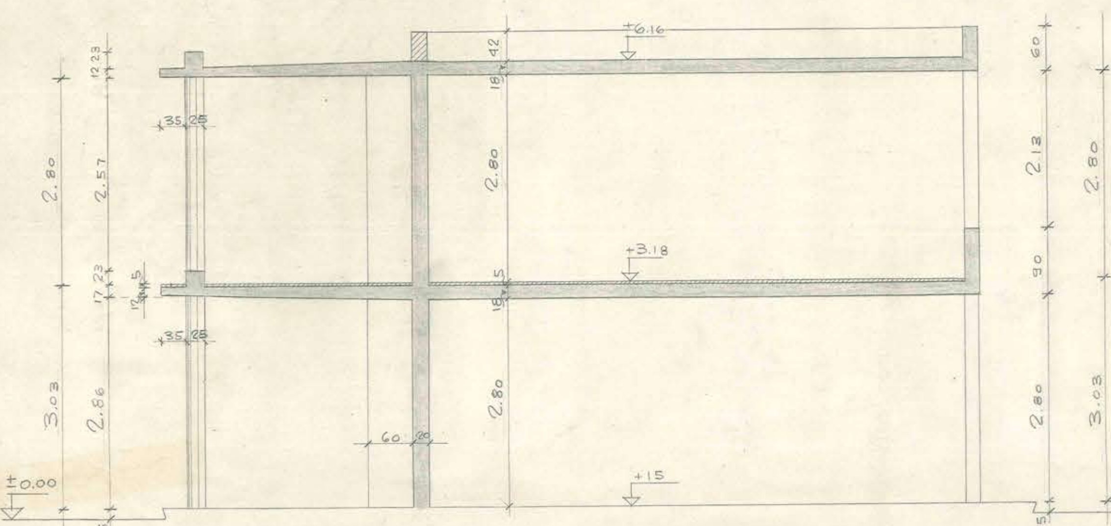
CORTE A-A
