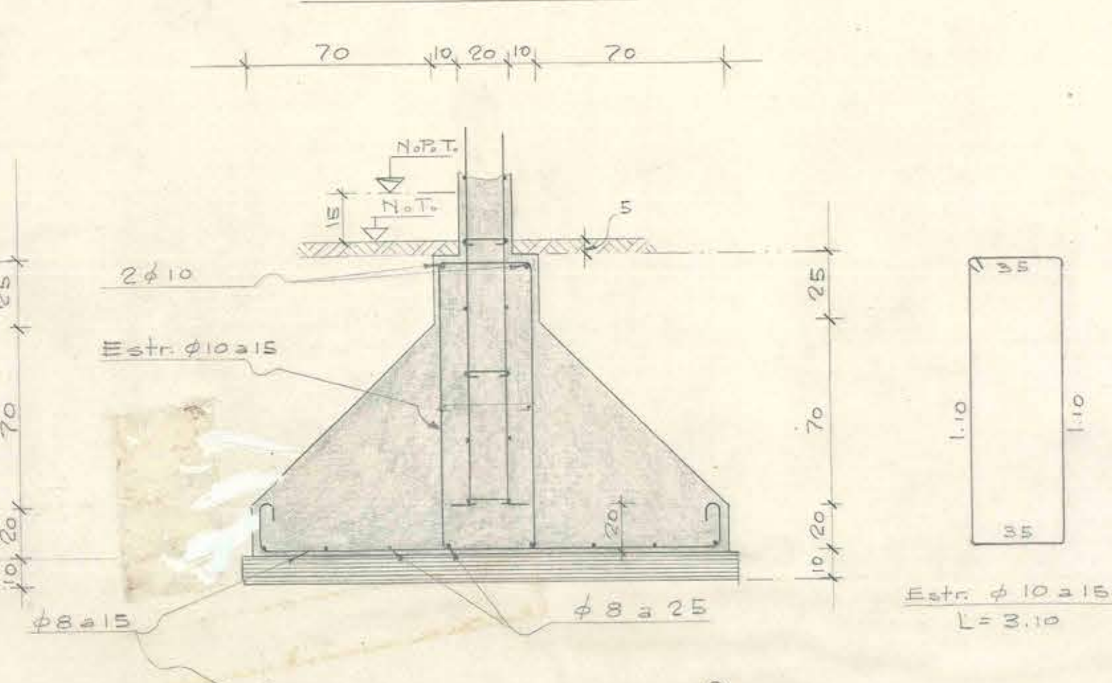
SECCIÓN 3-3
