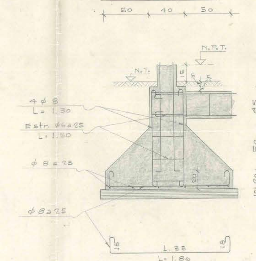
SECCIÓN 2-2
