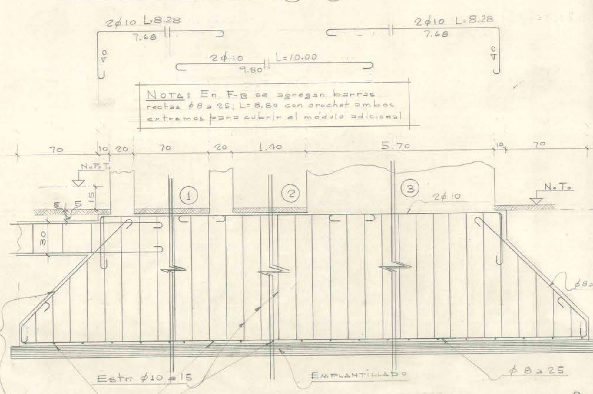
CORTE LONGITUDINAL F-A F-B
