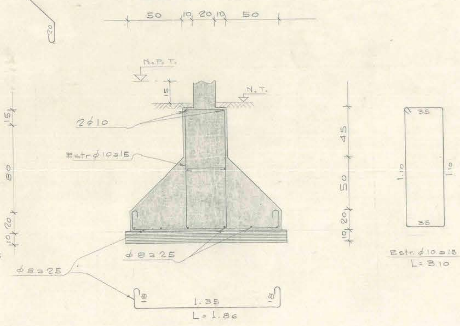
SECCIÓN 4-4
