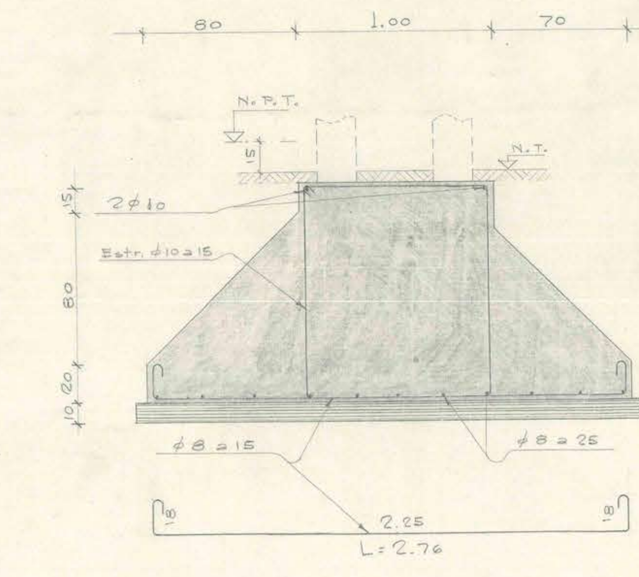
SECCIÓN 6-6
