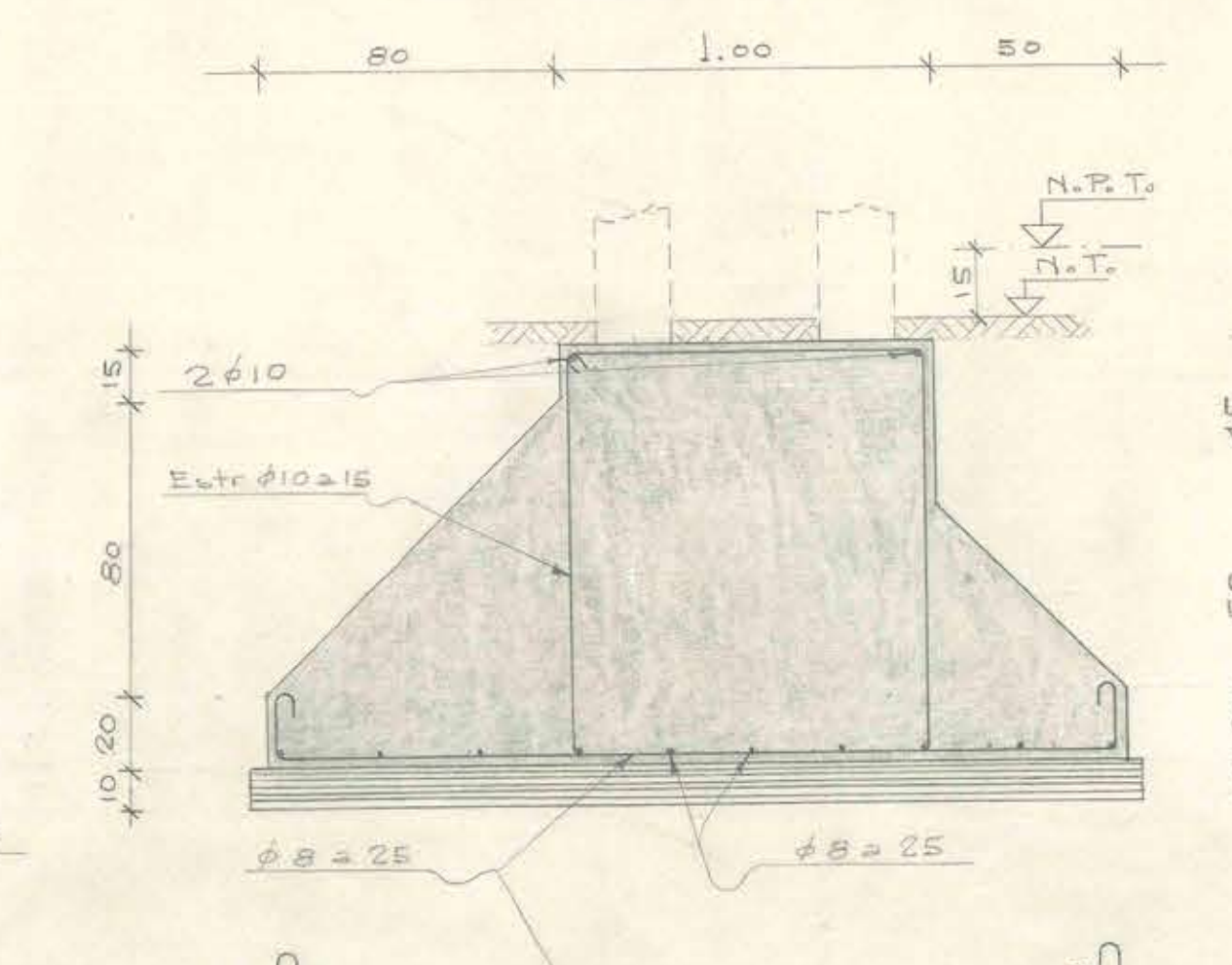
SECCIÓN 5-5
