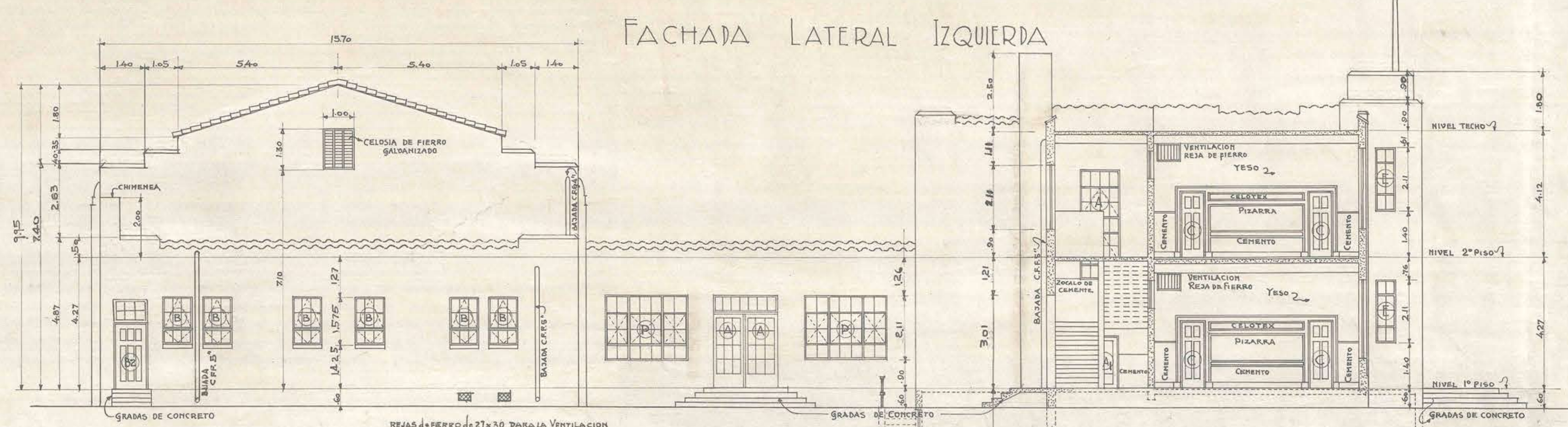
SECCION Y FACHADA INTERIOR
