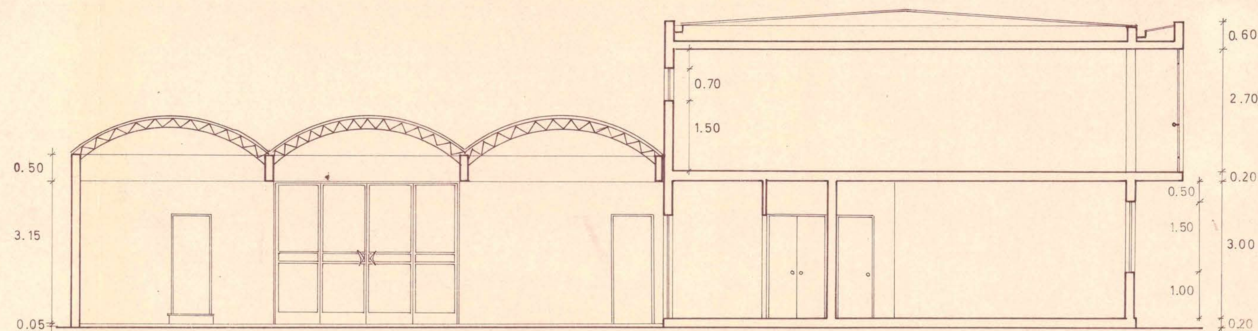
CORTE B-B.
