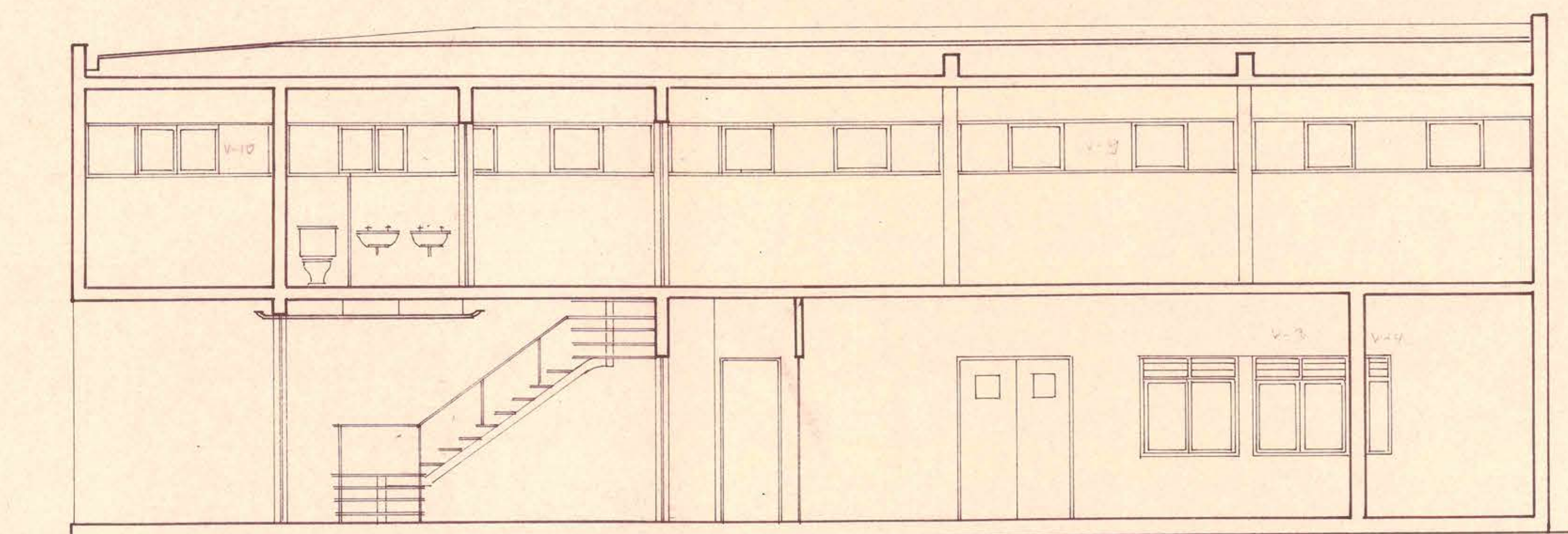
CORTE A-A.
