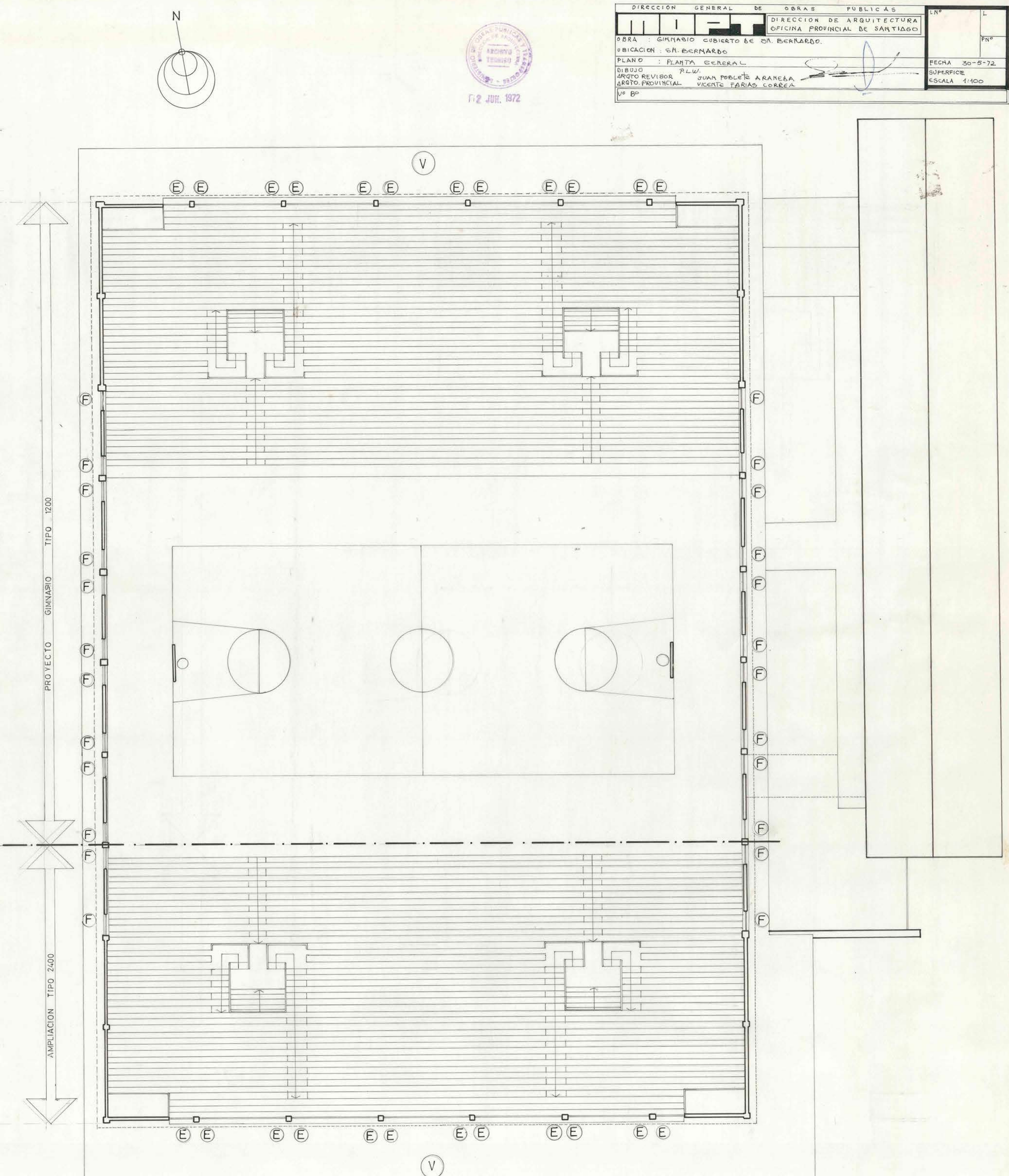
PLANTA esc. 1:100
