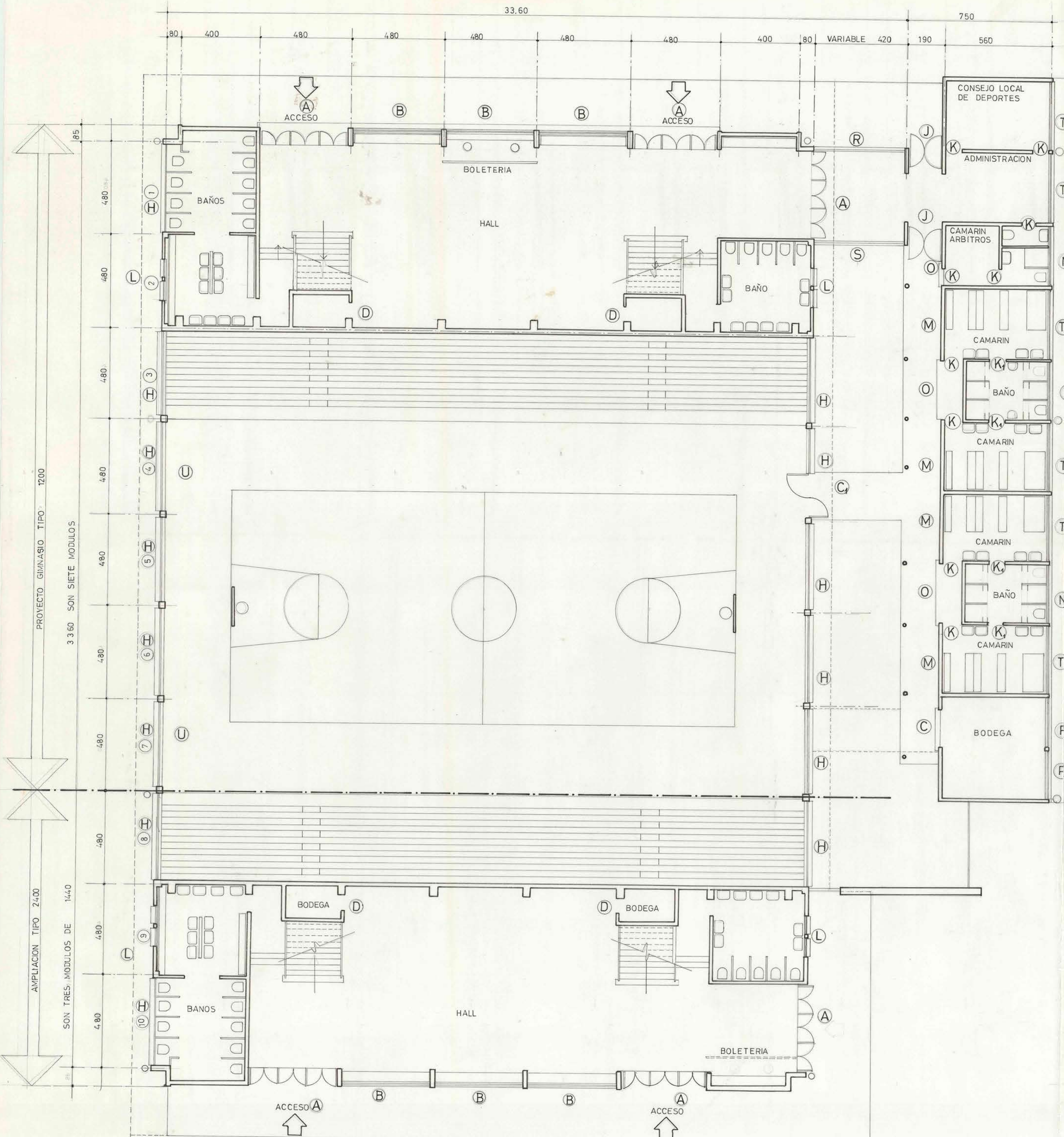
PLANTA esc. 1:100
