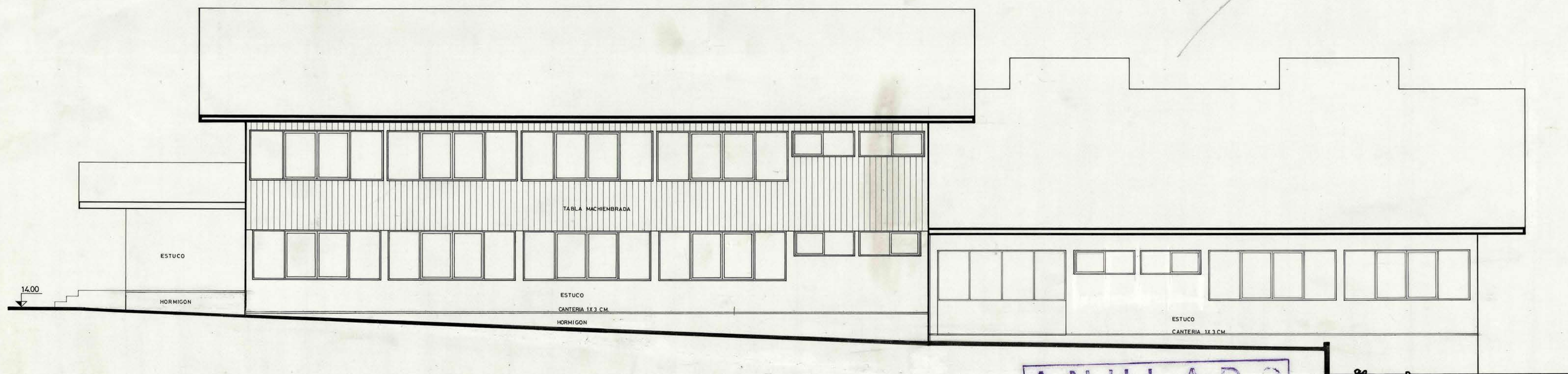
FACHADA POSTERIOR
