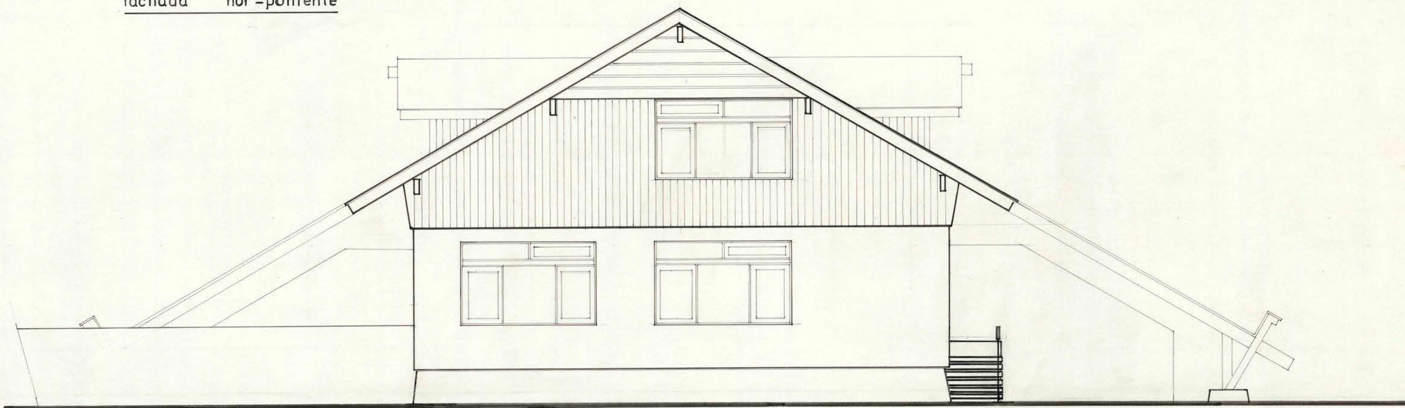
fachada nor-poniente
