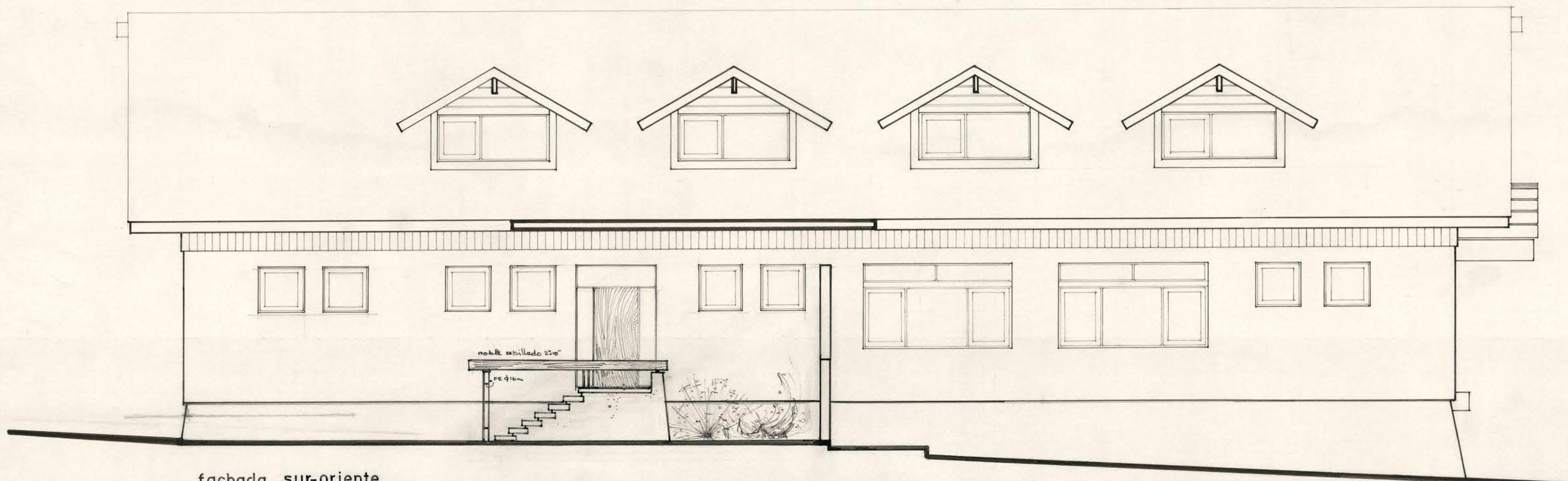
fachada sur-oriente
