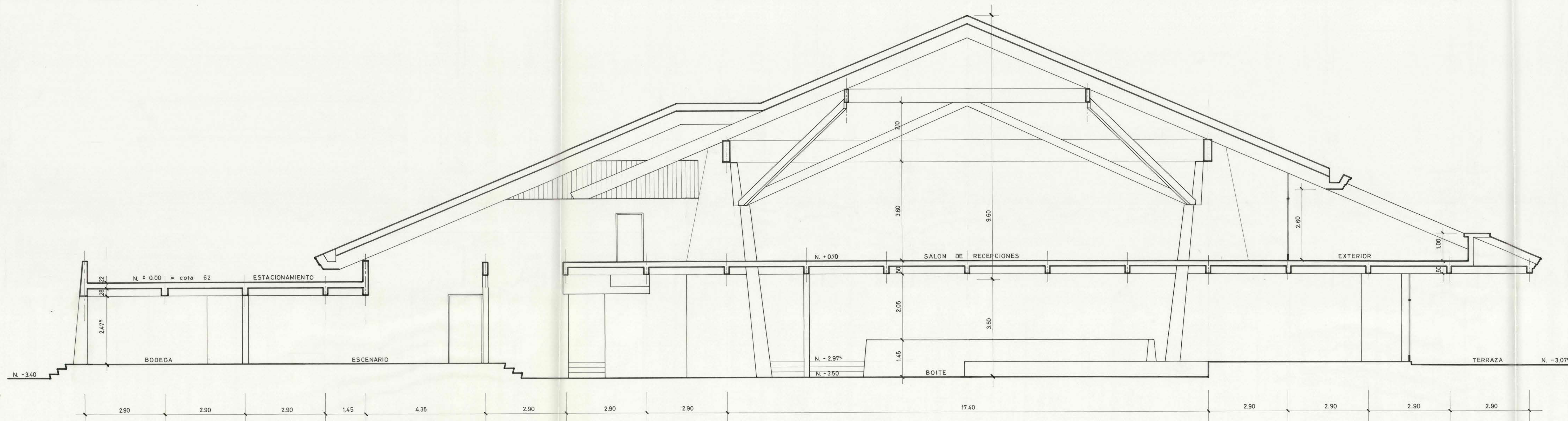
SECCION 4-4.
