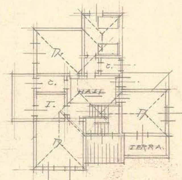
SEGUNDO PISO
