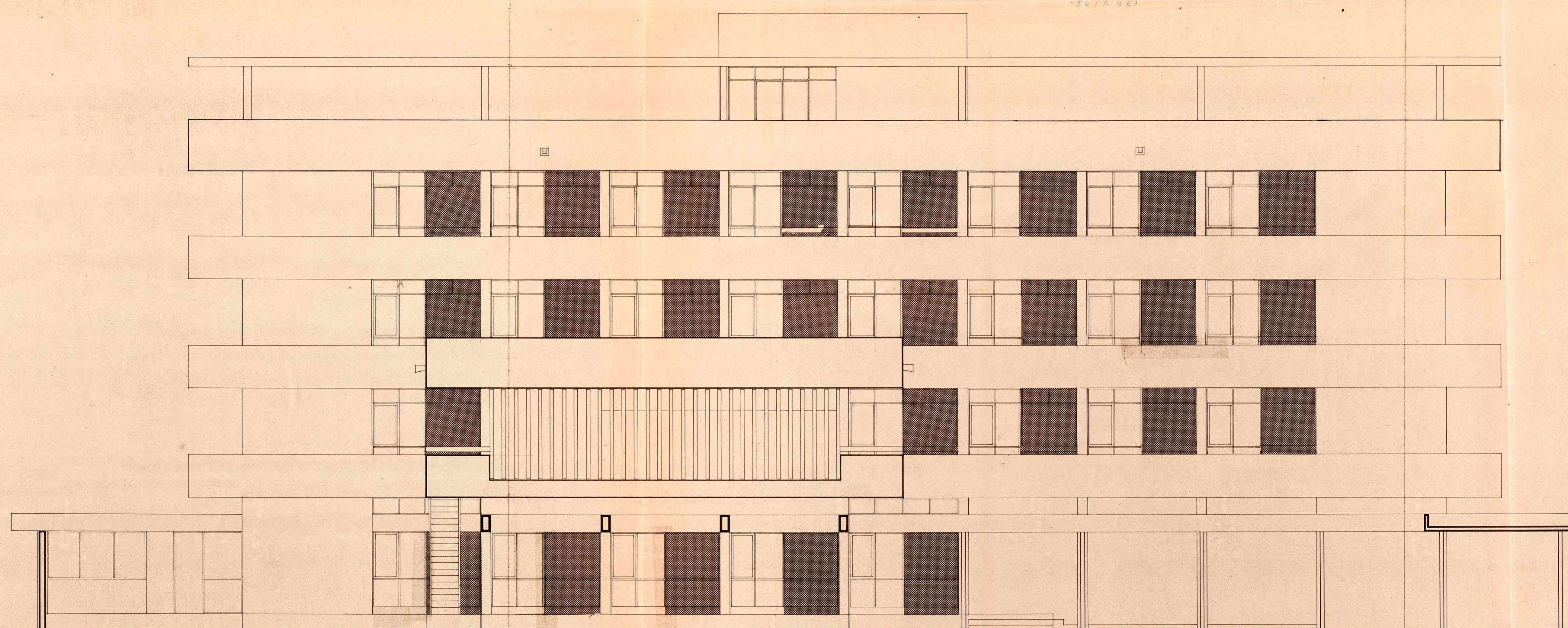
ELEVACION SUR-PONIENTE
