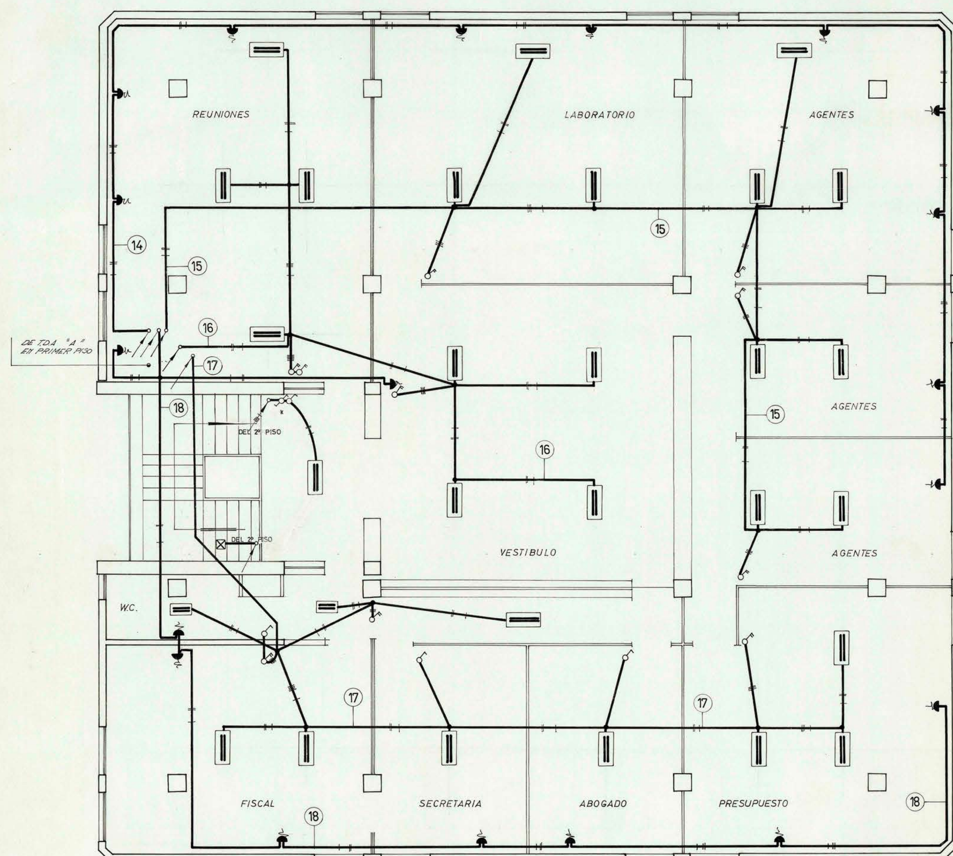
PLANTA TERCER PISO
