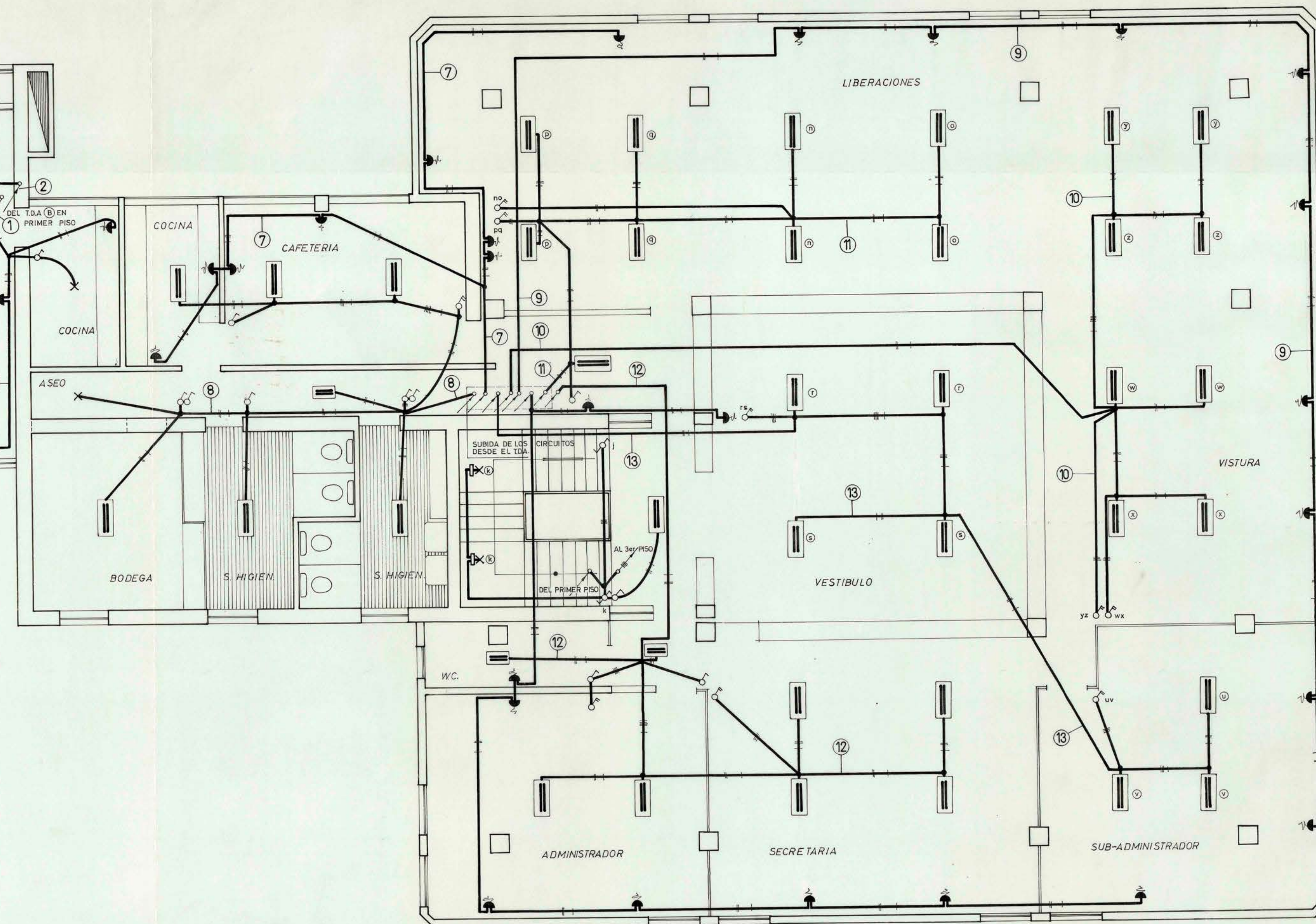
PLANTA SEGUNDO PISO
