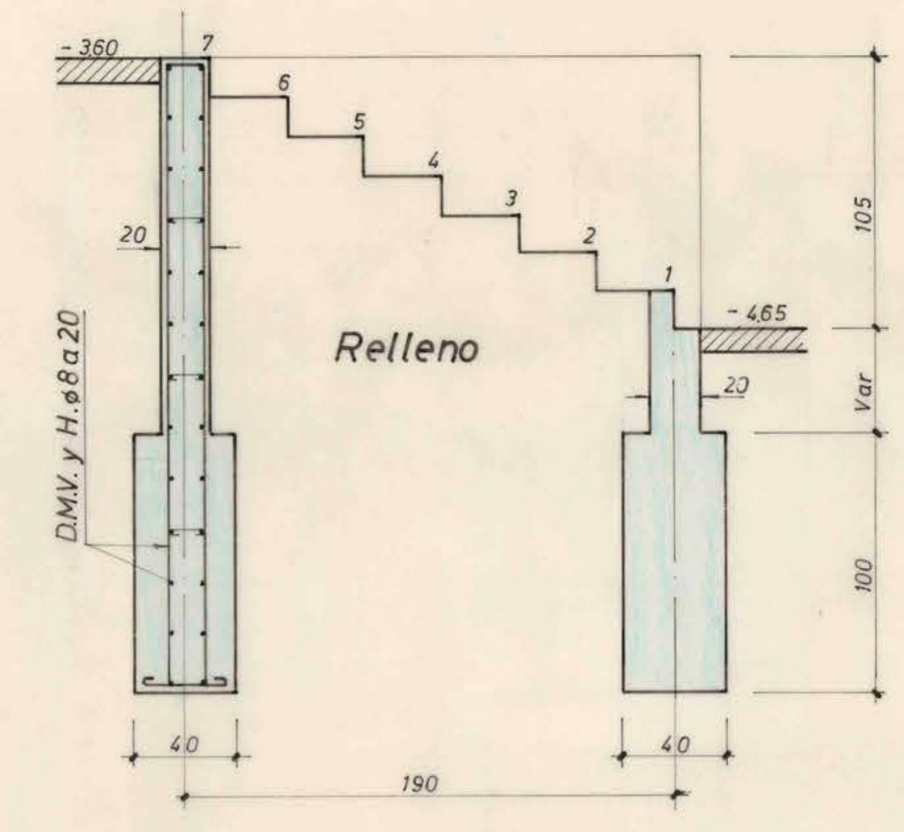
Corte Y-Y
