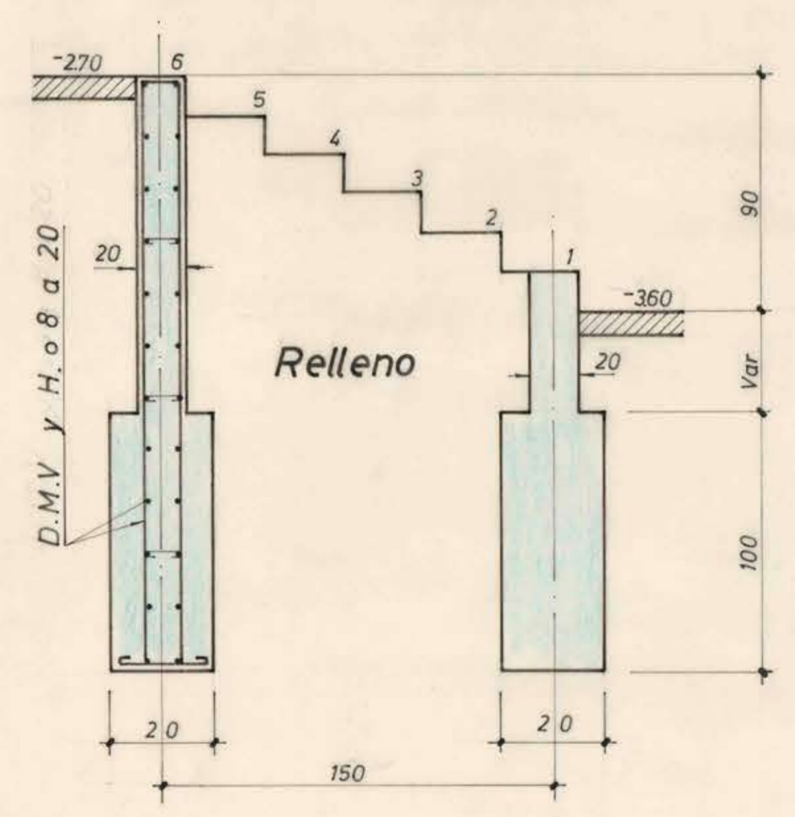
Corte Z-Z
