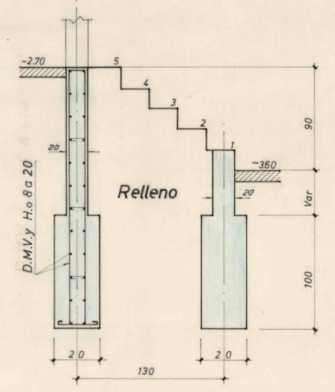
Corte X-X
