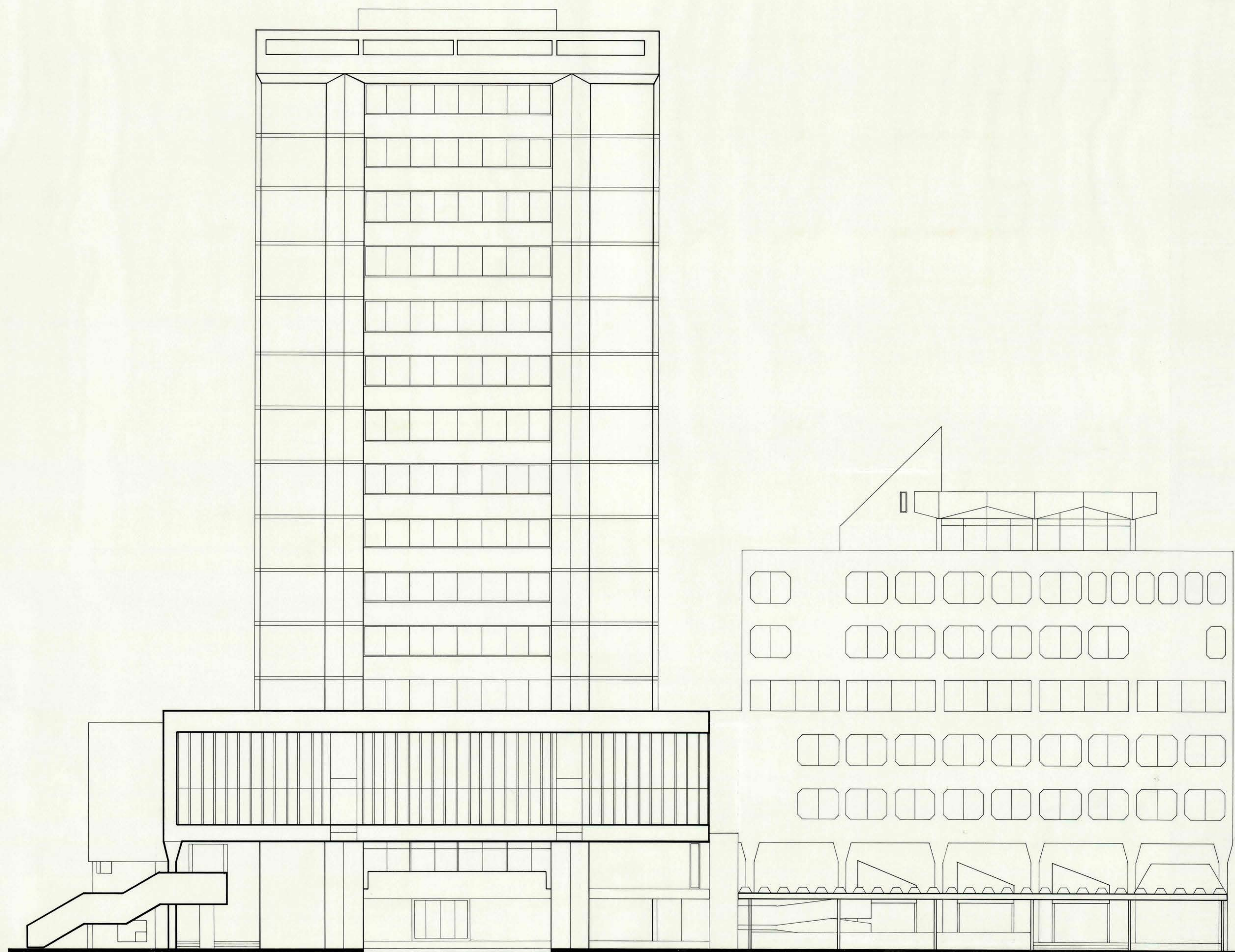
ELEVACION SUR PONIENTE
