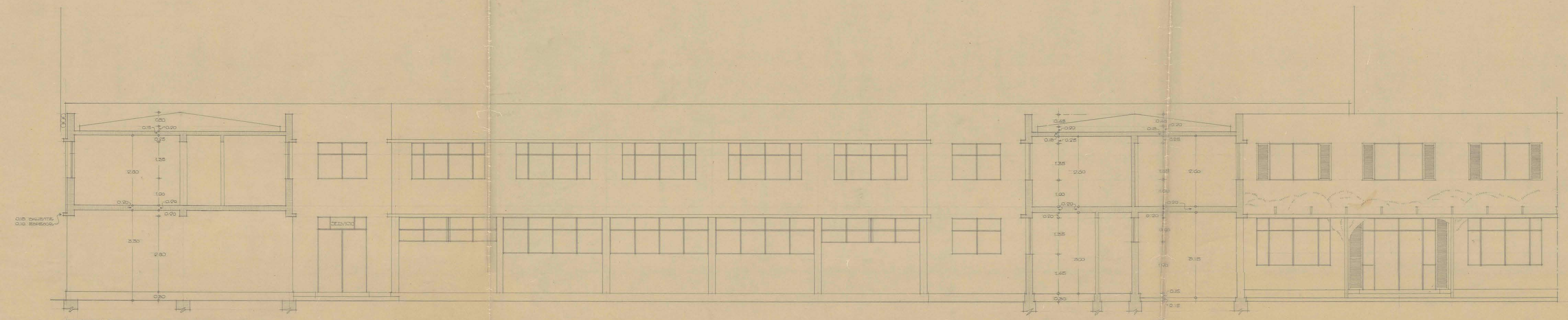
CORTE PARALELO A CALLE O'HIGGINS.
