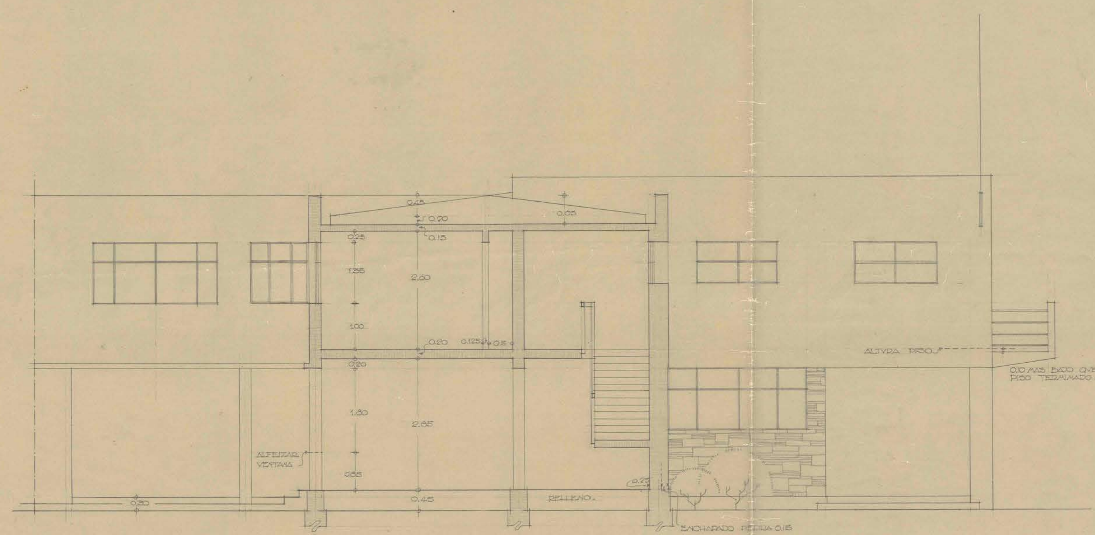
CORTE POR CASA GOBERNADOR.
