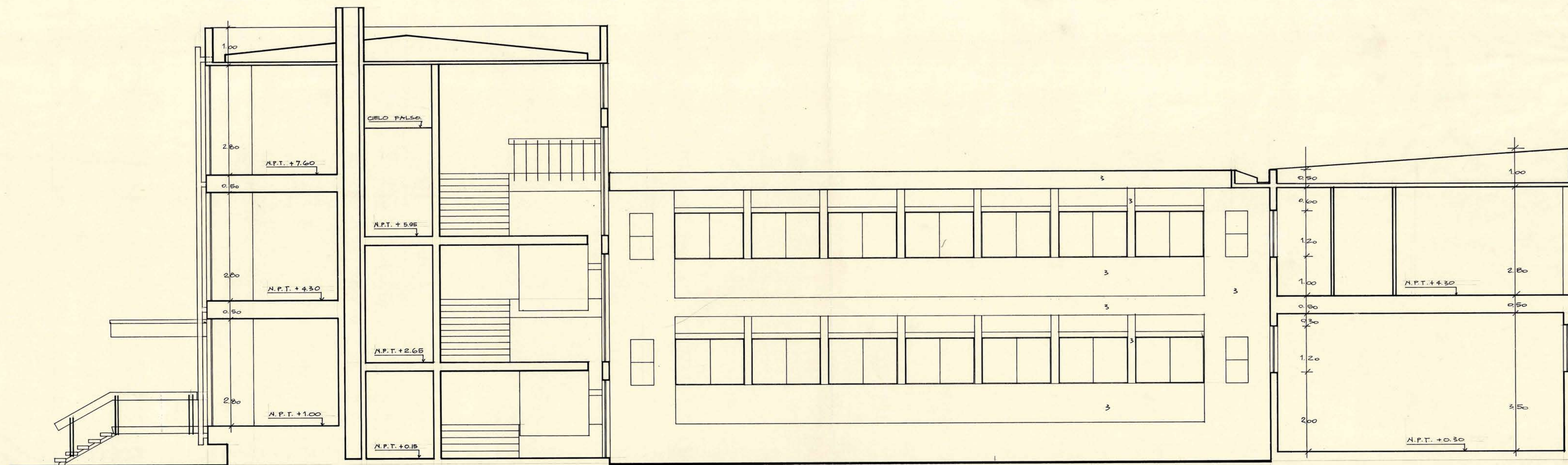
CORTE 9-10 FACHADA ORIENTE
