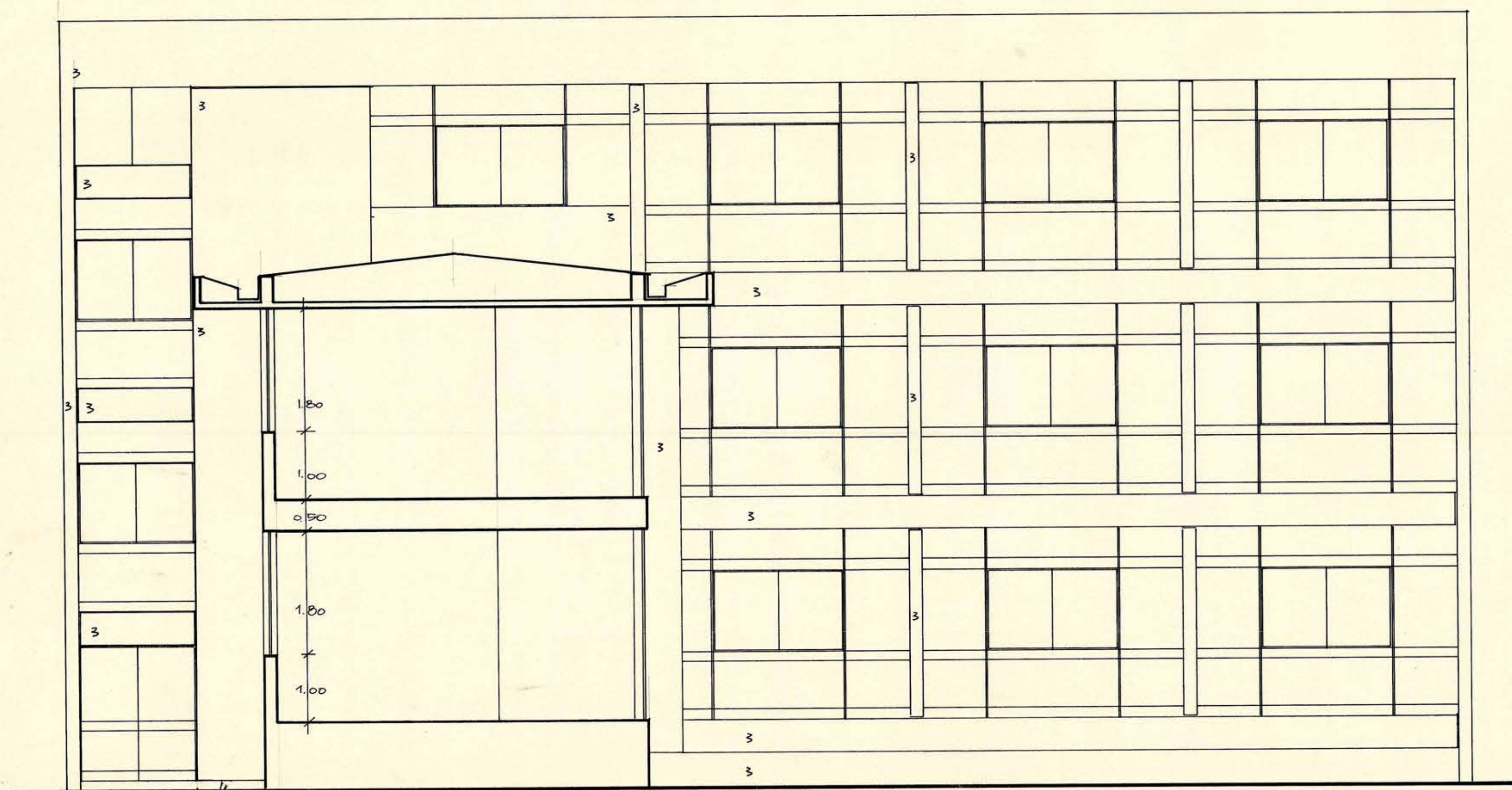
CORTE 5-6 FACHADA NORTE INTERIOR
