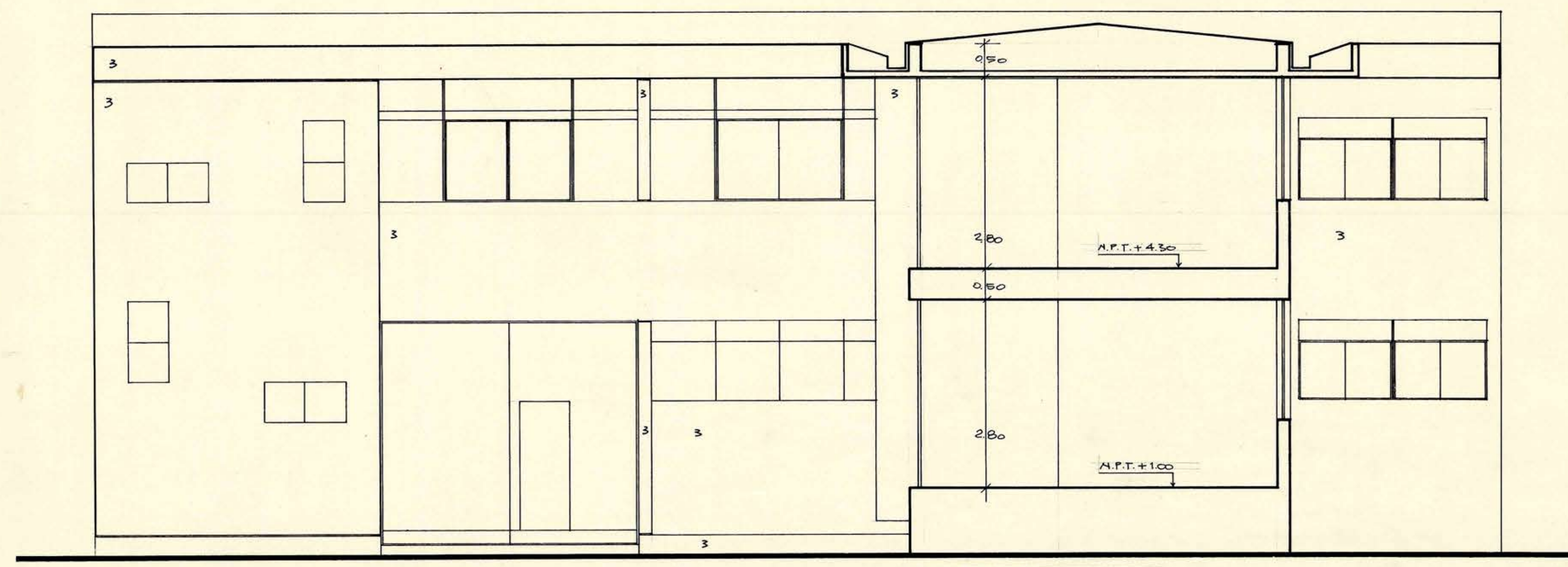
FACHADA SUR INTERIOR CORTE 7-8
