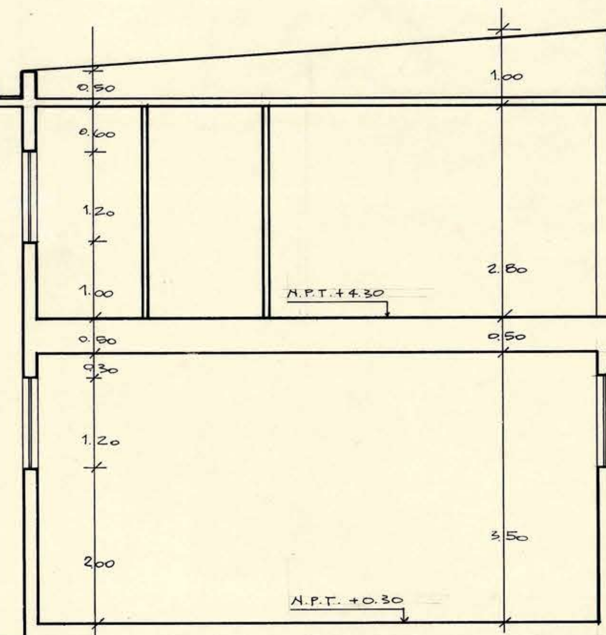
CORTE 11-12
