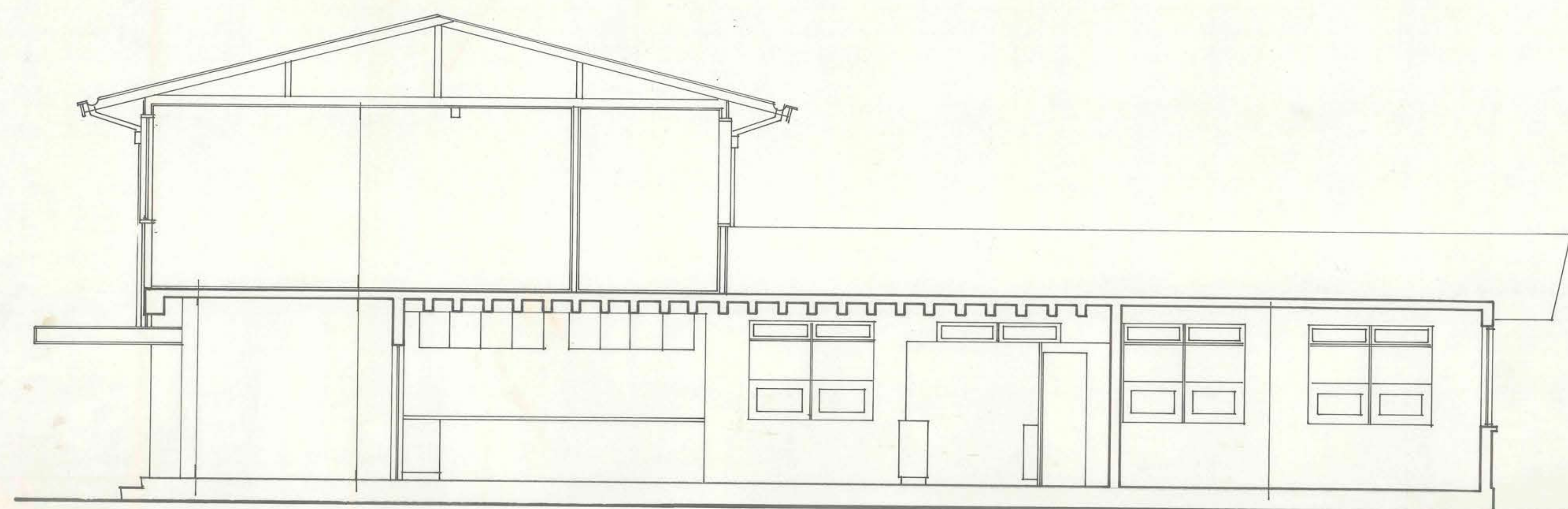
CORTE ESQUEMATICO AA
