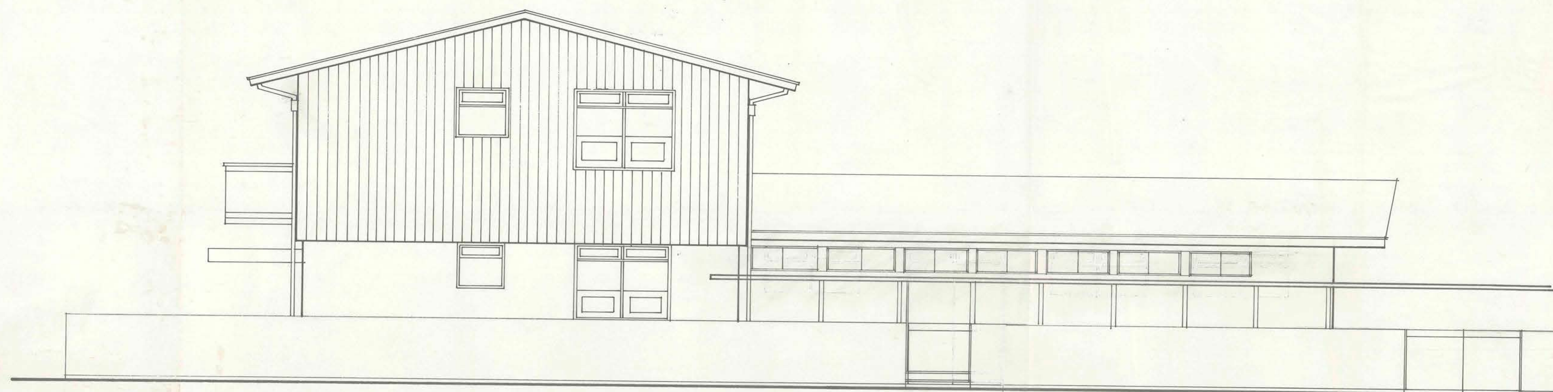
ELEVACION PONIENTE LATERAL
