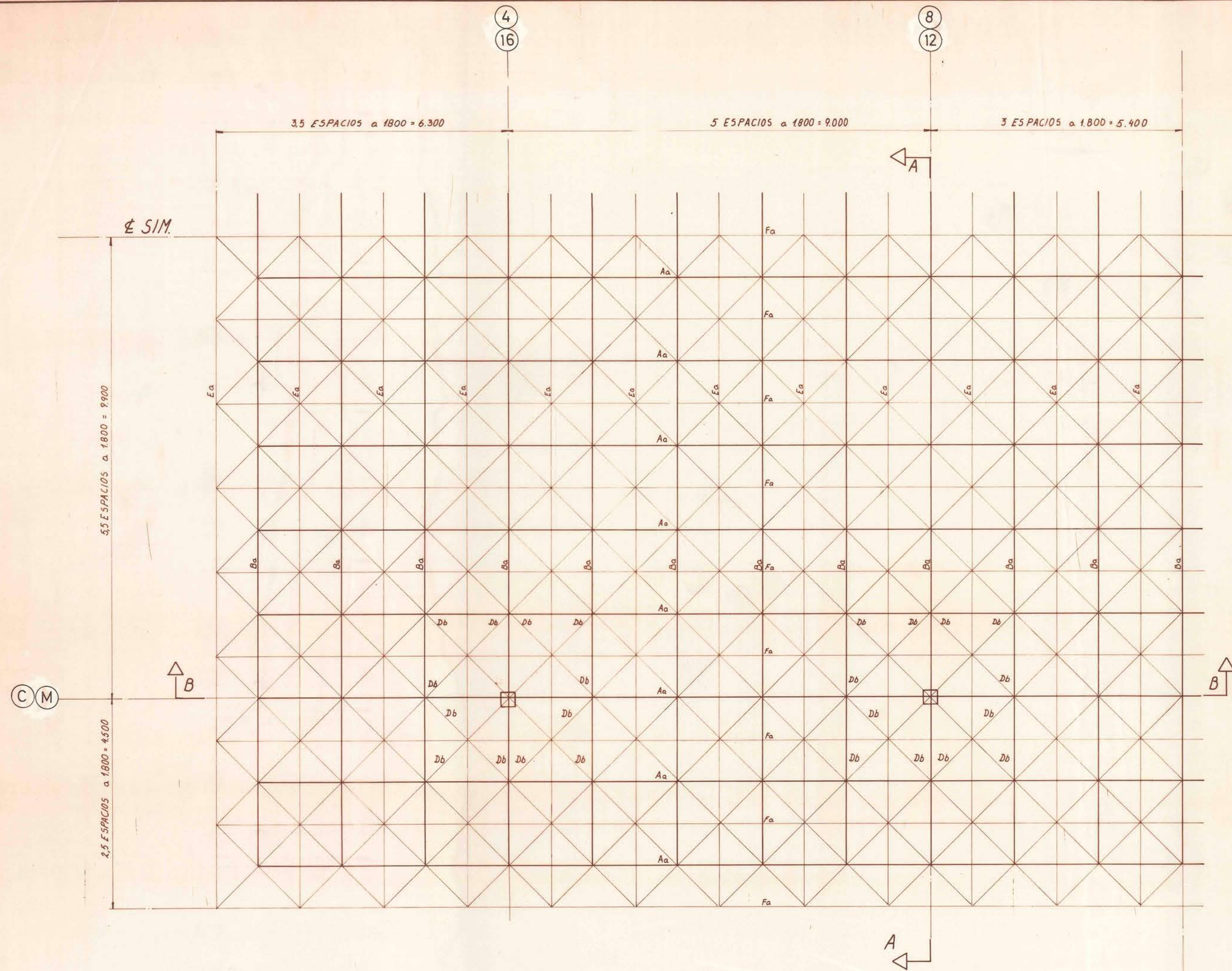
1/4 PLANTA GENERAL
