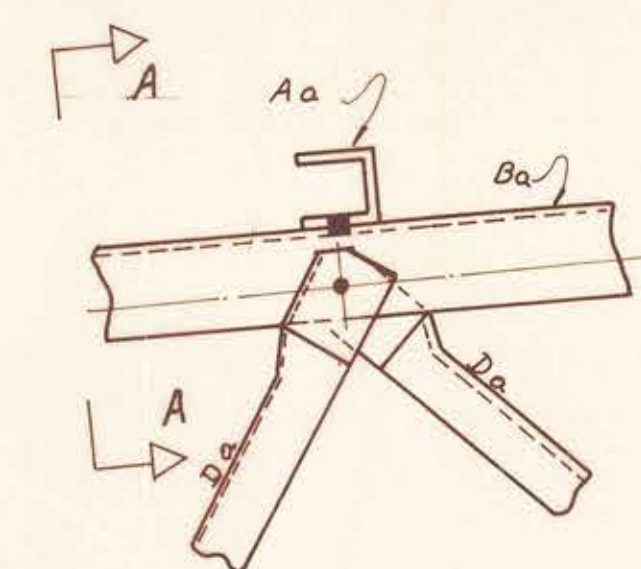
DET. NUDO SUP. TIP
