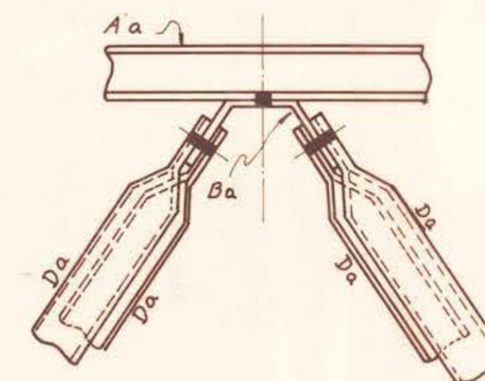
SECCION A-A
