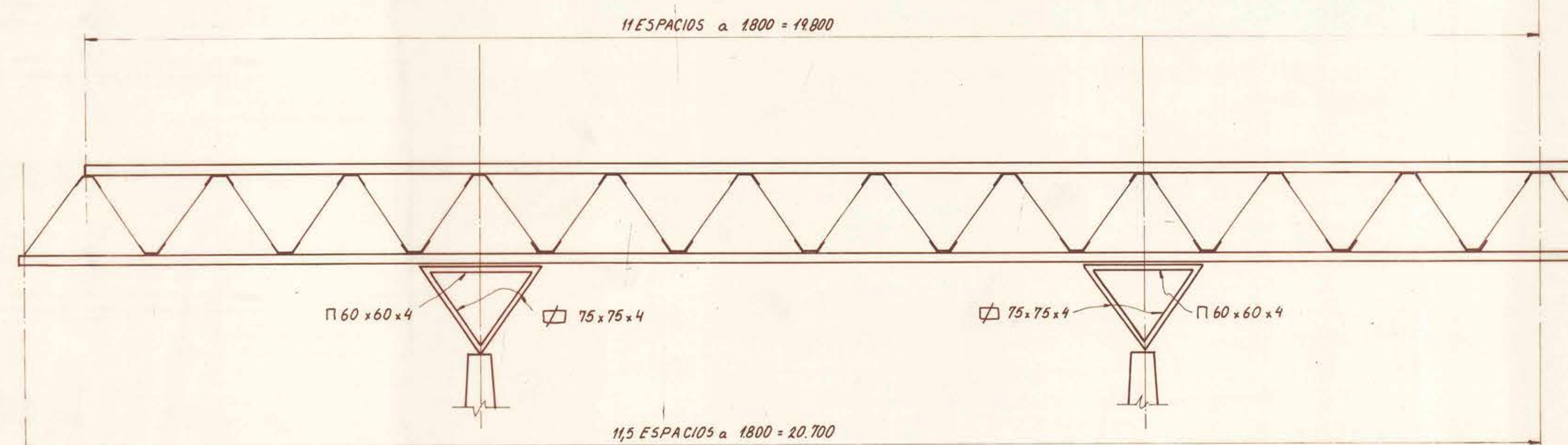
SECCION B-B
