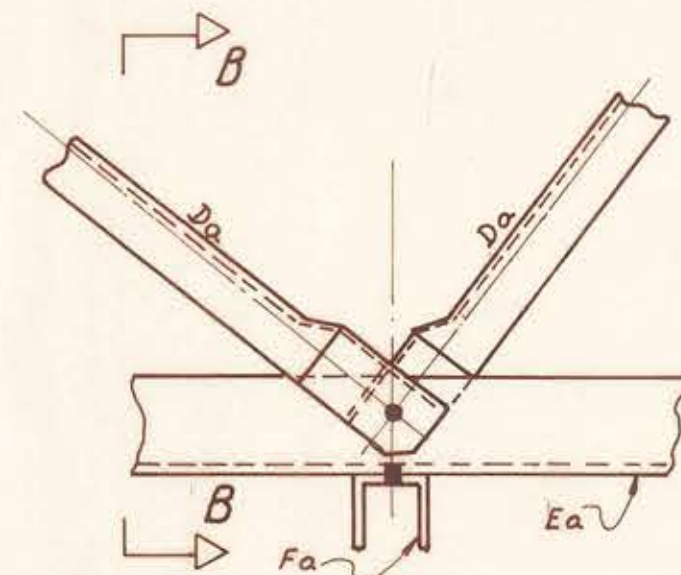
DET. NUDO INF. TIP
