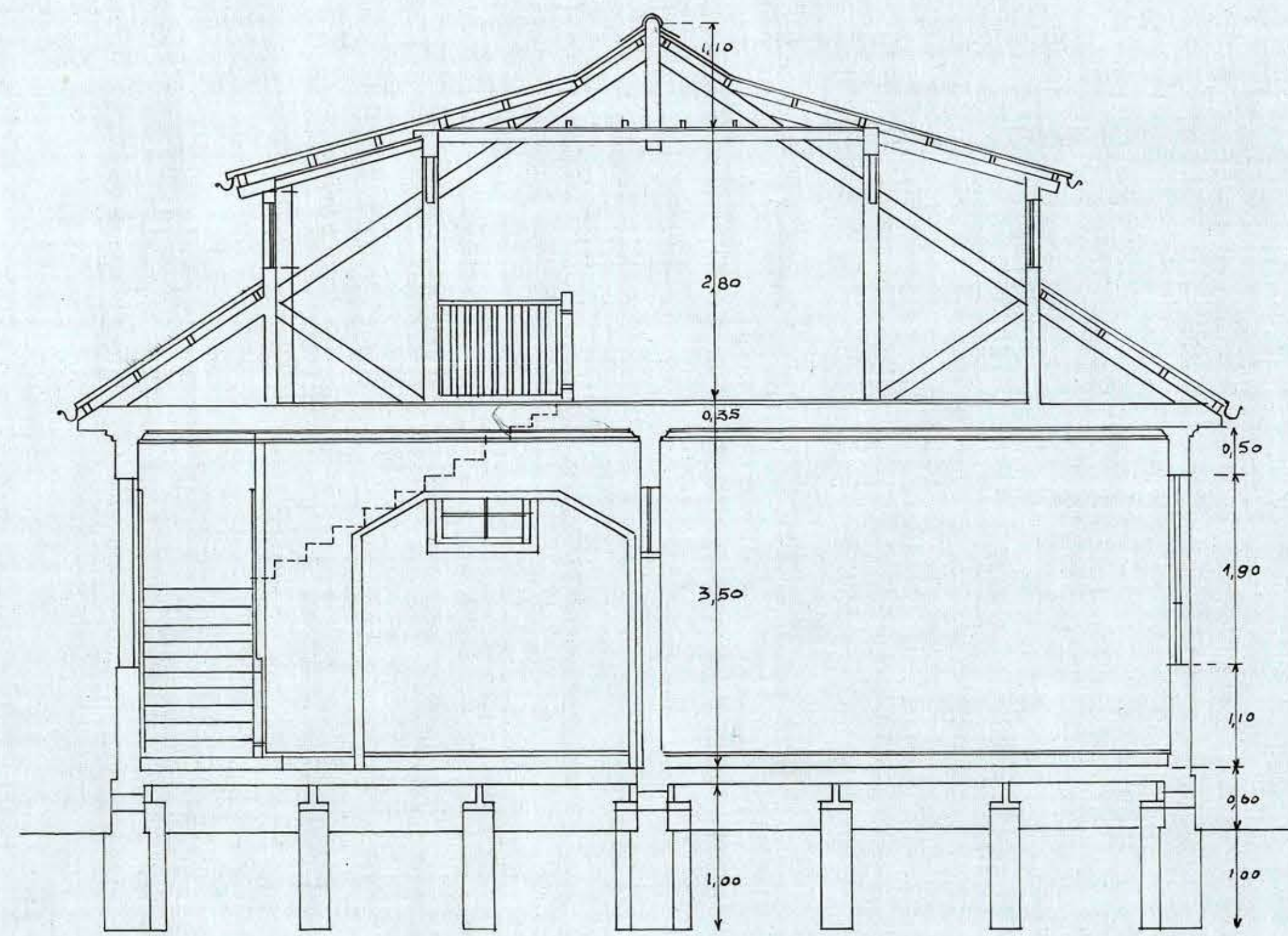
SECCIÓN TRANSVERSAL
