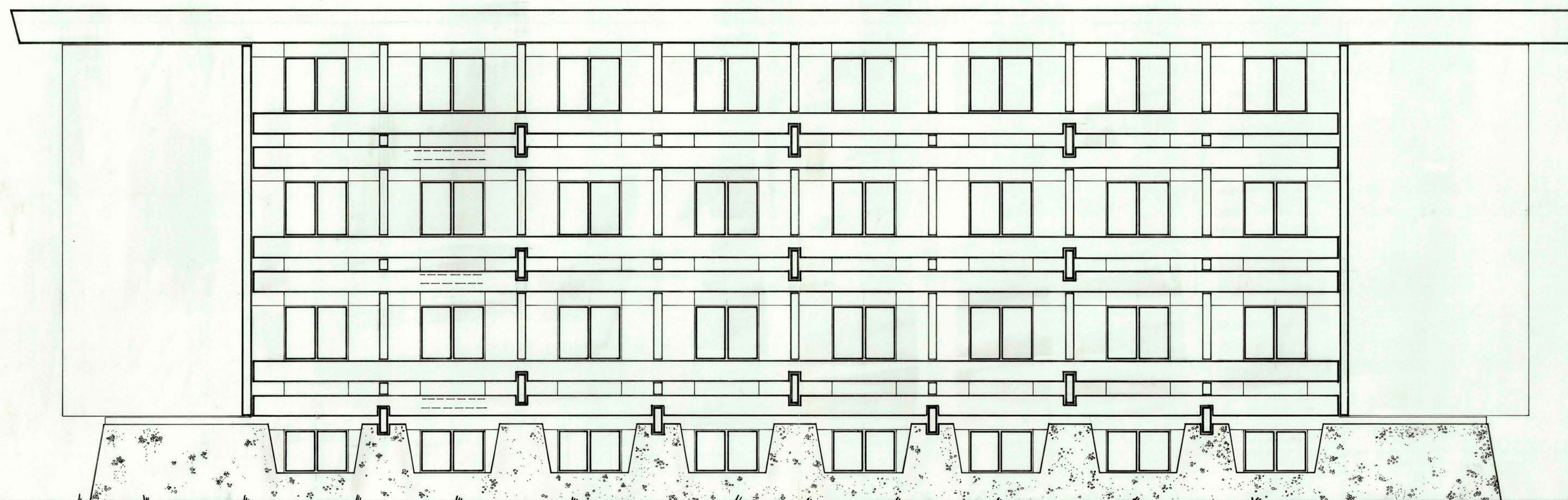
ELEVACION SUR PONIENTE (a calle balmaceda)
