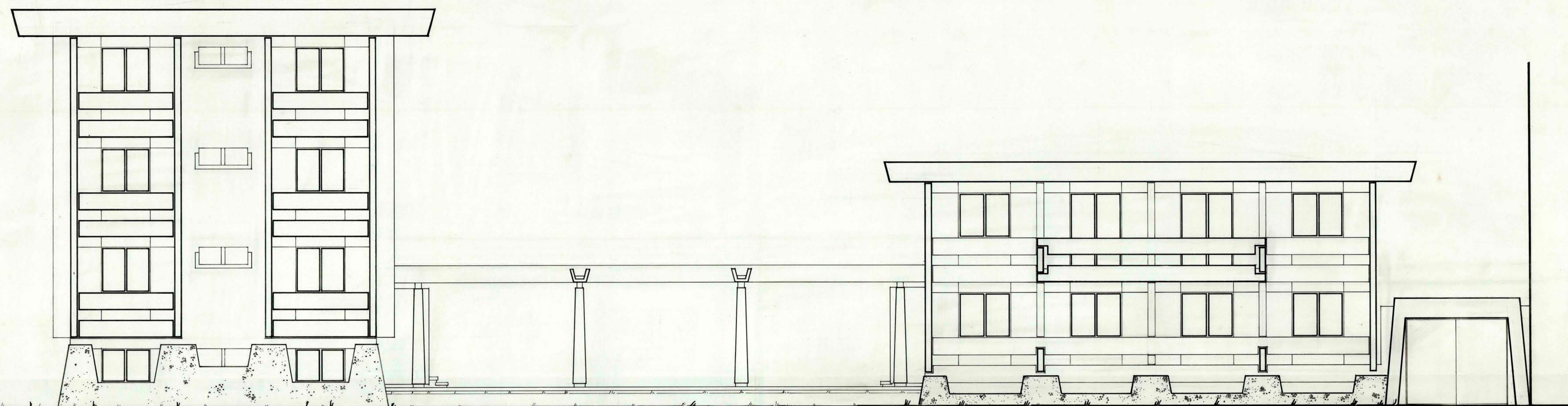
ELEVACION SUR ORIENTE (a calle manuel montt)
