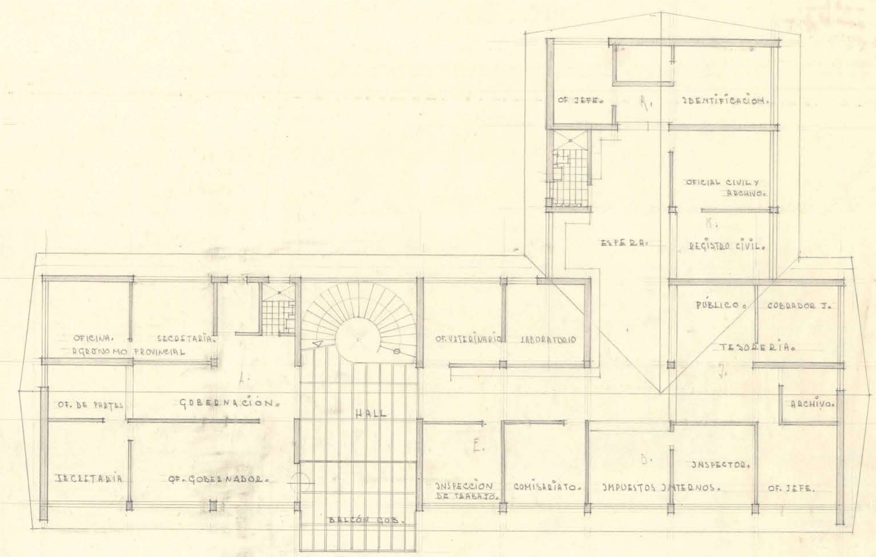
PLANO DEL SEGUNDO PISO...
