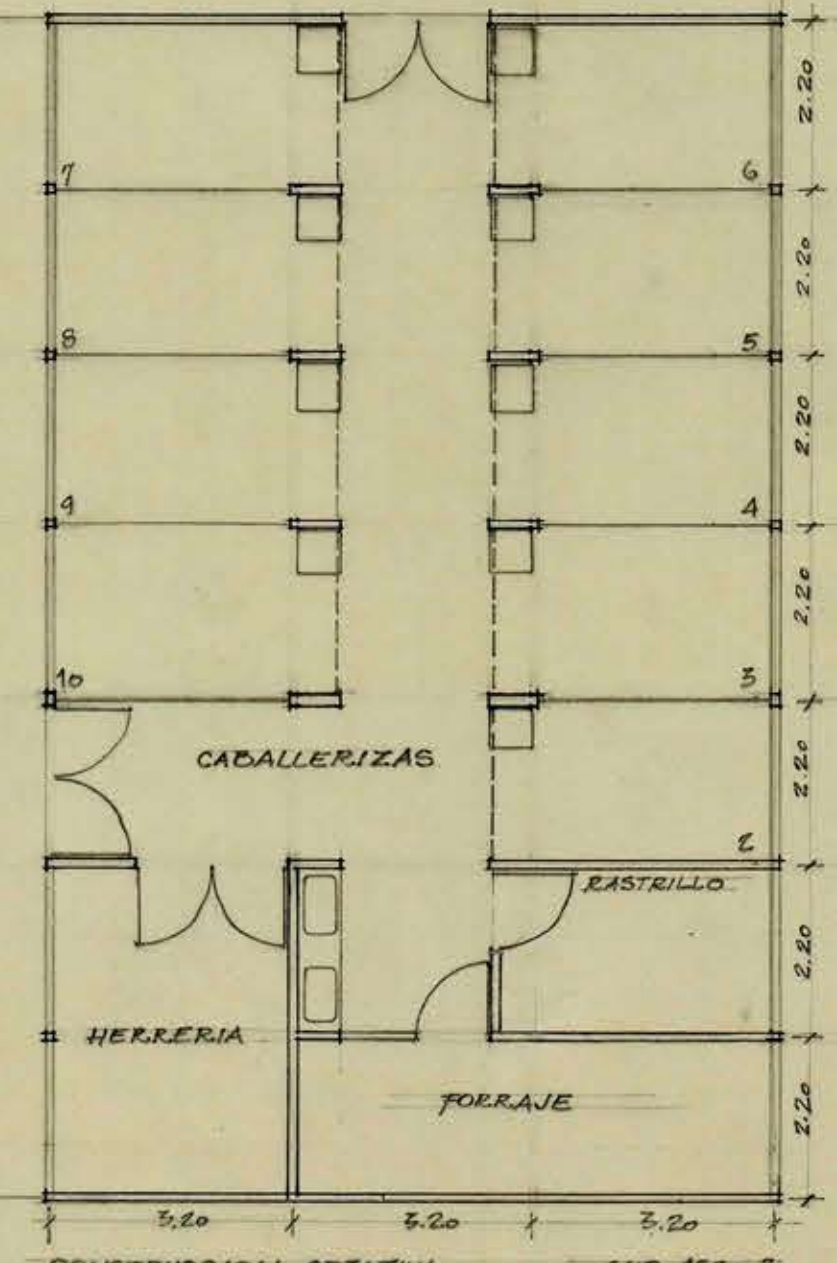
CONSTRUCCION OPTATIVA SUP. 156m 2
