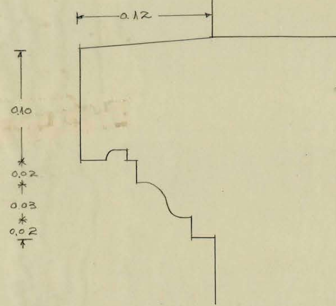
MOLDURA BALCON
