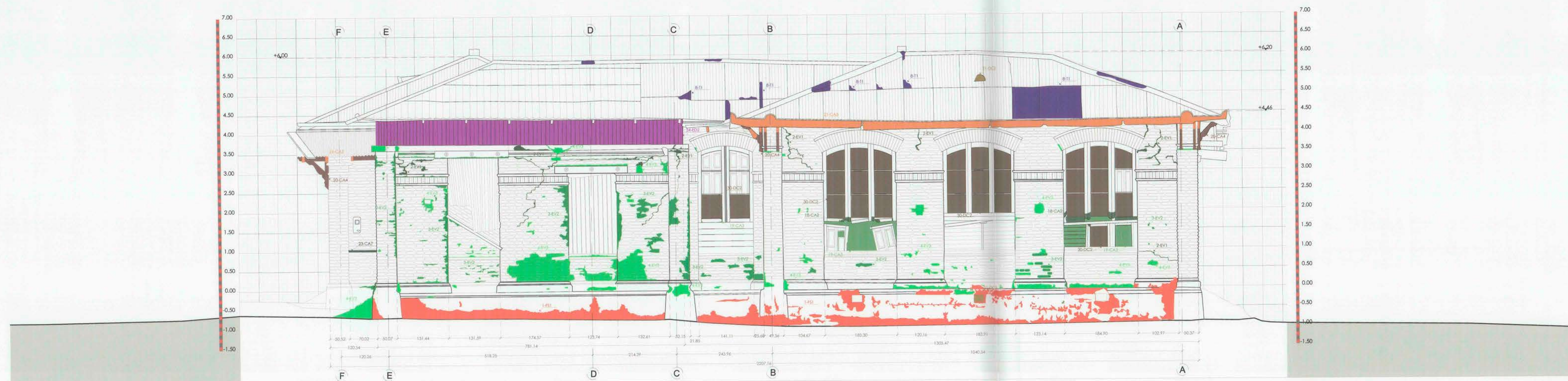
ELEVACIÓN NORTE Escala 1 : 50
