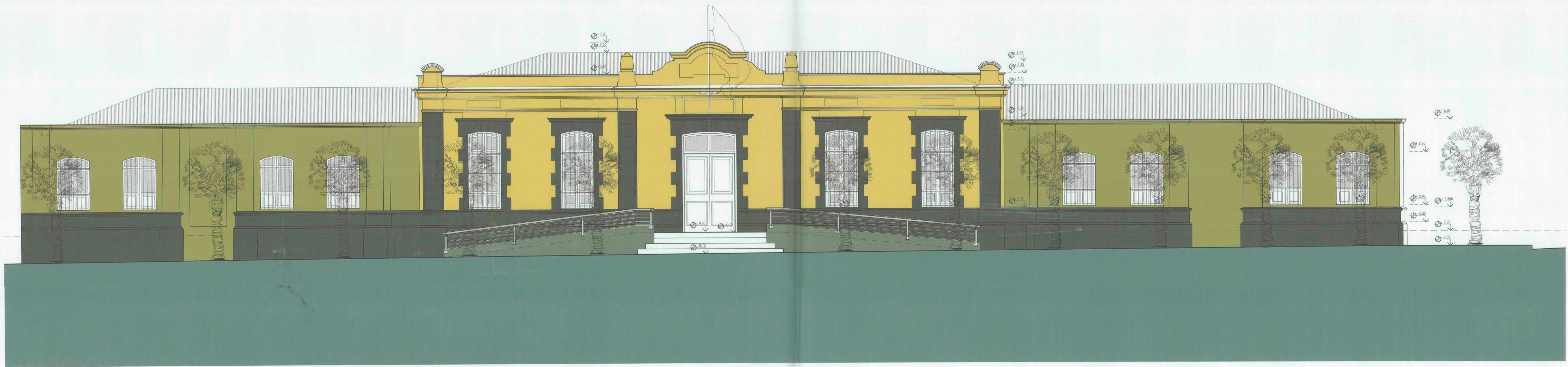
ELEVACION SUR (MERCED) ESC. 1:50
