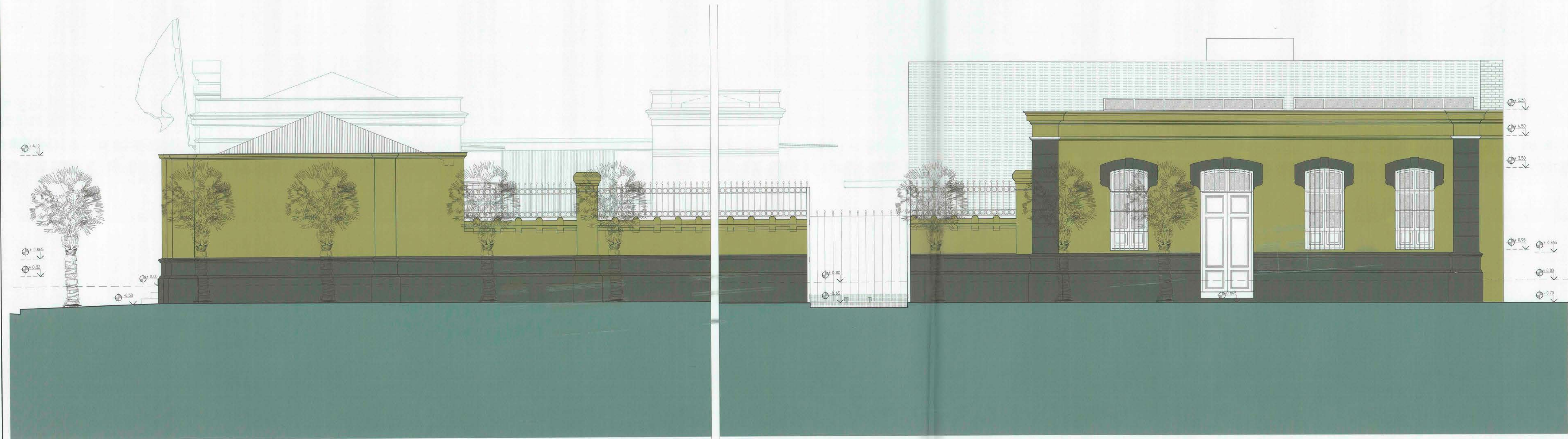
ELEVACION ORIENTE (O'HIGGINS) ESC. 1:50
