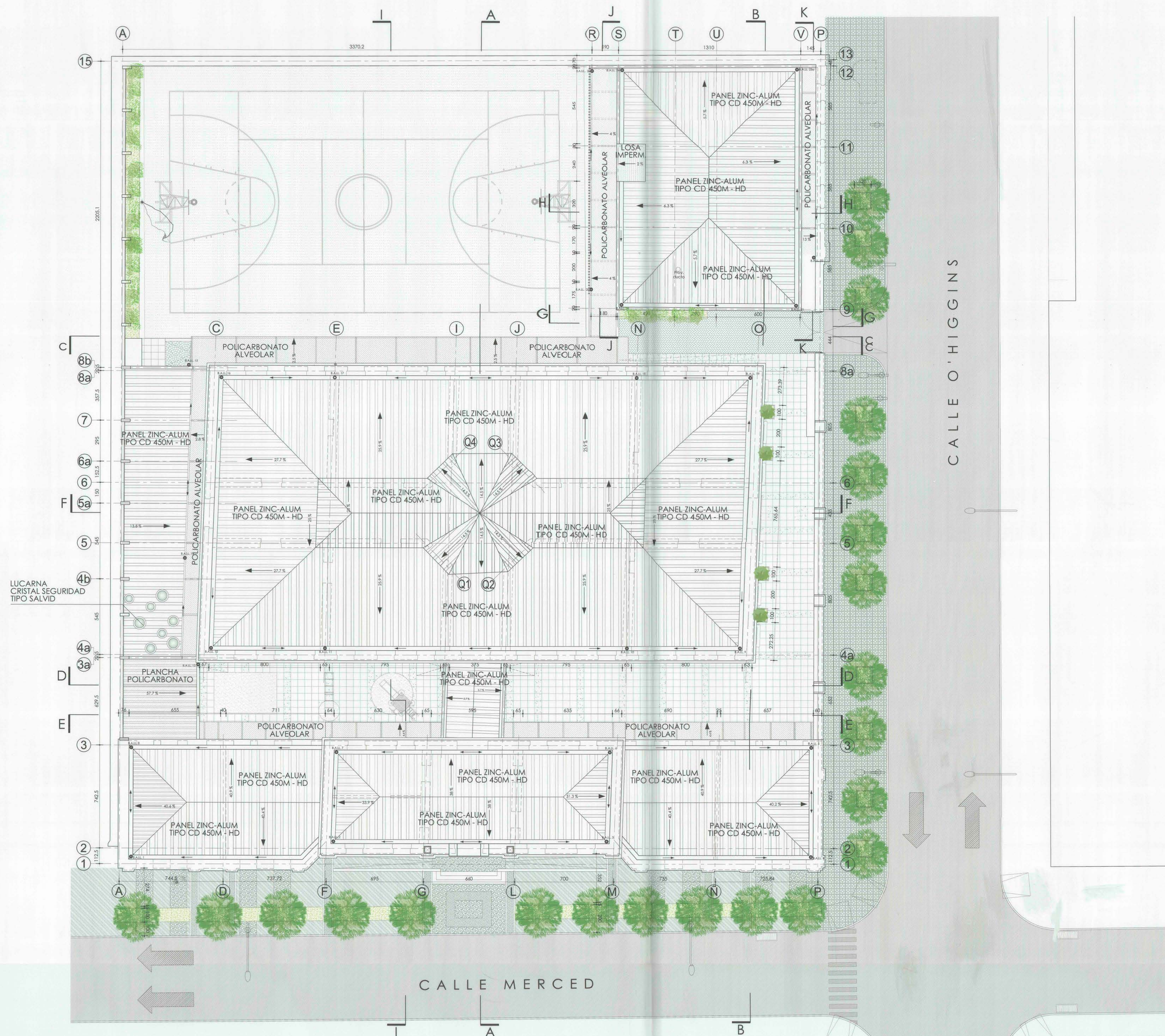
PLANTA GENERAL CUBIERTA
