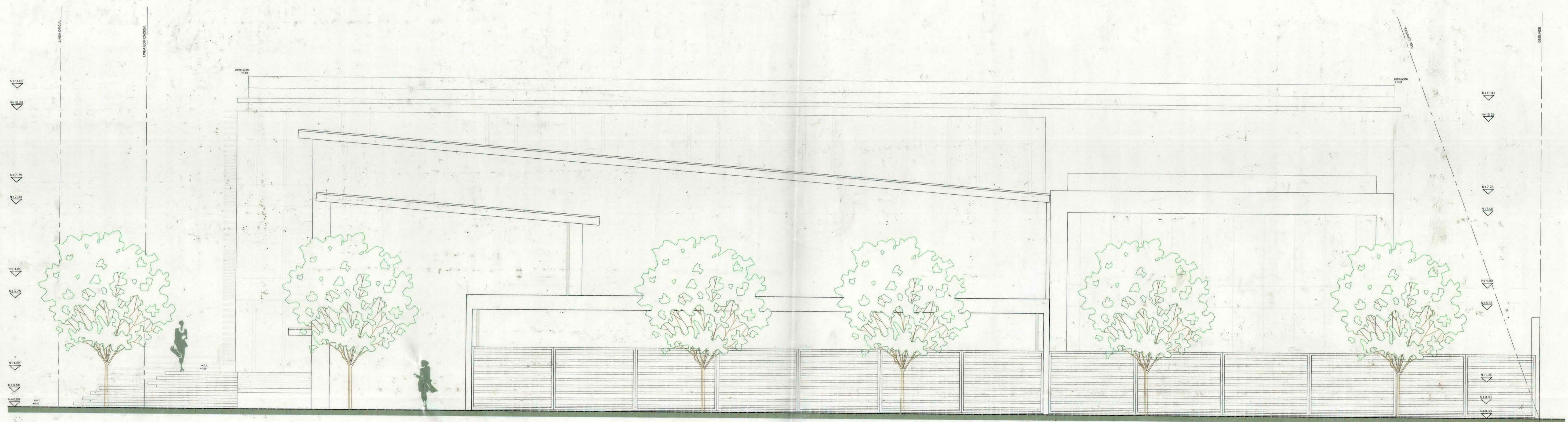
ELEVACIÓN SUR esc. 1:50
