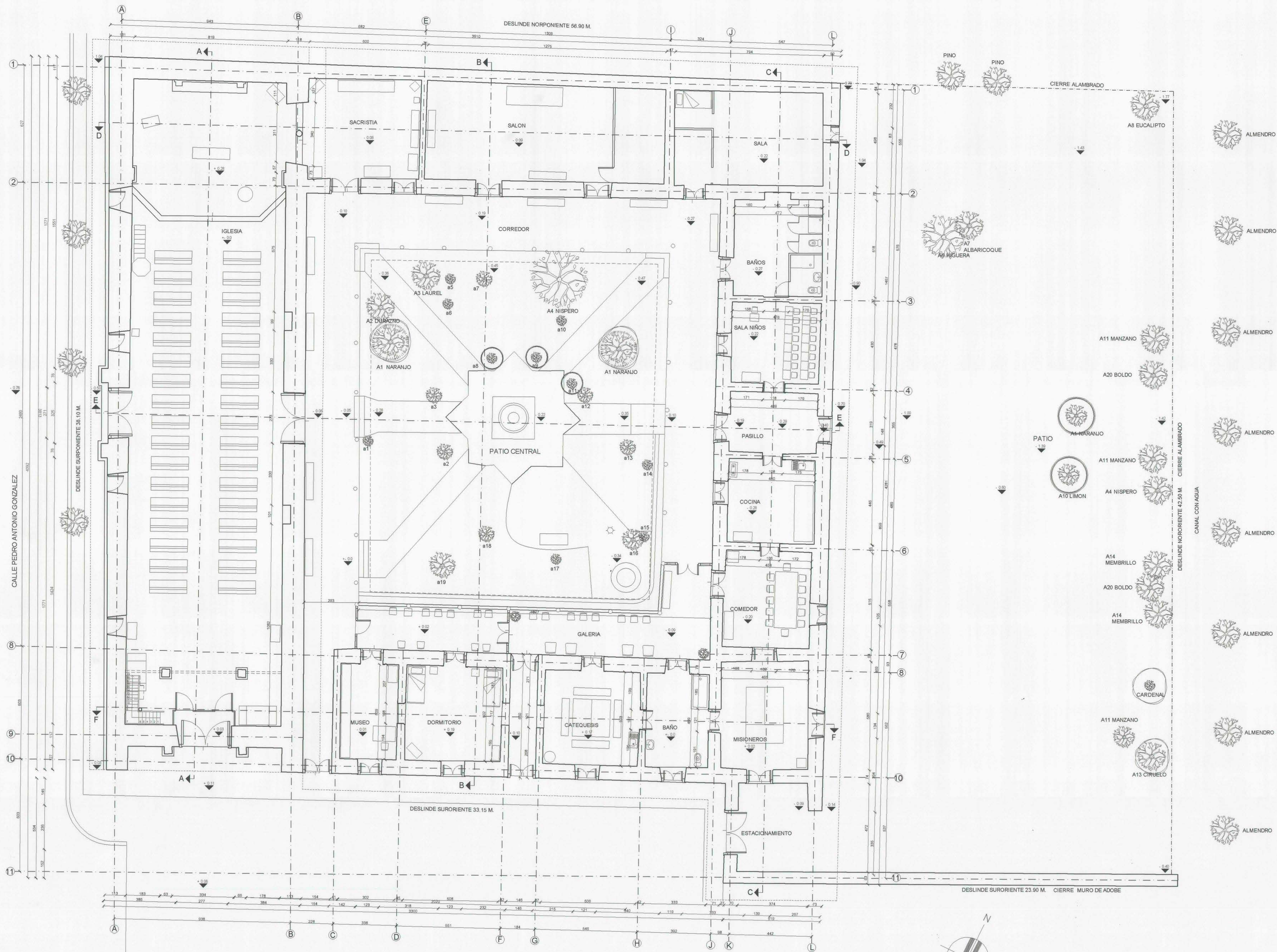
PLANTA PARROQUIA Y CASA PARROQUIAL ESCALA 1:75
