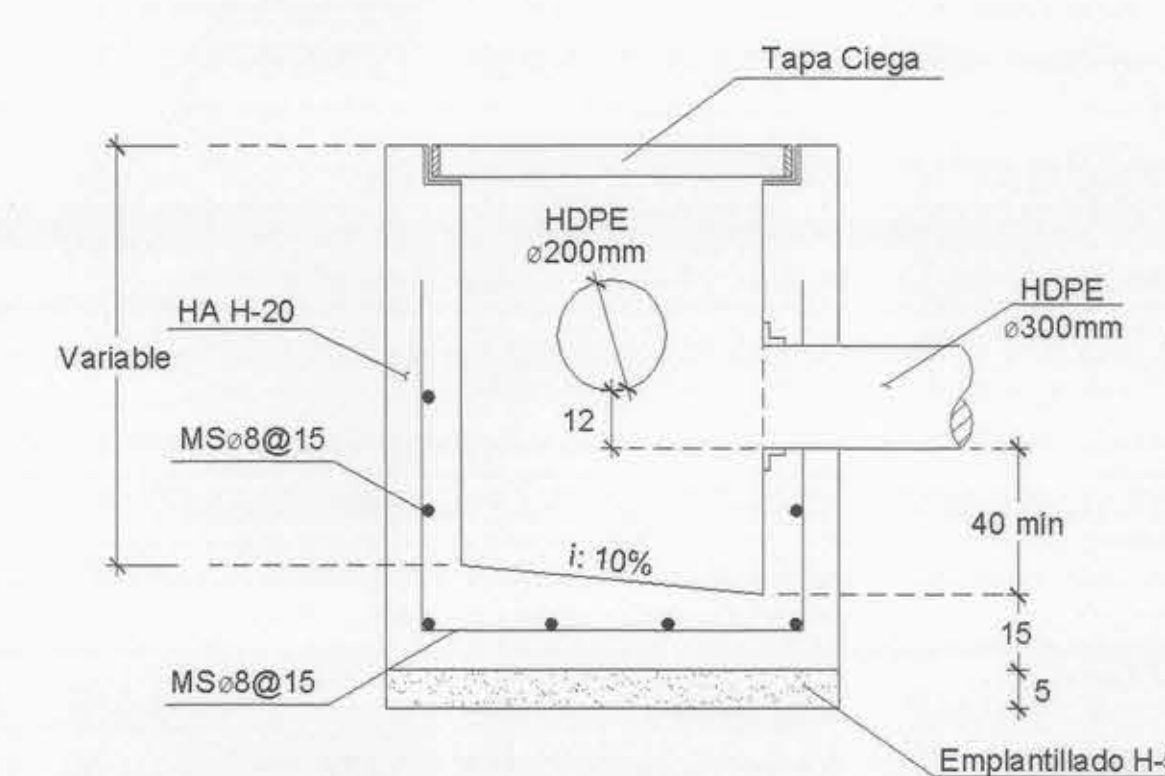
CORTE CÁMARA SEDIMENTACIÓN SIN ESCALA
