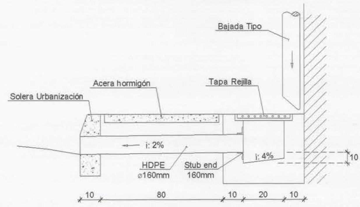
DETALLE BAJADA A CALZADA TIPO SIN ESCALA
