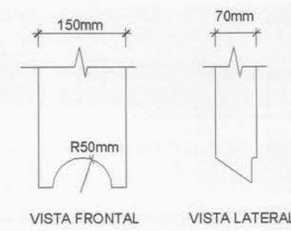
DETALLE BAJADA CORTA GOTA SIN ESCALA
