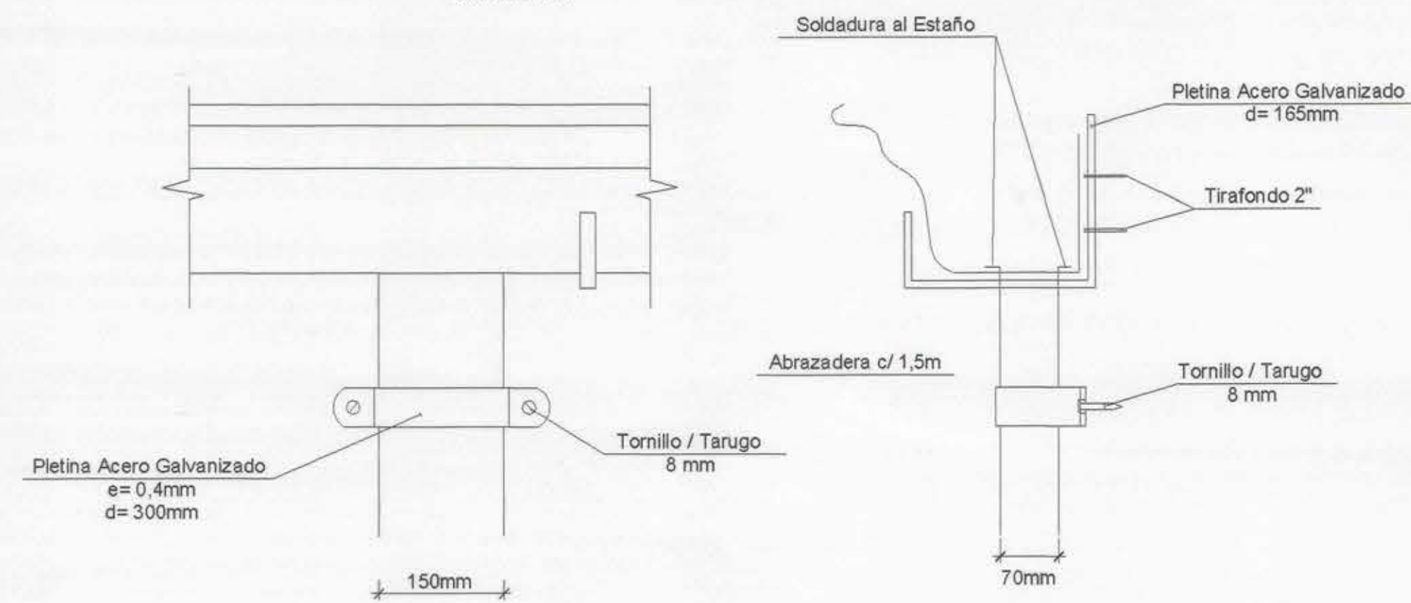
DETALLE UNION / ABRAZADERA SIN ESCALA
