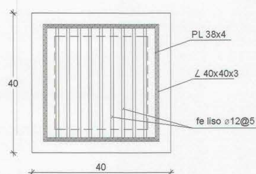
PLANTA CÁMARA TIPO SIN ESCALA
