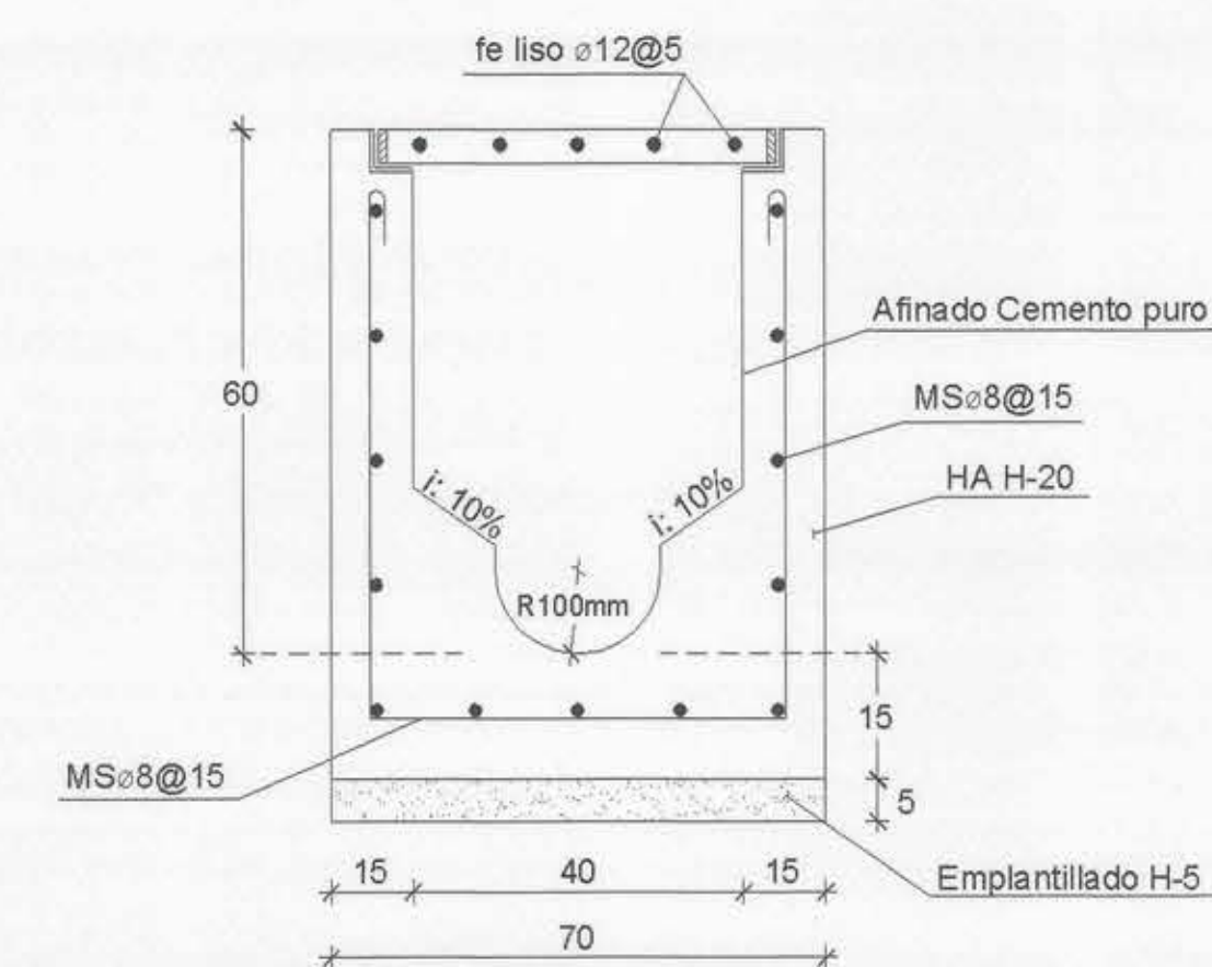
CORTE CÁMARA TIPO SIN ESCALA
