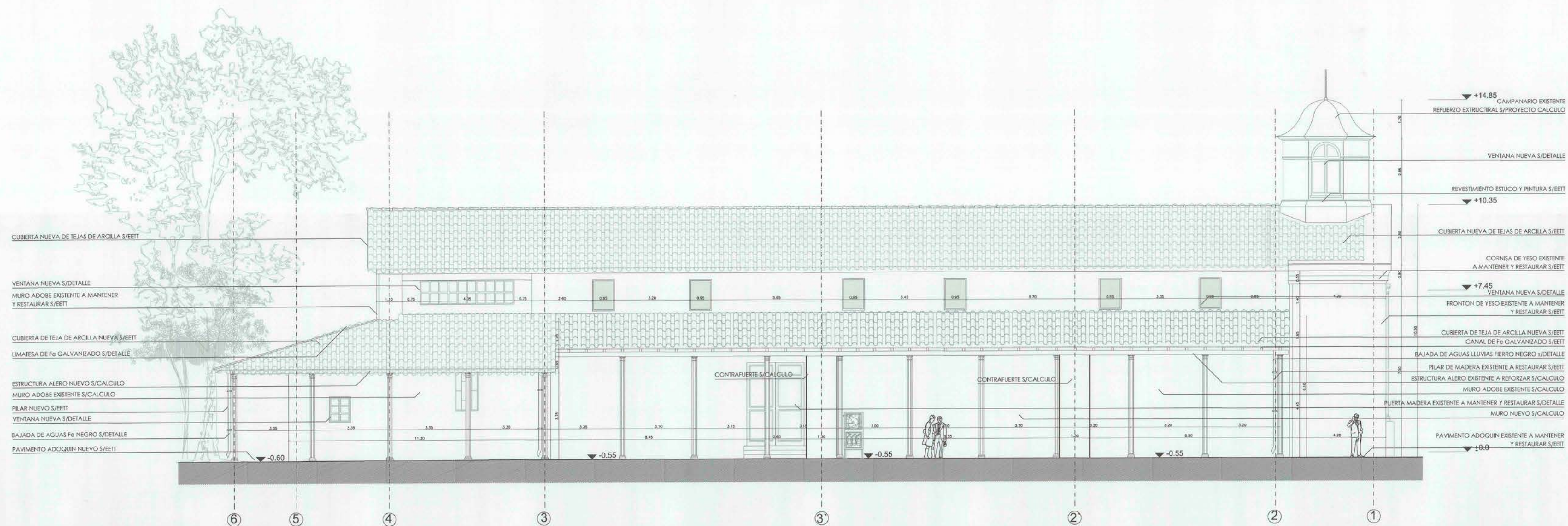
ELEVACIÓN SUR esc. 1:100
