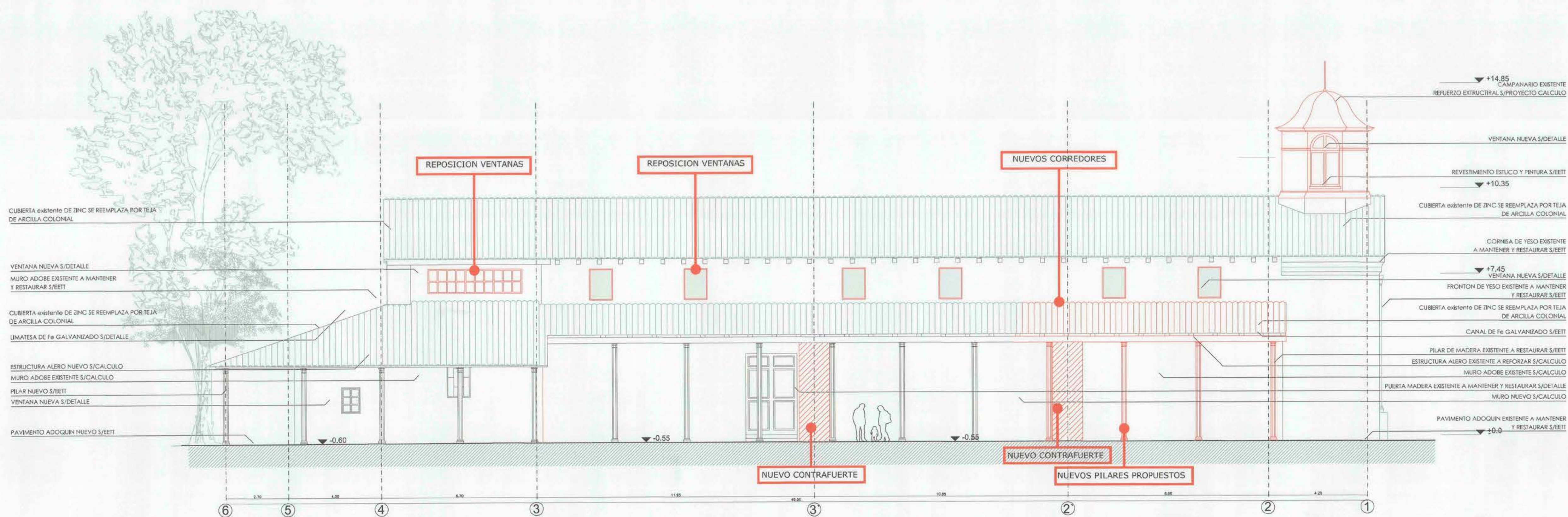
ELAVACIÓN SUR INTERVENCIONES esc. 1:100
