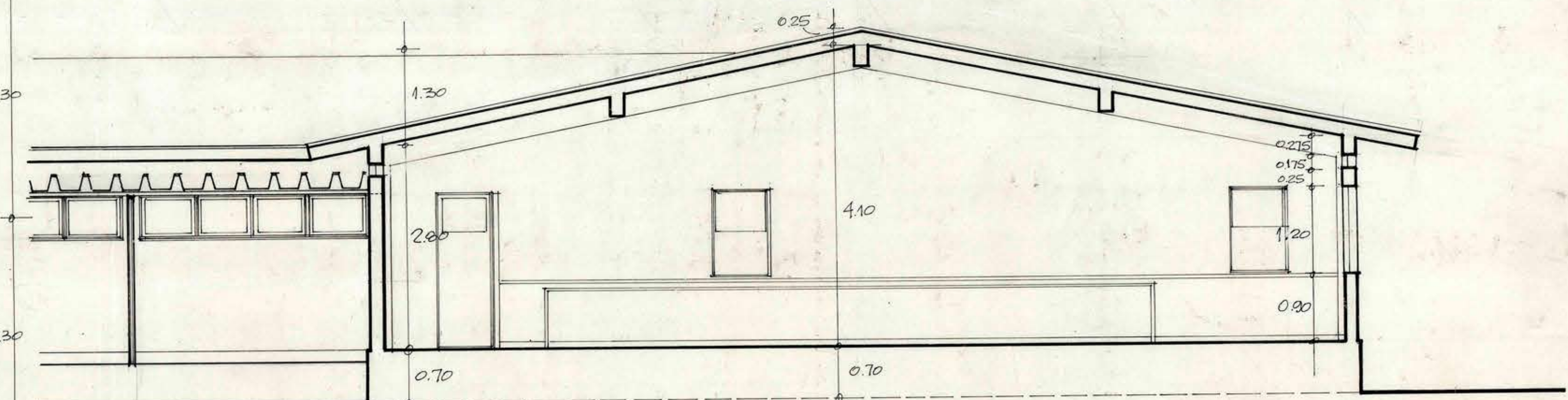
CORTE C - D
