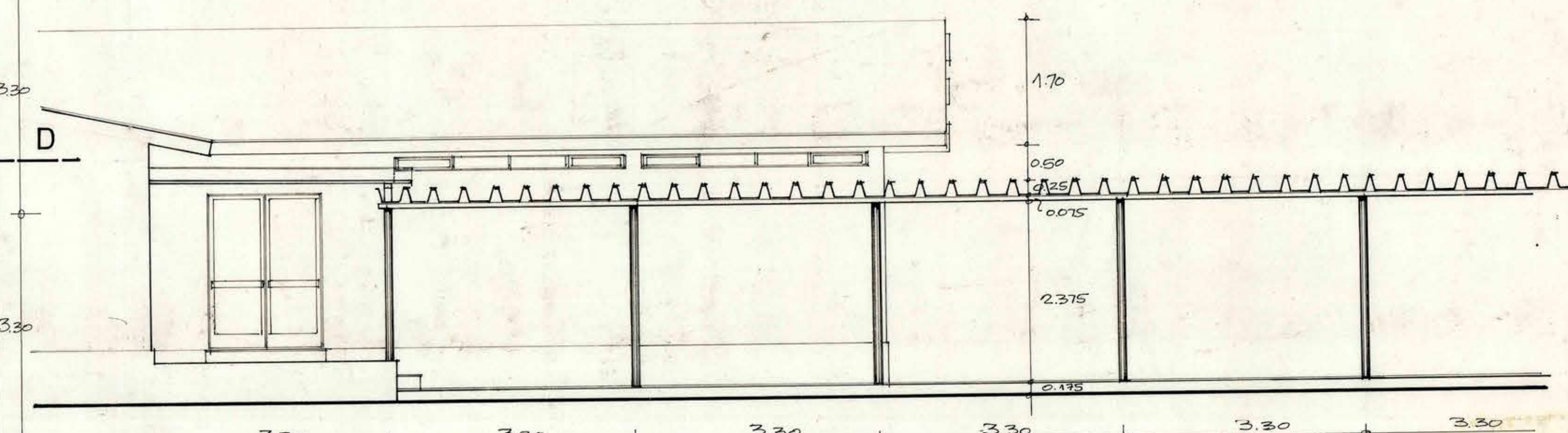
ELEVACION SUR parcial paso cubierto
