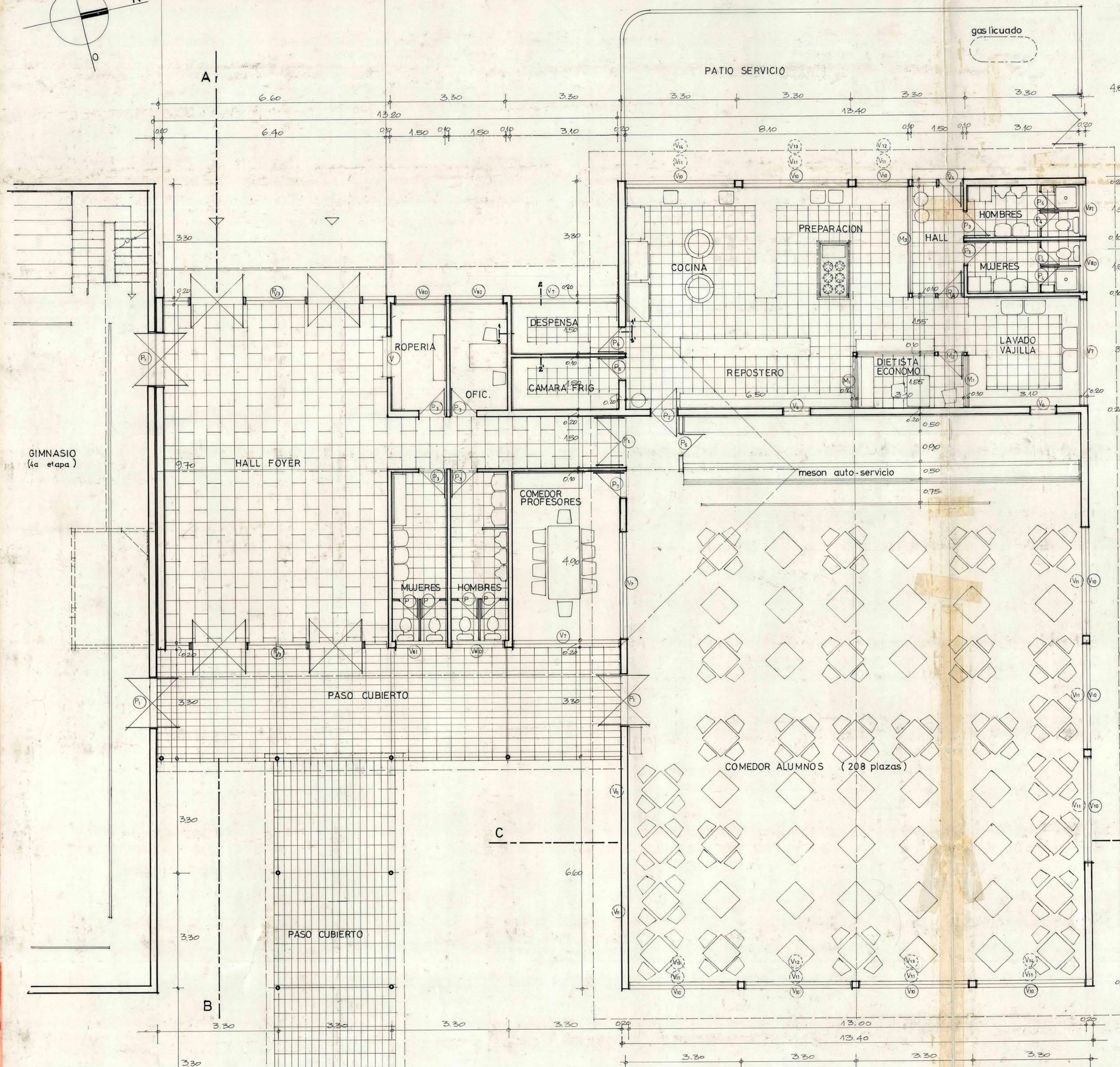
PLANTA ESC 1:50
