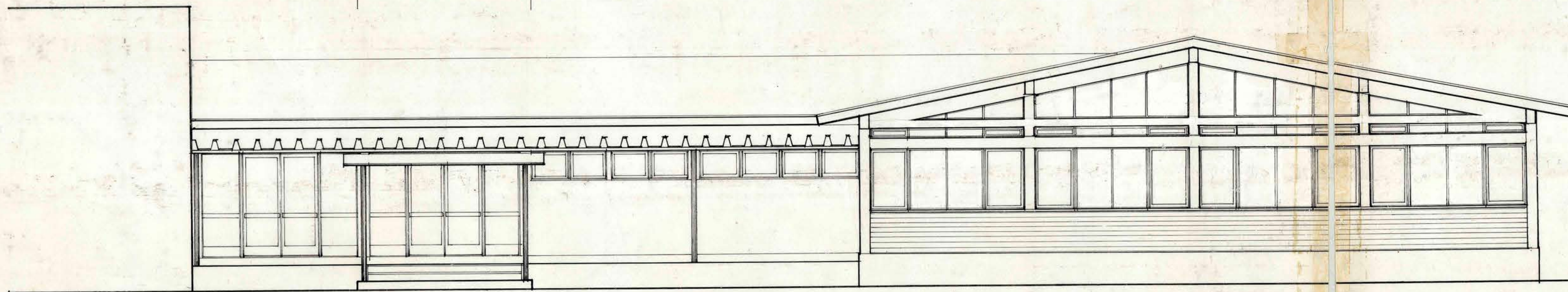
FACHADA ORIENTE
