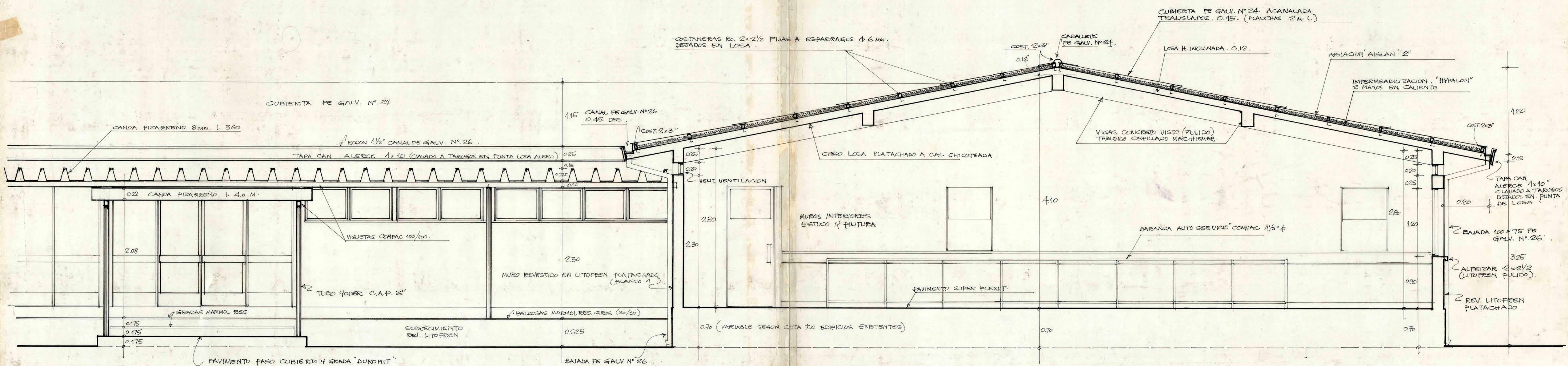
CORTE CONSTRUCCION C - D esc 1:25
