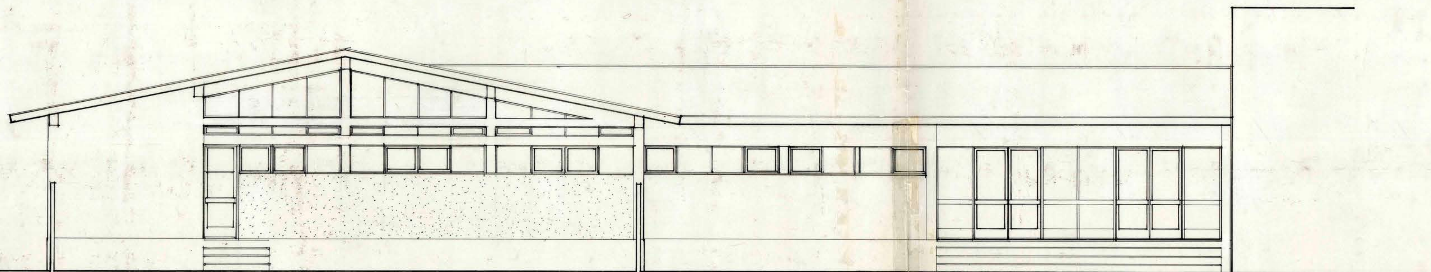
FACHADA PONIENTE
