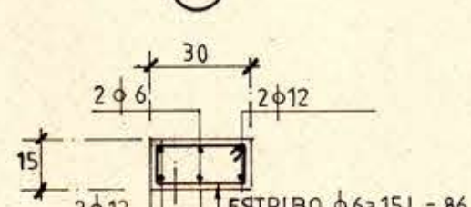
DETALLE PILARES Y MACHONES
