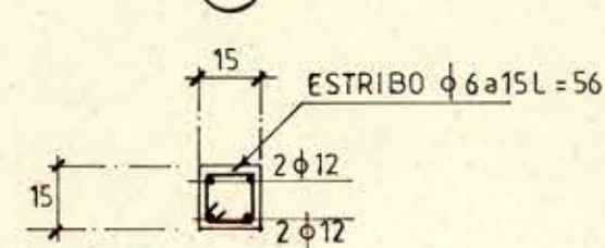
DETALLE PILARES Y MACHONES
