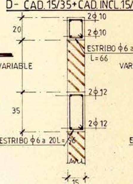
PLANTA ESCALA 1:50 DETALLES CADENAS, DINTES Y VIGAS ESCALA 1:20
