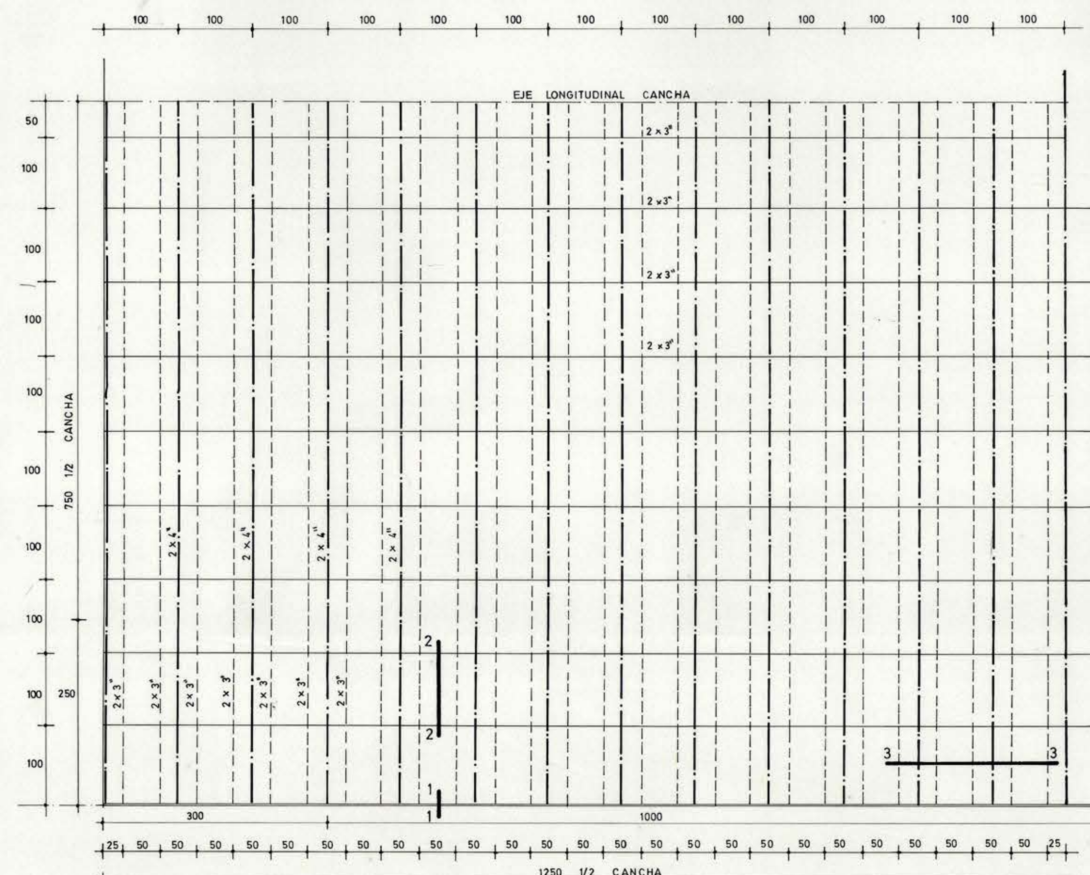
PLANTA ENTRAMADO PAVIMENTO CANCHA ESC 1:50
