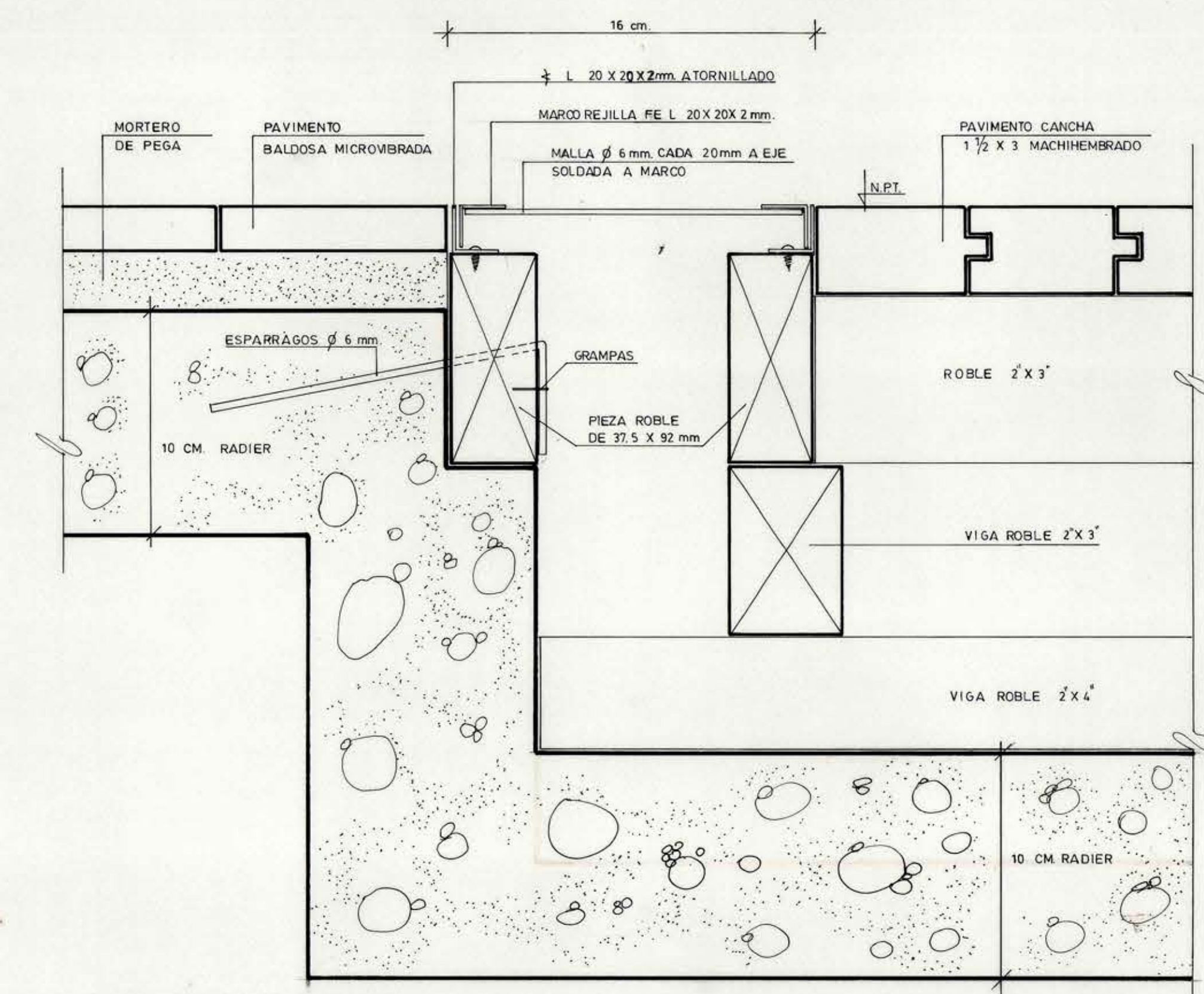
DETALLE ENCUESTRO PAVIMENTO CANCHA Y PAVIMENTO BALDOSA Y REJILLA DE VENTILACION PERIMETRAL DE CANCHA ESC 1:2
